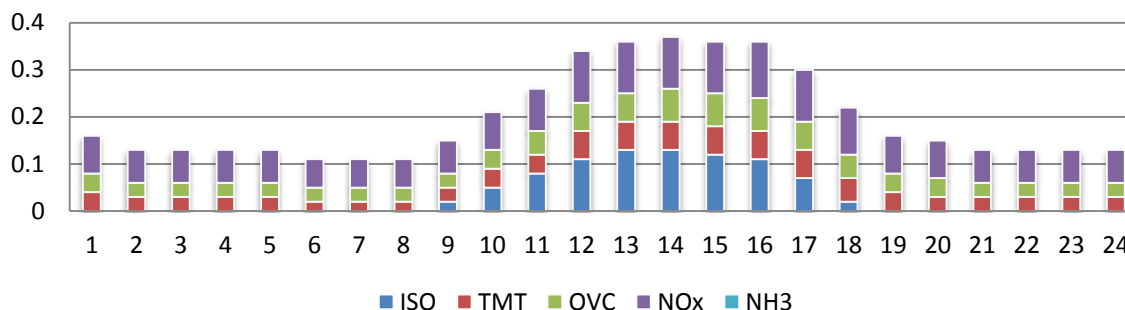
Figura 3.27 Emisiones horarias de fuentes biogénicas en el Estado de Tlaxcala.
