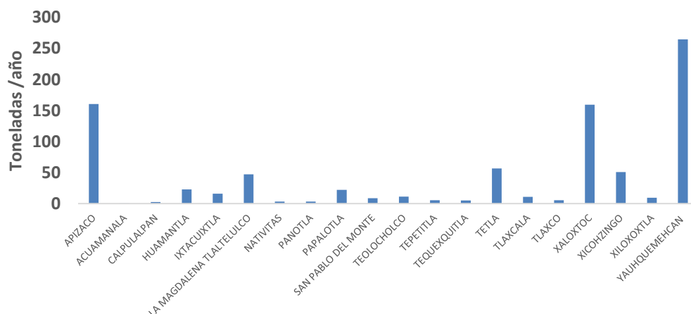
Figura 3.10 Emisiones de fuentes fijas desglosadas por municipio en toneladas al año.
