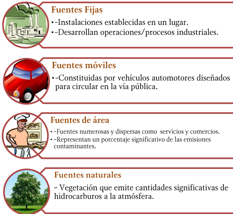
Figura 3.1 Fuentes del inventario de emisiones a la atmósfera.
