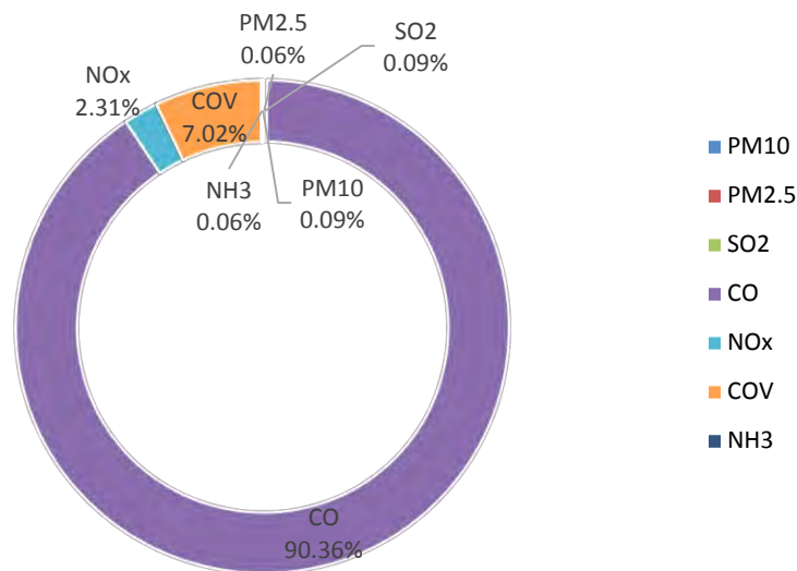
Figura 3.14 Distribución porcentual por contaminante en fuentes móviles del Estado de Tlaxcala.
