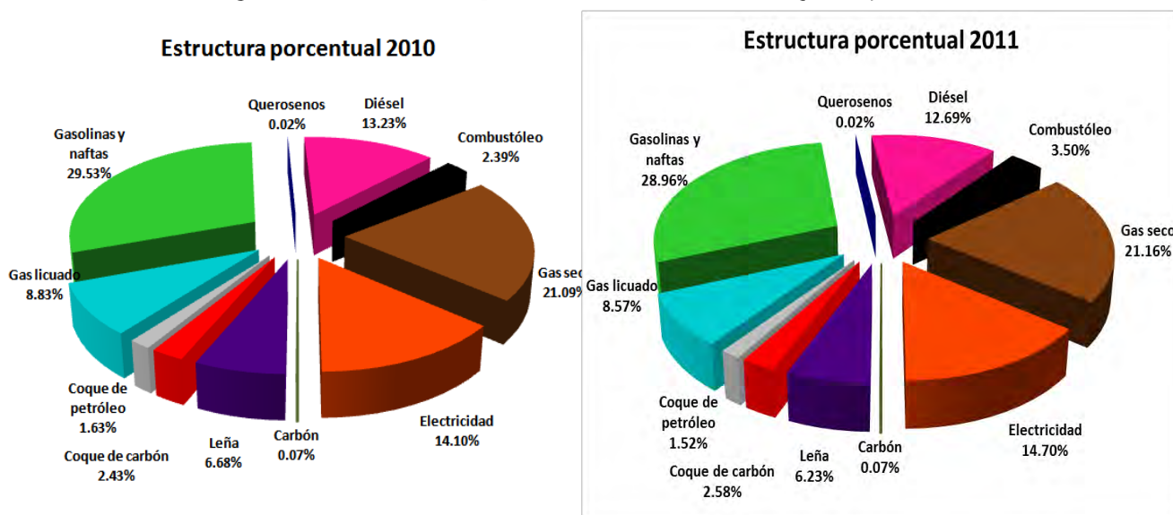
Figura 3.32 Estructura porcentual del consumo energético final total.
