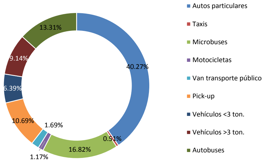
Figura 3.15 Distribución porcentual de partículas PM10 por categoría vehicular.
