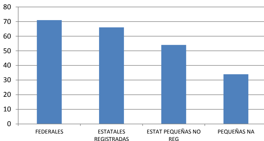
Figura 3.7 Número de industrias por competencia en el Estado de Tlaxcala.
