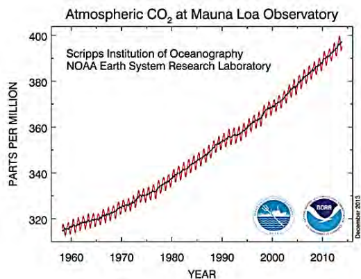
Figura 2.10 Promedios anuales de dióxido de carbono en el observatorio de Mauna Loa, Hawaii. Dr. Pieter Tans, NOAA/ESRL ( www.esrl.noaa.gov/gmd/ccgg/trends/ ) and Dr. Ralph Keeling, Scripps.
