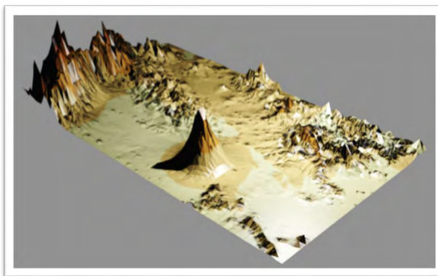
Figura 4.5 Digitalización de elevación del Estado de Tlaxcala.
