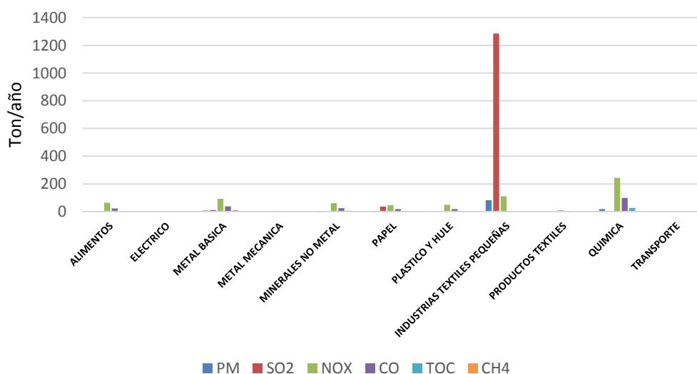
Figura 3.11 Generación de contaminantes por giro industrial en el Estado de Tlaxcala.
