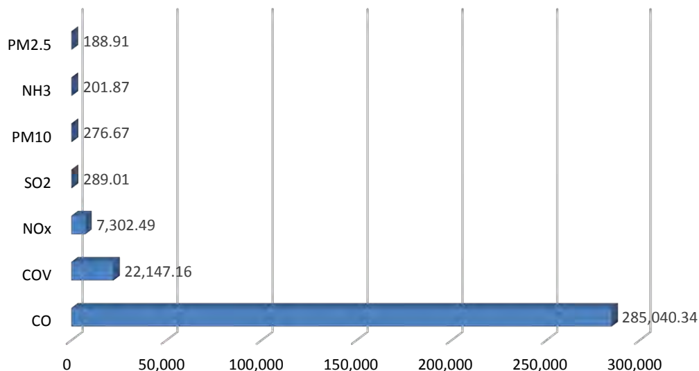
Figura 3.13 Resultados de los contaminantes en fuentes móviles (ton/año).
