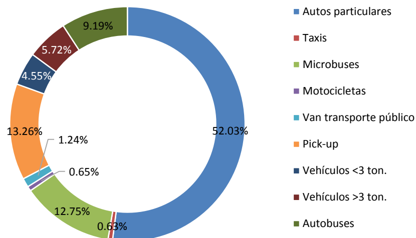
Figura 3.17 Distribución porcentual de contaminante SO_2 por categoría vehicular.
