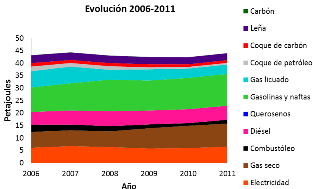
Figura 3.33 Evolución anual del consumo final total de energía.
