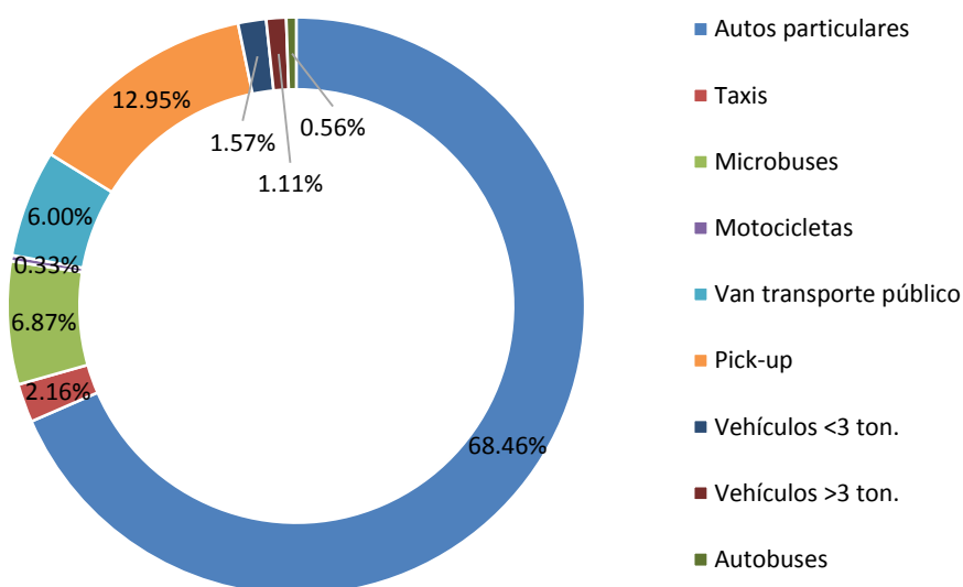
Figura 3.21 Distribución porcentual de contaminante \text{NH}_3 por categoría vehicular.
