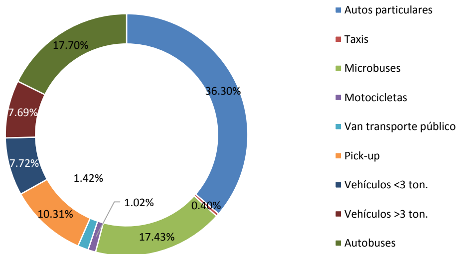
Figura 3.16 Distribución porcentual de partículas PM2.5 por categoría vehicular.
