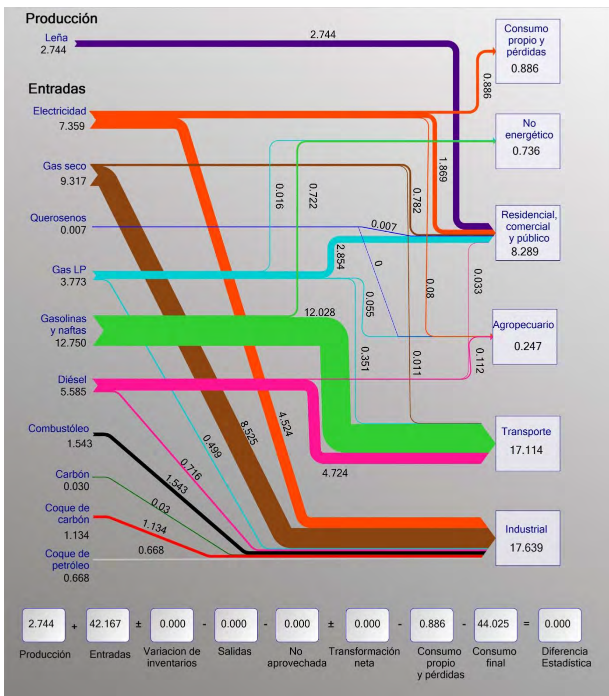
Figura 3.30 Balance energético estatal 2011, en petajoules (PJ).
