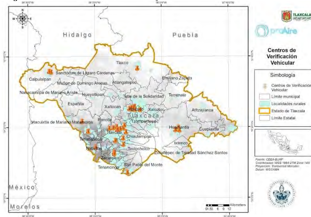
Figura 2.7 Ubicación de centros de verificación vehicular del Estado de Tlaxcala.
