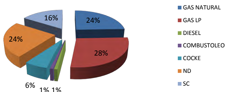
Figura 3.8 Consumo de combustibles por las fuentes fijas en el Estado de Tlaxcala.
