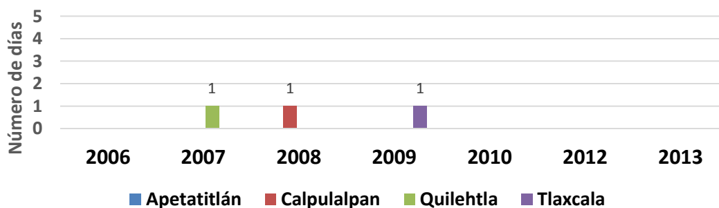
Figura 2.3 Días por arriba del valor límite permisible por estación de monitoreo de PM 10 .
