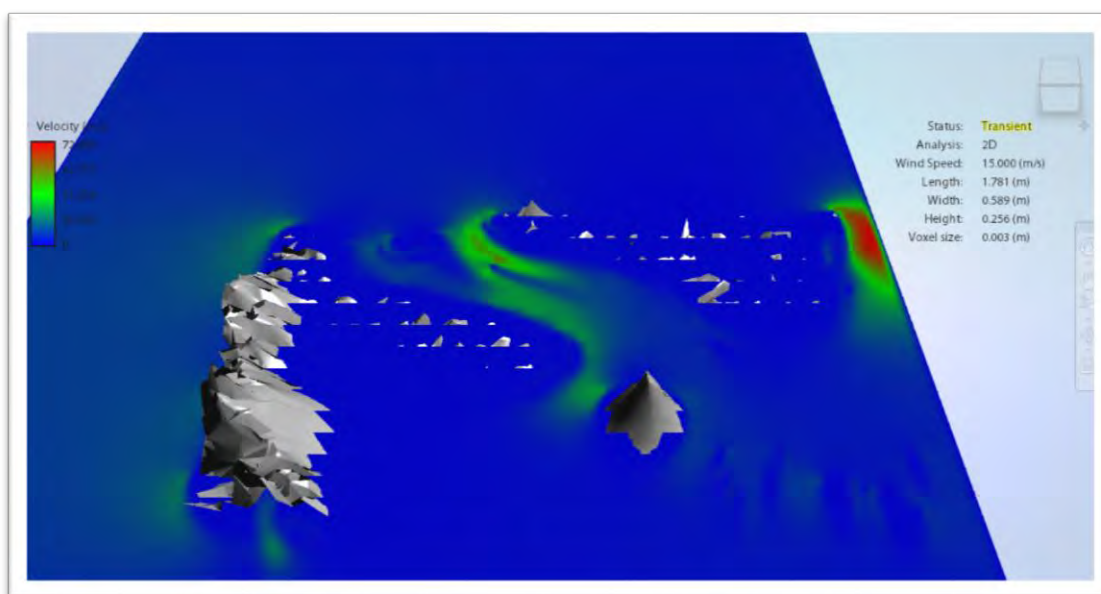
Figura 4.7 Canales de viento.
