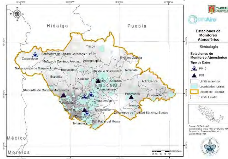
Figura 2.1 Ubicación de estaciones de la red de monitoreo atmosférico del Estado de Tlaxcala.
