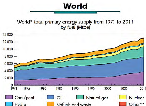
Figura 2.11 Producción mundial de energía 1971-2011.
