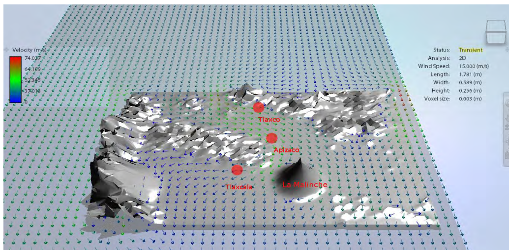
Figura 4.8 Vectorización de los canales de viento.
