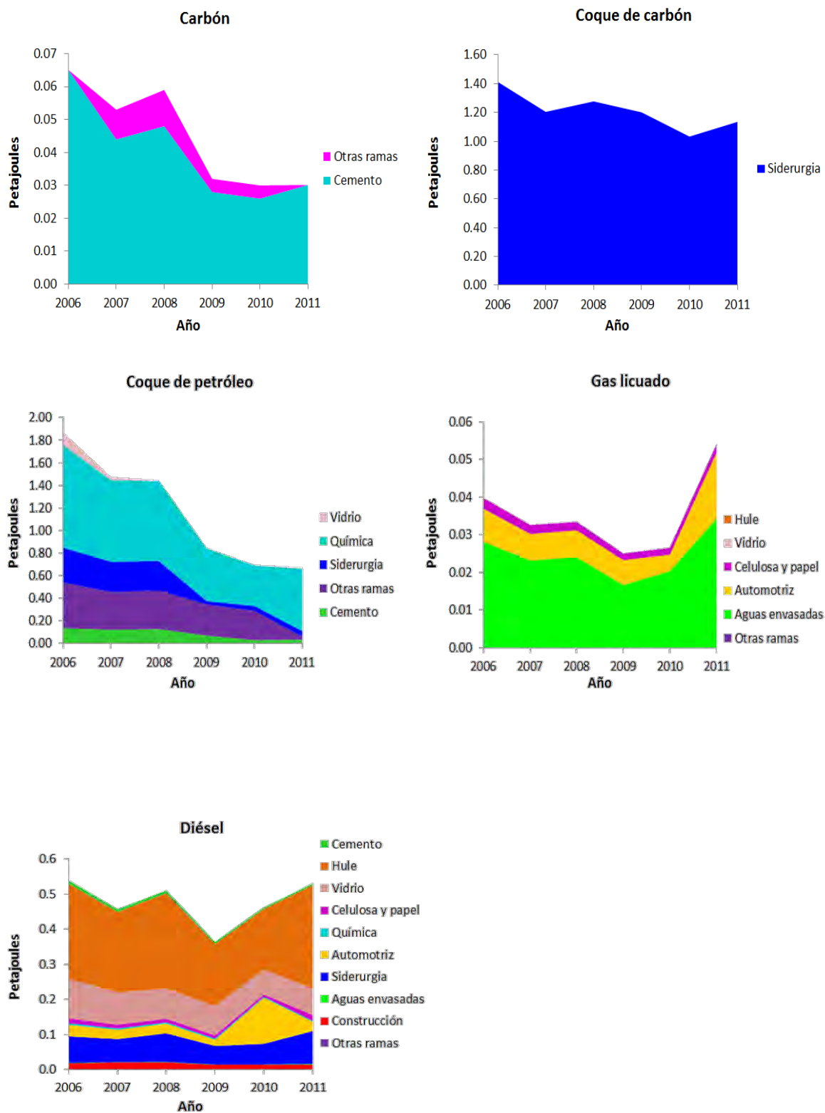
Figura 3.34 Evolución anual del consumo energético por rama industrial.
