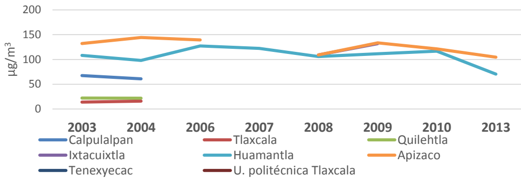
Figura 2.4 Concentración promedio anual por estación de monitoreo de PST ( \mu\text{g}/\text{m}^3 ).
