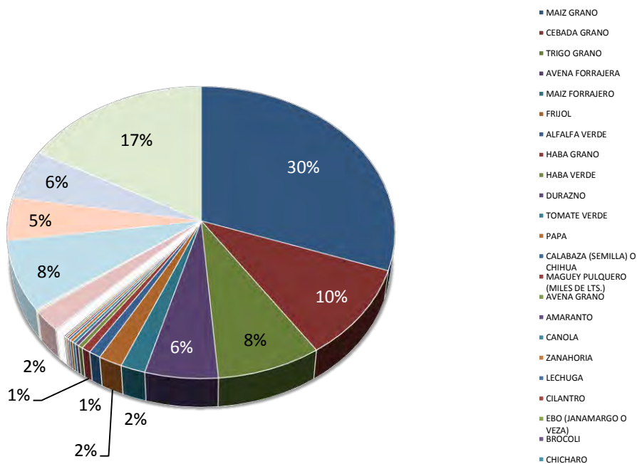
Figura 3.26 Uso de suelo general Estado de Tlaxcala (hectáreas), total de Ha sembradas 248,776.75.
