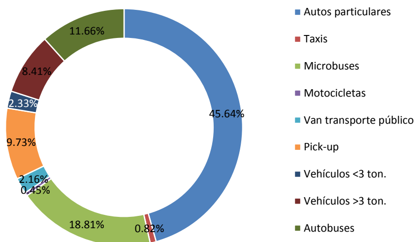
Figura 3.19 Distribución porcentual de contaminante NOx por categoría vehicular.
