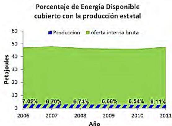
Figura 3.31 Porcentaje de la energía disponible cubierto con producción estatal. La franja azul constituyen la producción, el fondo verde representa el total de energía disponible.
