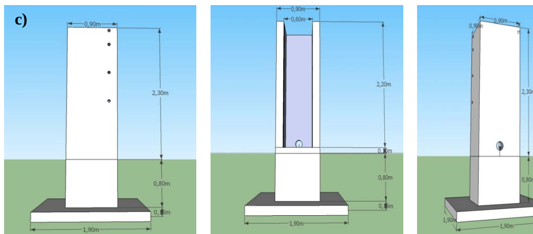
Figura. Sistema excluidor de fauna acuática de prototipo Bolso conectado a registro con tubo excluidor (SEFA-2): a) vista general, b) dispositivo de filtrado y c) especificaciones del colector de organismos.
