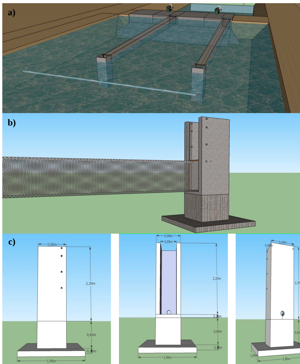
Figura. Sistema excluidor de fauna acuática de prototipo Bolso conectado a registro con tubo excluidor (SEFA-2): a) vista general, b) dispositivo de filtrado y c) especificaciones del colector de organismos.
