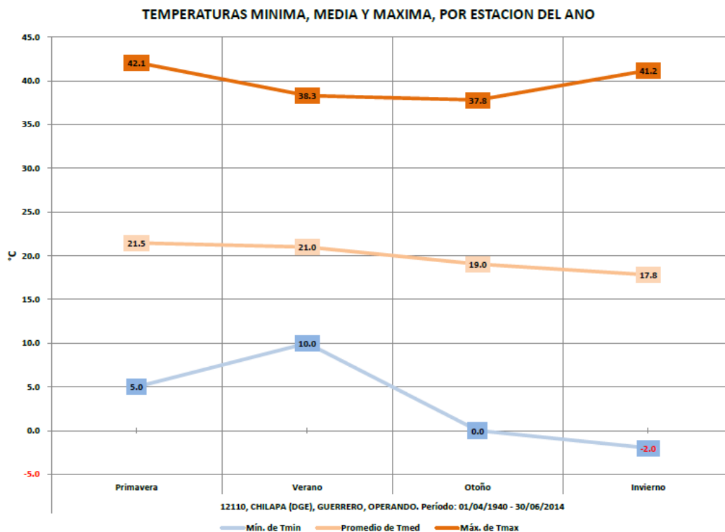
Gráfico 1. Temperaturas de la estación Chilapa (DGE) TEMPERATURAS MÍNIMA, MEDIA Y MÁXIMA, POR ESTACIÓN DEL AÑO
