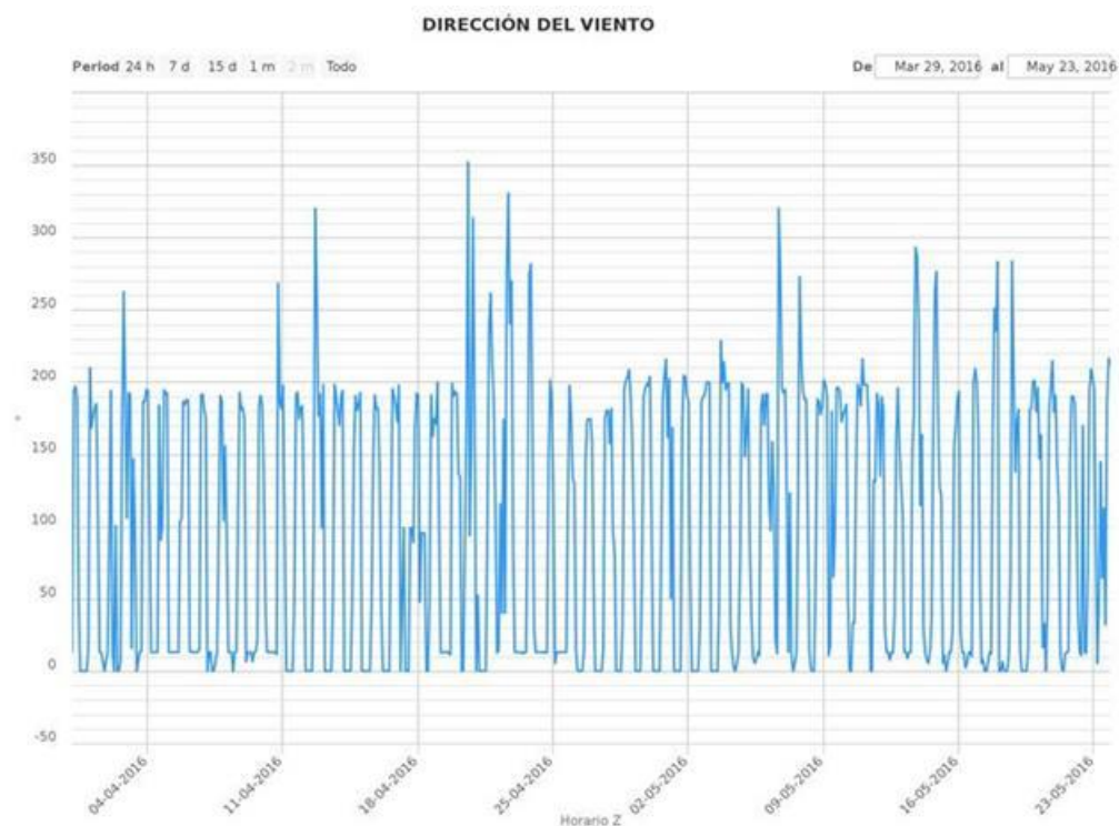
Gráfico 8. Dirección del viento en la estación meteorológica de Chilapa.
