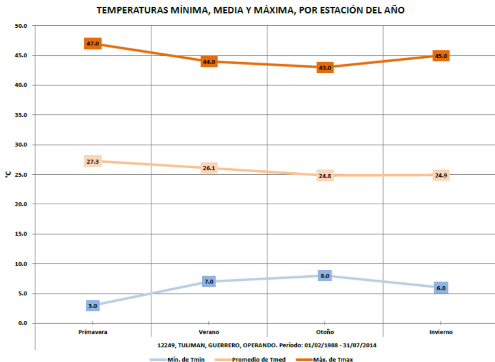
Gráfico 5. Temperaturas de la estación Tuliman
