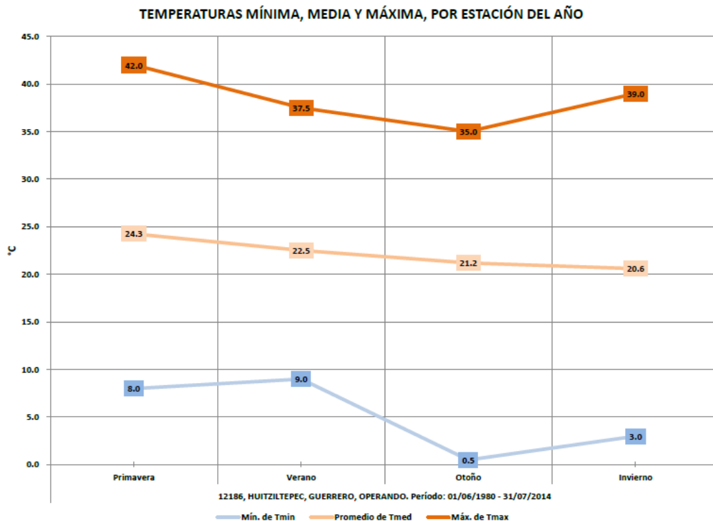
Gráfico 3. Temperaturas de la estación Huitziltepec. TEMPERATURAS MÍNIMA, MEDIA Y MÁXIMA, POR ESTACIÓN DEL AÑO
