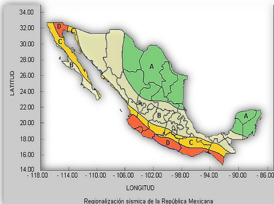
Figura 47. Regionalización sísmica de la República Mexicana.
