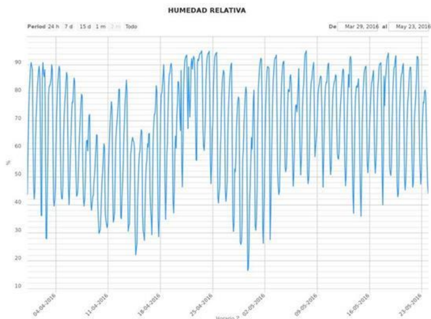
Gráfico 6. Humedad relativa en la estación meteorológica automática de Chilapa.
