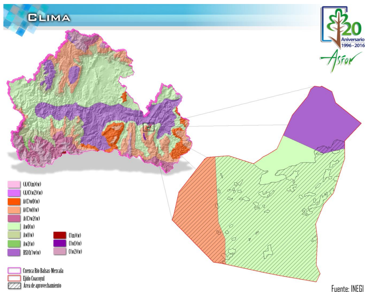
Figura 39. Tipos de climas de la Cuenca y predio del proyecto (INEGI)
