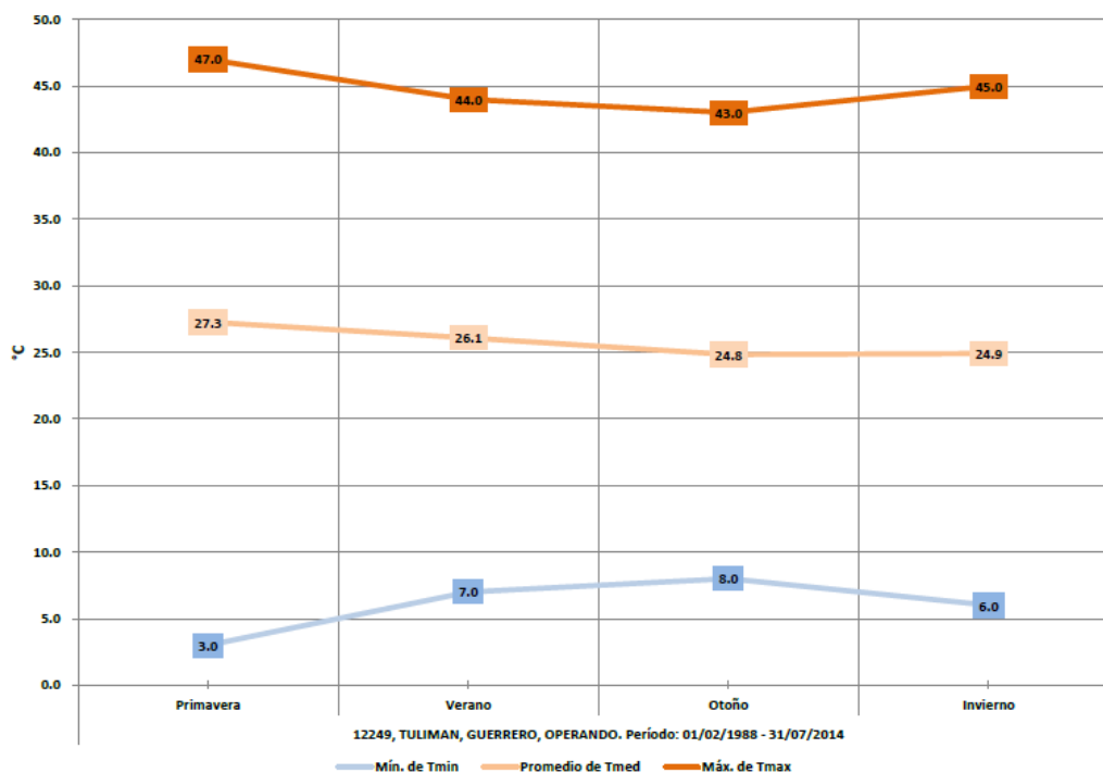
Gráfico 5. Temperaturas de la estación Tuliman
