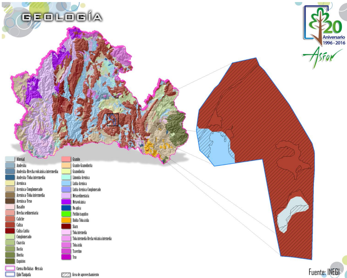
Figura 41. Geología en la cuenca y sitio del proyecto.
