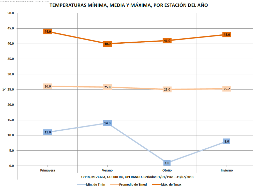
Gráfico 2. Temperaturas de la estación Mezcala.
