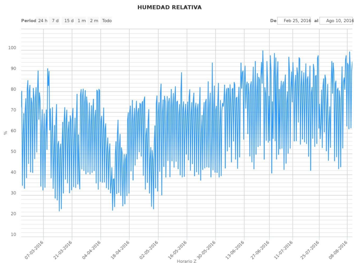
Gráfico 6. Humedad relativa en la estación meteorológica automática de Chilpancingo.
