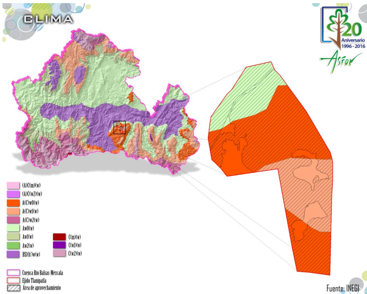
Figura 37. Tipos de climas de la Cuenca y predio del proyecto (INEGI)
