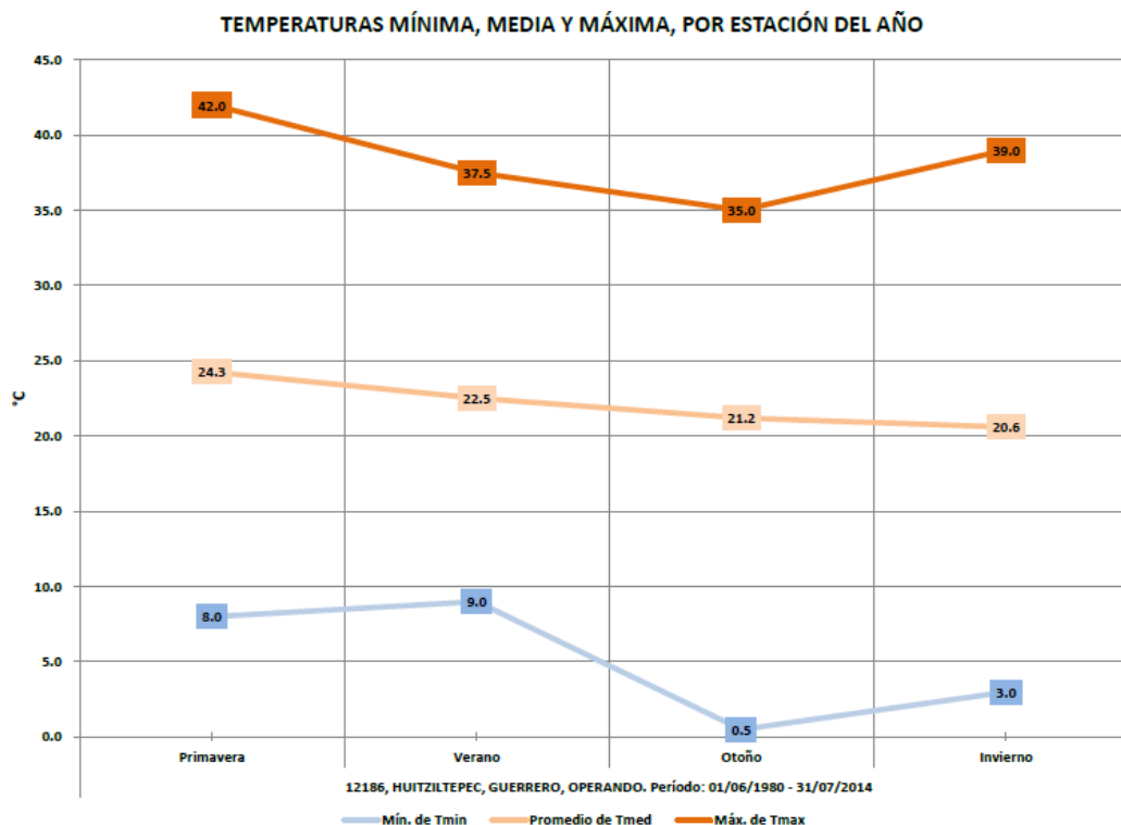
Gráfico 4. Temperaturas de la estación Huitziltepec. TEMPERATURAS MÍNIMA, MEDIA Y MÁXIMA, POR ESTACIÓN DEL AÑO
