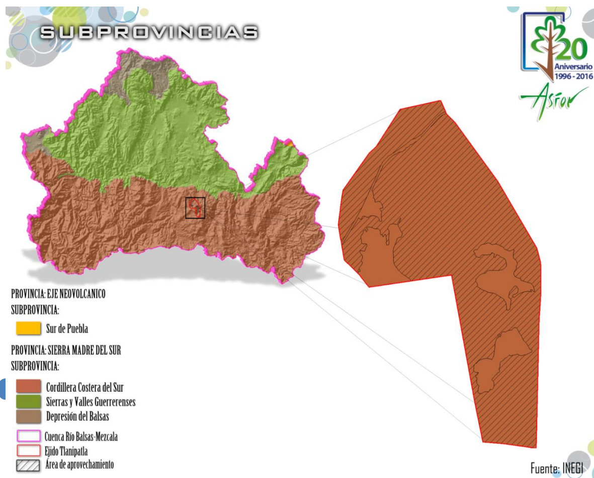
Figura 42. Fisiografía de la cuenca y sitio del predio.
