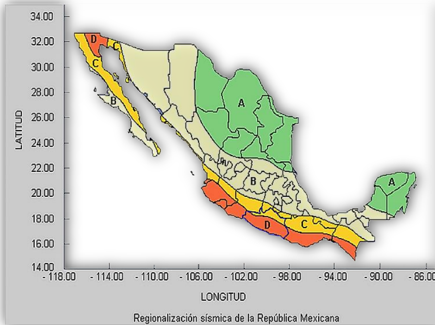
Figura 45. Regionalización sísmica de la República Mexicana.
