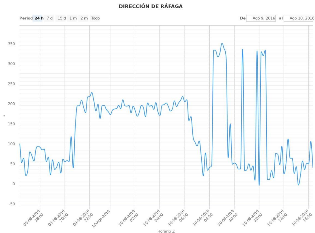
Gráfico 7. Dirección del viento de ráfaga en la estación meteorológica automática de Chilapa.
