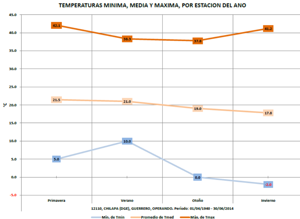
Gráfico 1. Temperaturas de la estación Chilapa (DGE)
