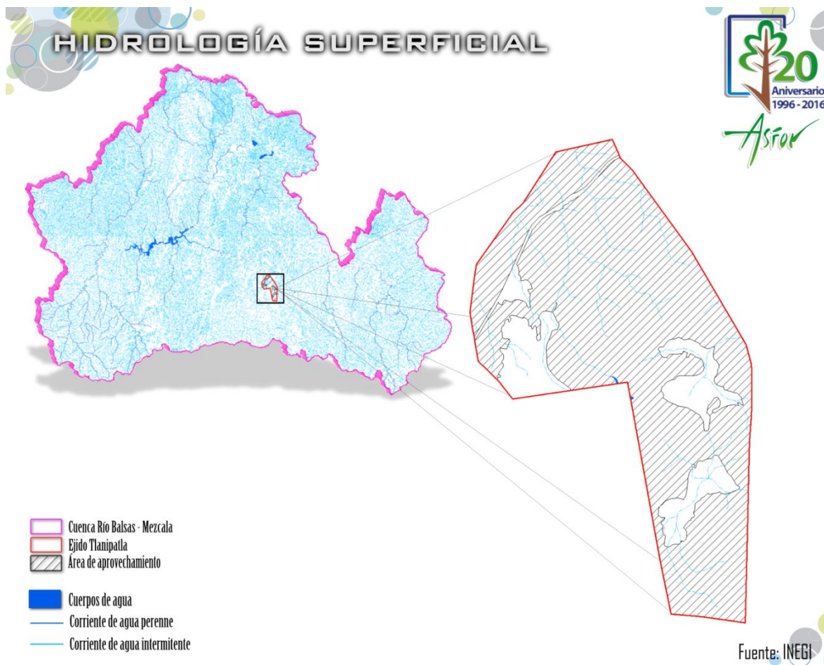
Figura 46. Hidrología superficial de la cuenca.
