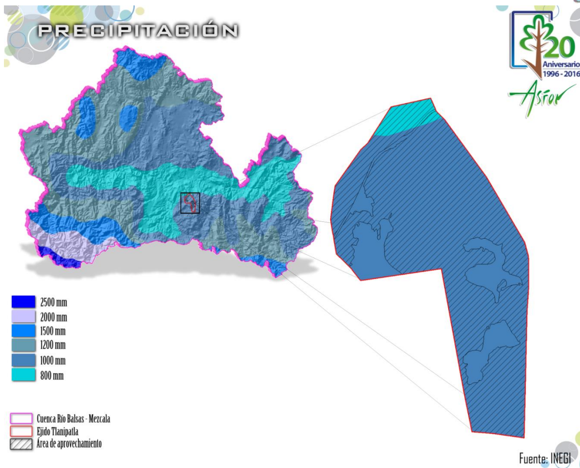
Figura 40. Precipitación registrada en el área del proyecto.
