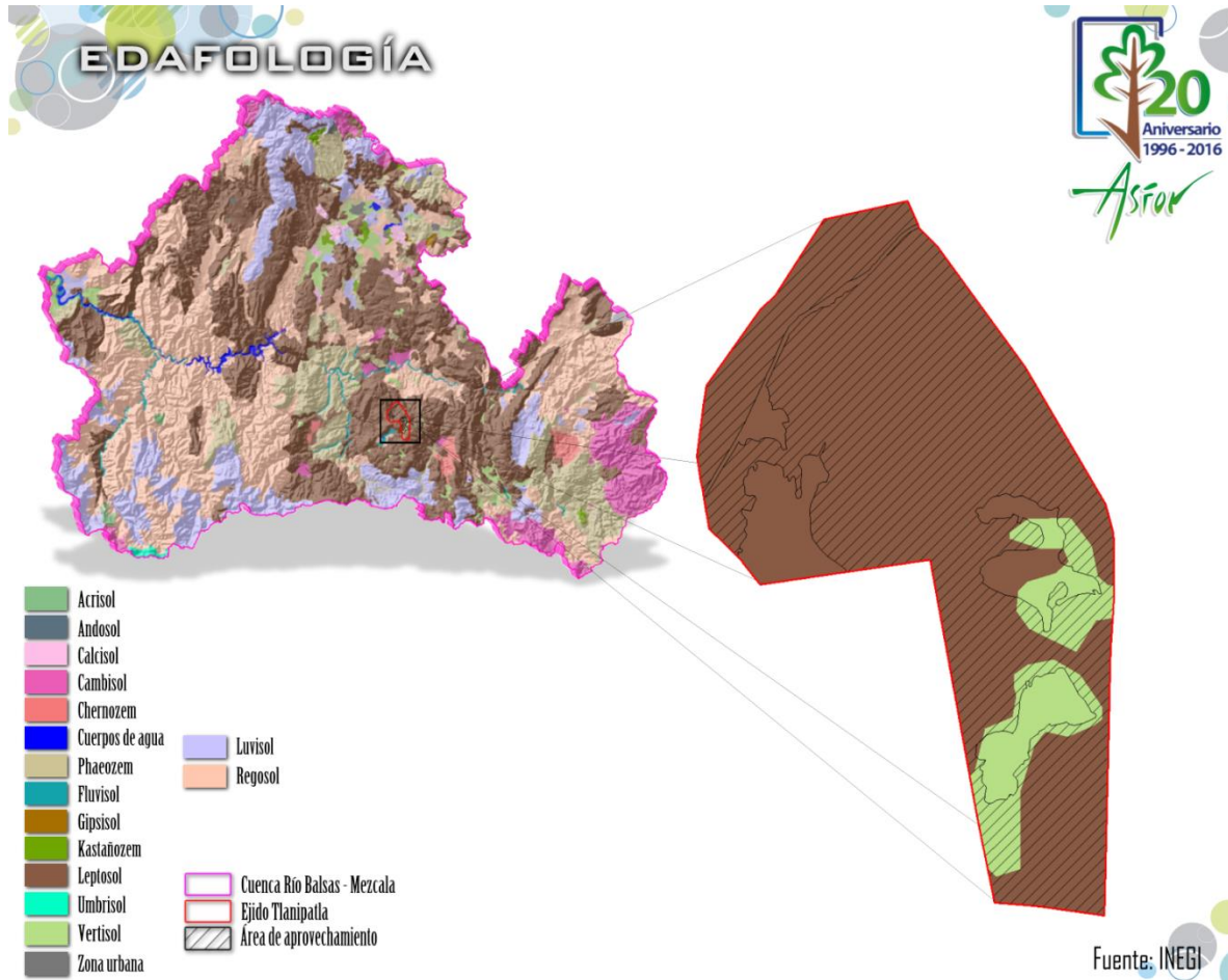
Figura 44. Tipo de suelo edafológico presente en el área del proyecto.
