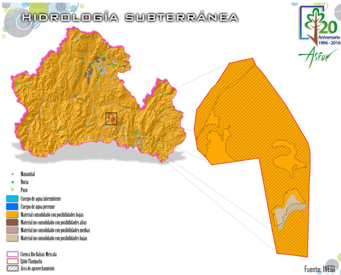
Figura 47. Hidrología subterránea de la cuenca.
