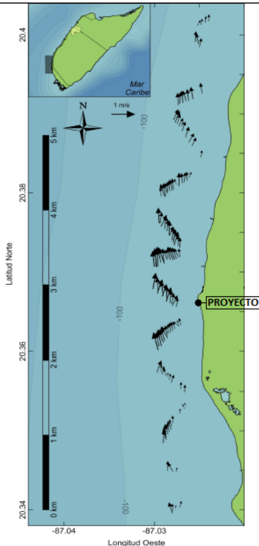
Figura 40. Vectores de velocidad obtenidos con el perfilador acústico de corrientes durante los recorridos de marzo de 2011. área suroeste del PNAC.
