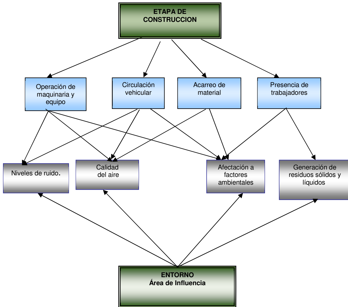
Figura 40. Diagrama de la interrelación causa-efecto, de las acciones durante la etapa de construcción del sitio modificado de Gómez Orea (2003).
