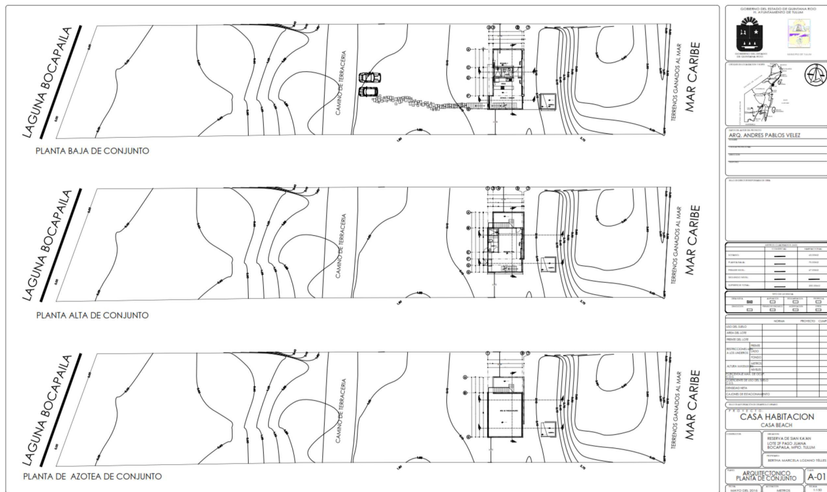
Figura 5. Plano de conjunto de proyecto.
