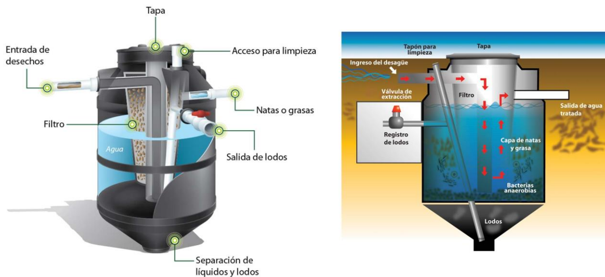
Ilustración 42.- Detalle Biodigestor
