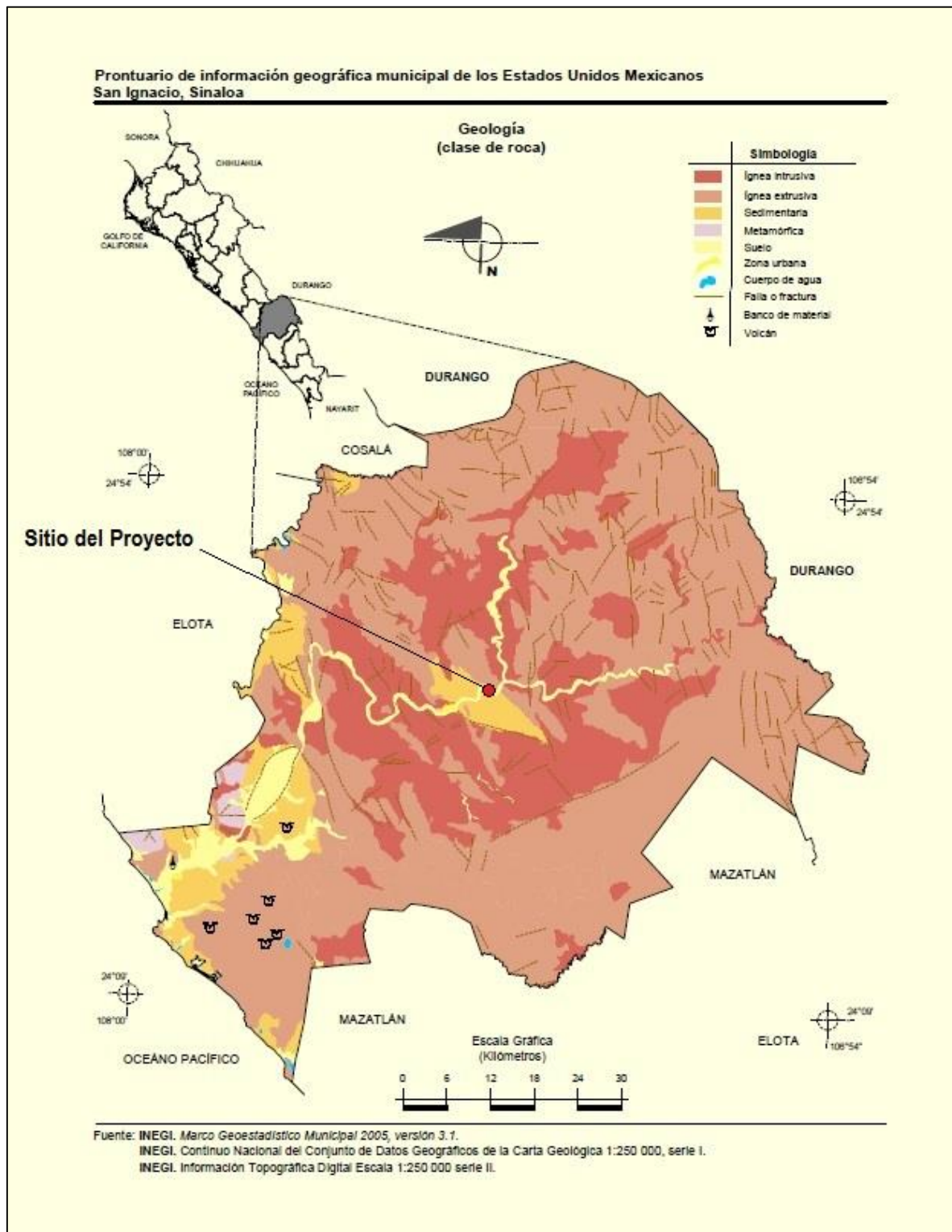
Imagen IV.7. Geología del Municipio de San Ignacio. INEGI.
