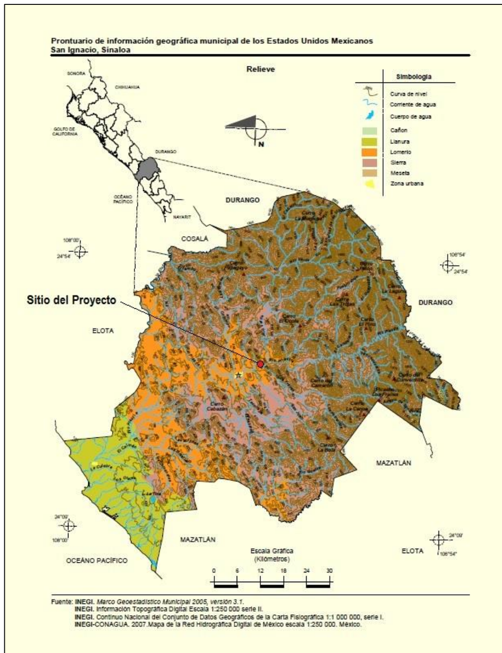
Imagen IV.9. Relieve del Municipio de San Ignacio. INEGI.
