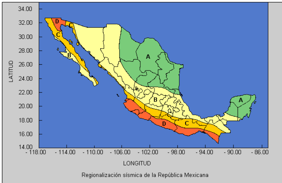
Imagen VI.18. Regionalización Sísmica de México.
