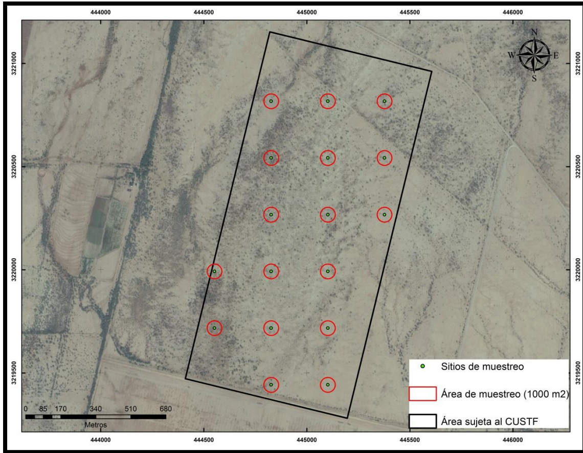
Figura 11. Distribución espacial de los sitios de muestreo en el área sujeta a la primera etapa del proyecto.
