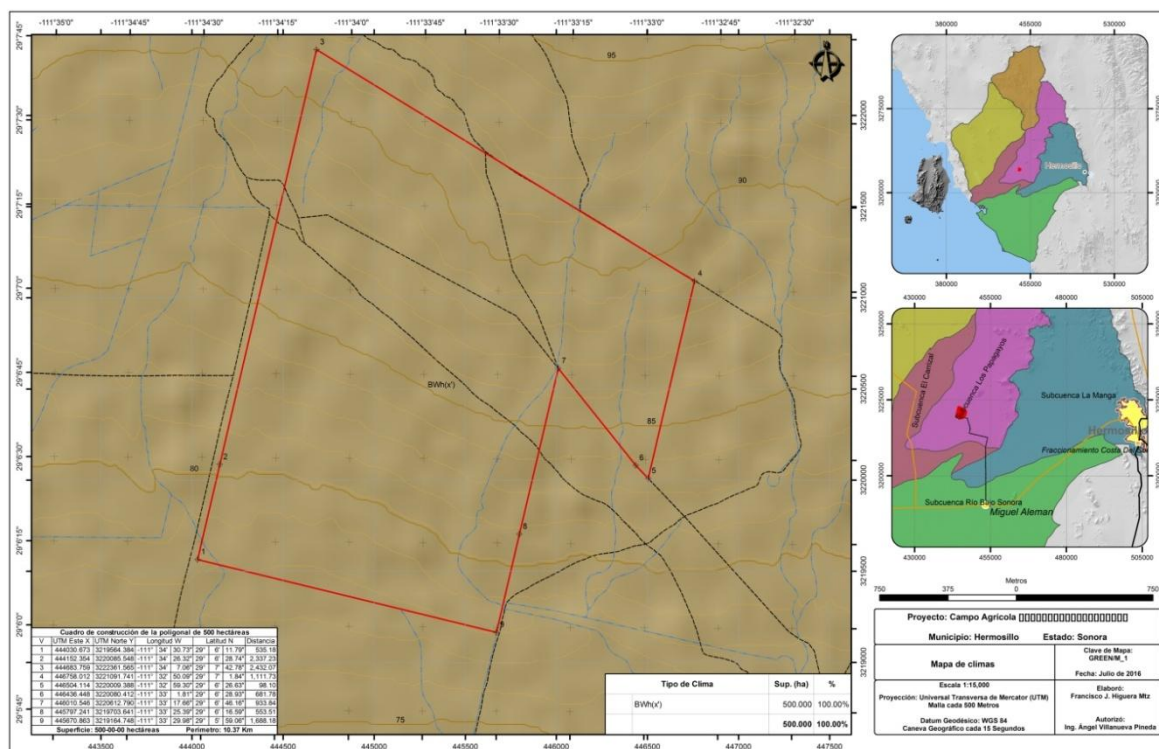
Figura 14. Tipo de clima dentro del área del proyecto "Ampliación Campo Agrícola Santa Eduwiges"
