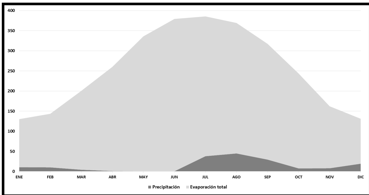
Figura 4. Precipitación y evaporación potencial en el área del proyecto
