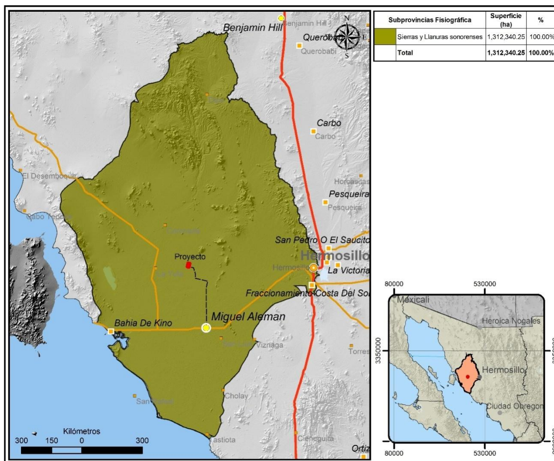
Figura 20. Subprovincias Fisiográficas en el Municipios de Hermosillo
