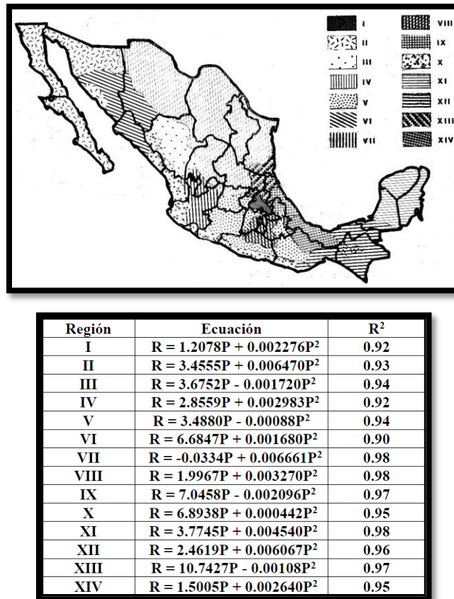
Figura 5. Mapa y ecuaciones para estimar la Erosividad de la Lluvia (R) en las diferentes regiones del país
