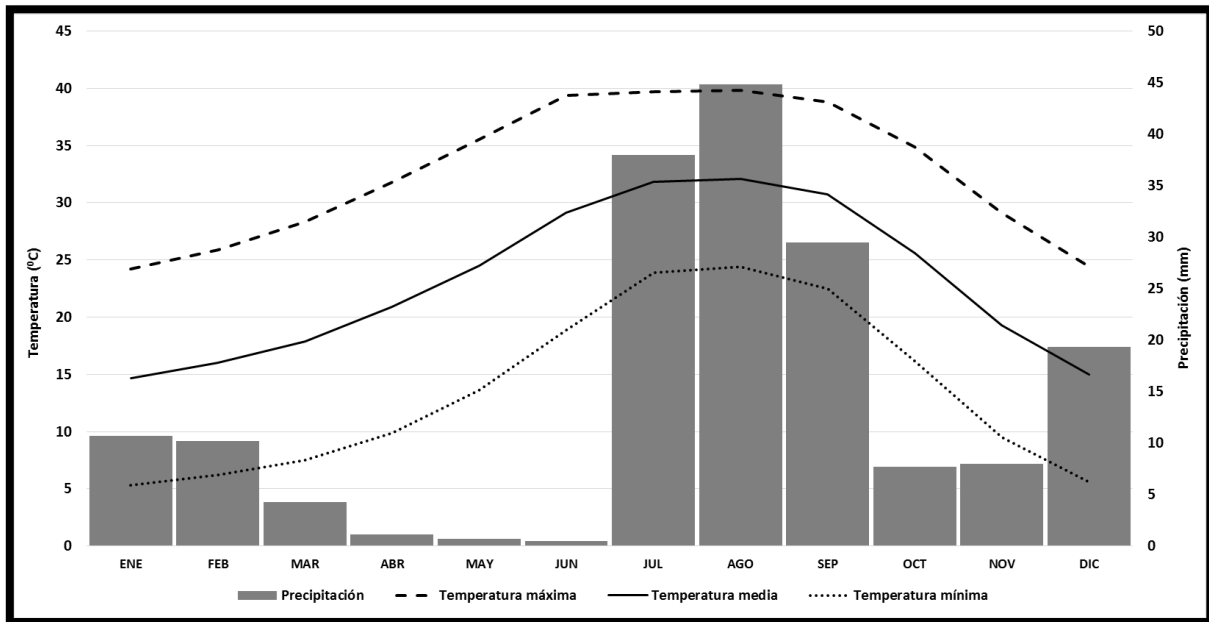
Figura 3. Climograma de la región en donde se ubica el proyecto.
