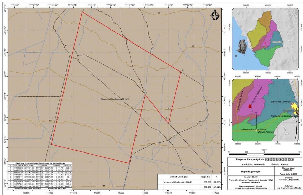
Figura 15. Geología dentro del área del proyecto "Ampliación Campo Agrícola Santa Eduwiges"
