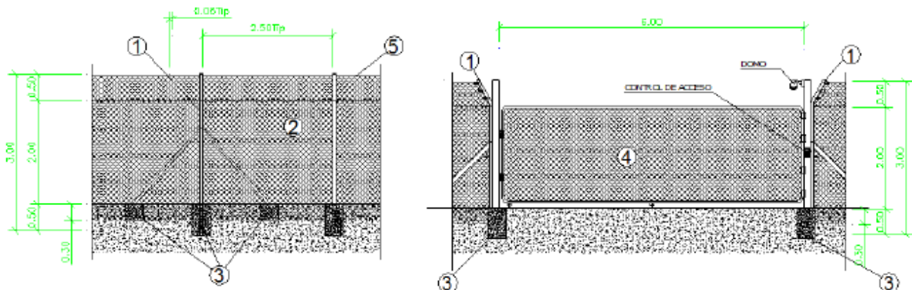
Figura. Vallado y puerta de acceso tipo
