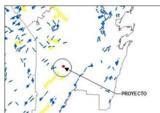
Figura 4. 8 Ubicación de un plano de fallas y fracturas con datos vectoriales del INEGI.
