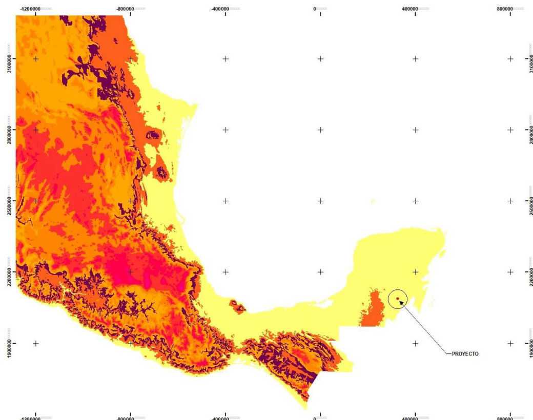
Figura 4. 7 Plano de hipsometría en la Península de Yucatán.
