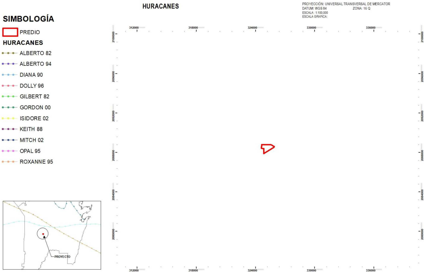
Figura 4. 3 Incidencia de huracanes en el área del proyecto.
