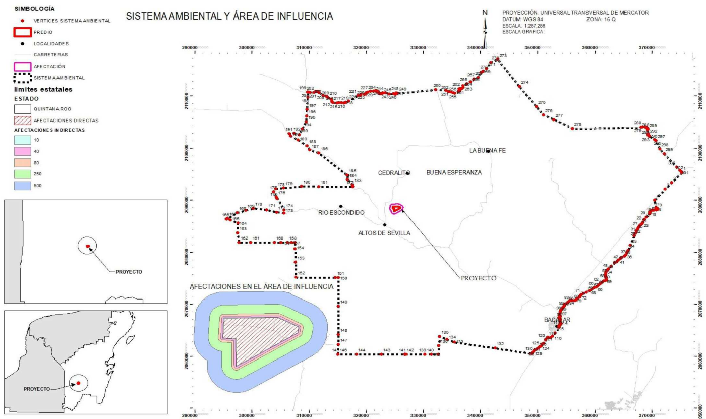
Figura 4. 1 Delimitación del sistema ambiental (SA) y del área de influencia (AI).
