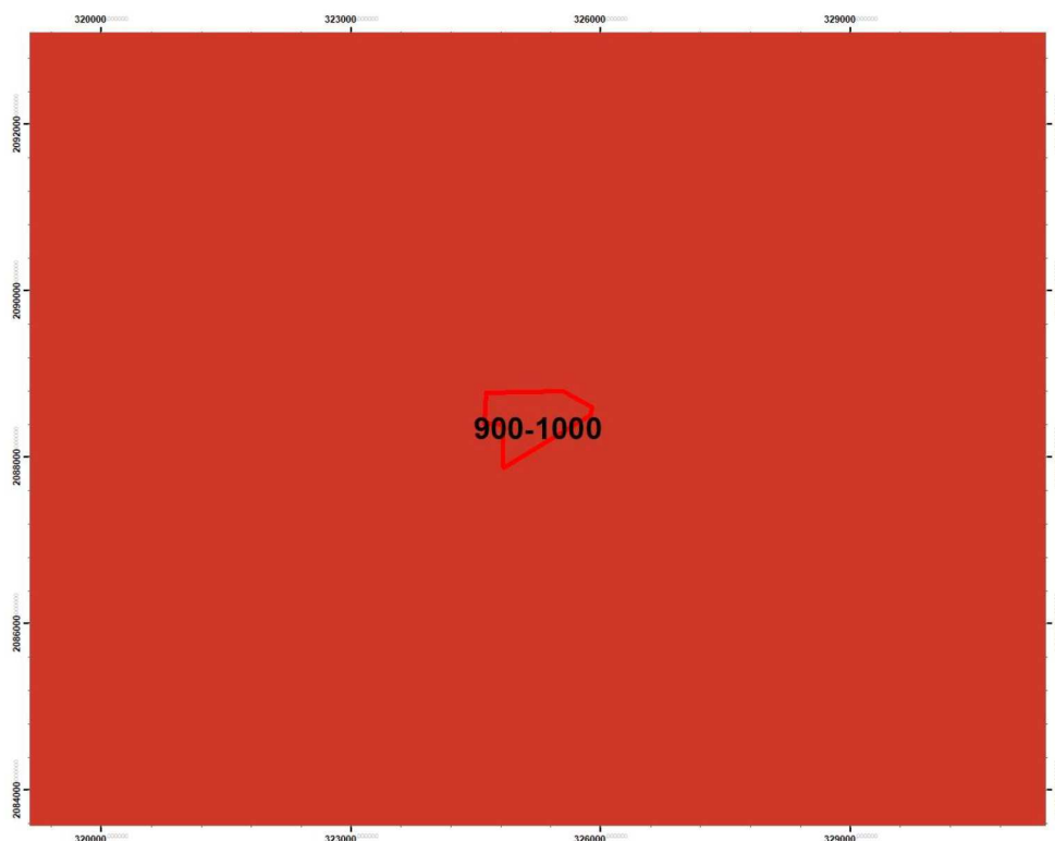
Figura 4. 2 Evapotranspiración en la zona del proyecto.
