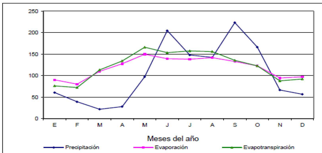
Figura 4. 1 Balance hídrico (valores en mm) en el área de estudio.
