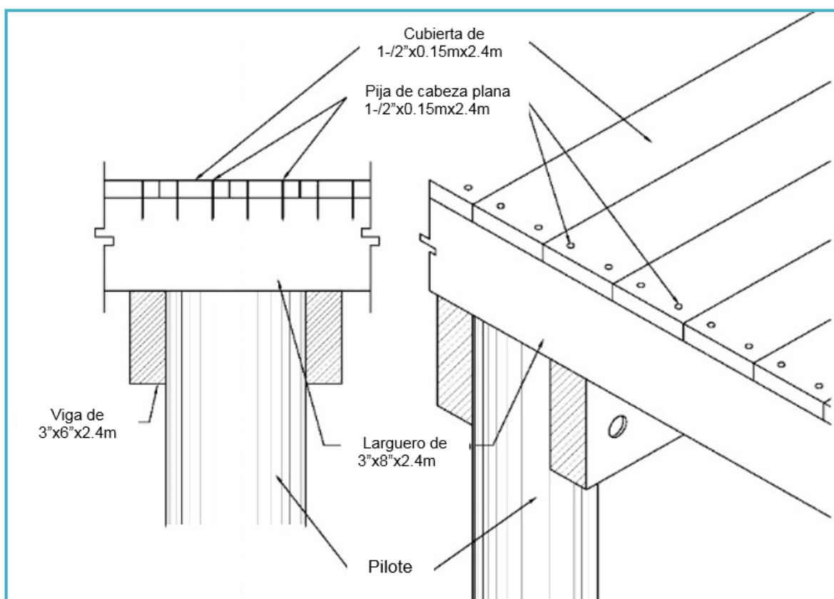
Figura II_ 32. Detalle de la cubierta de madera de los rompeolas.
