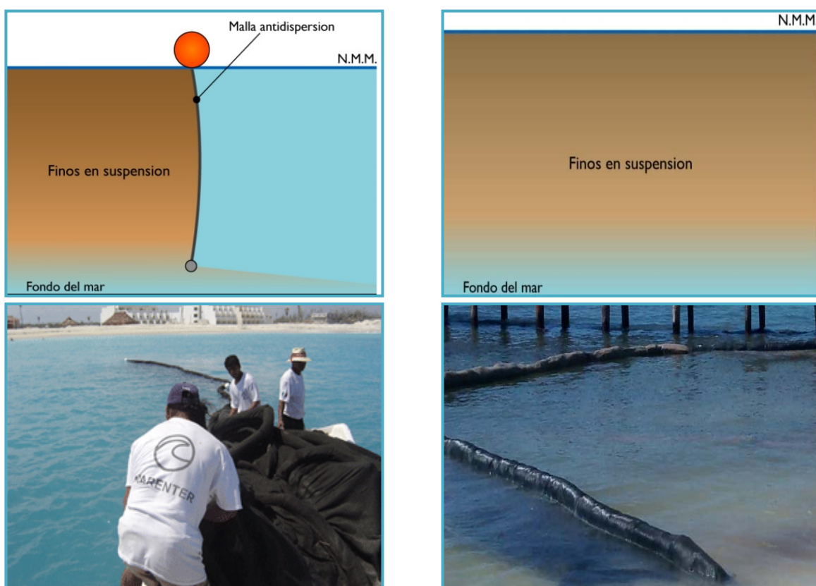
Figura II_ 24. Colocación y funcionamiento de malla antidispersión, en proyectos similares.
