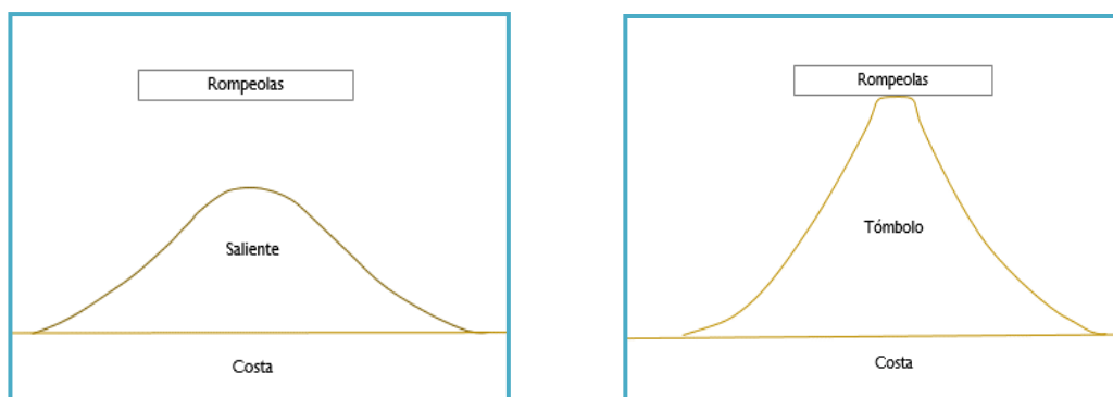
Figura II_ 12. Ejemplos de respuesta de playa con rompeolas paralelos (A Salientes, B tómbolos).
