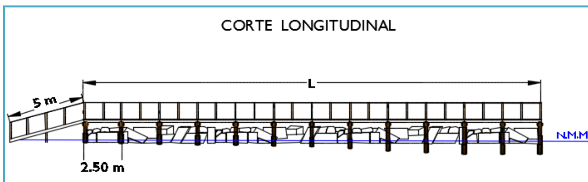
Figura II_ 14. Vista longitudinal de la terraza.
