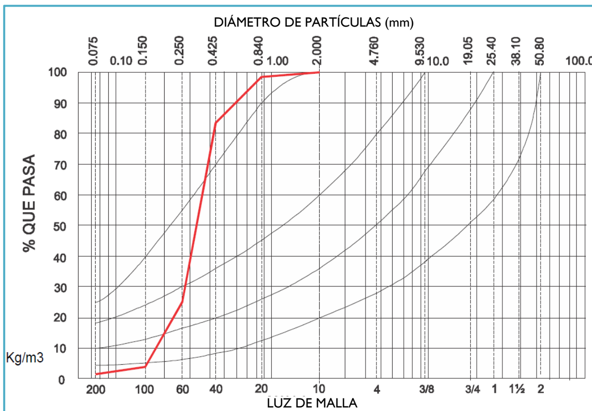
Figura IV_ 13. Análisis de la granulometría de las muestras de arena en la playa.
