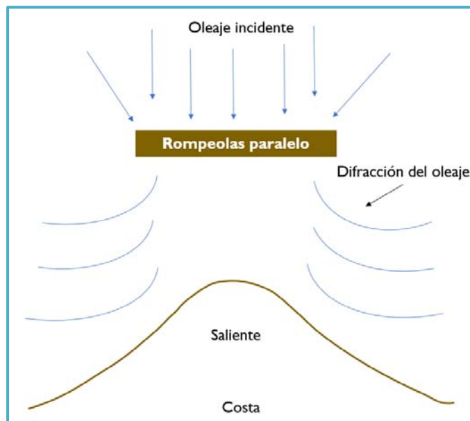
Figura II_ 11. Efecto ante la presencia de un rompeolas paralelo.
