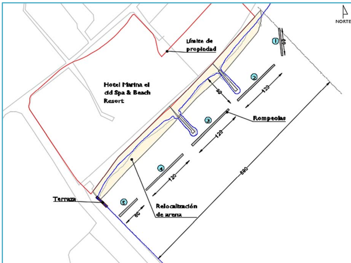
Figura VII_ 1. Plano general de obras del proyecto.
