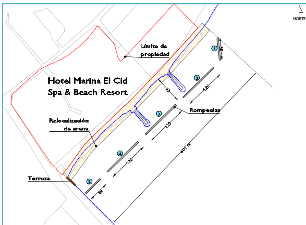
Figura II_ 2. Plano general de obras del proyecto.
