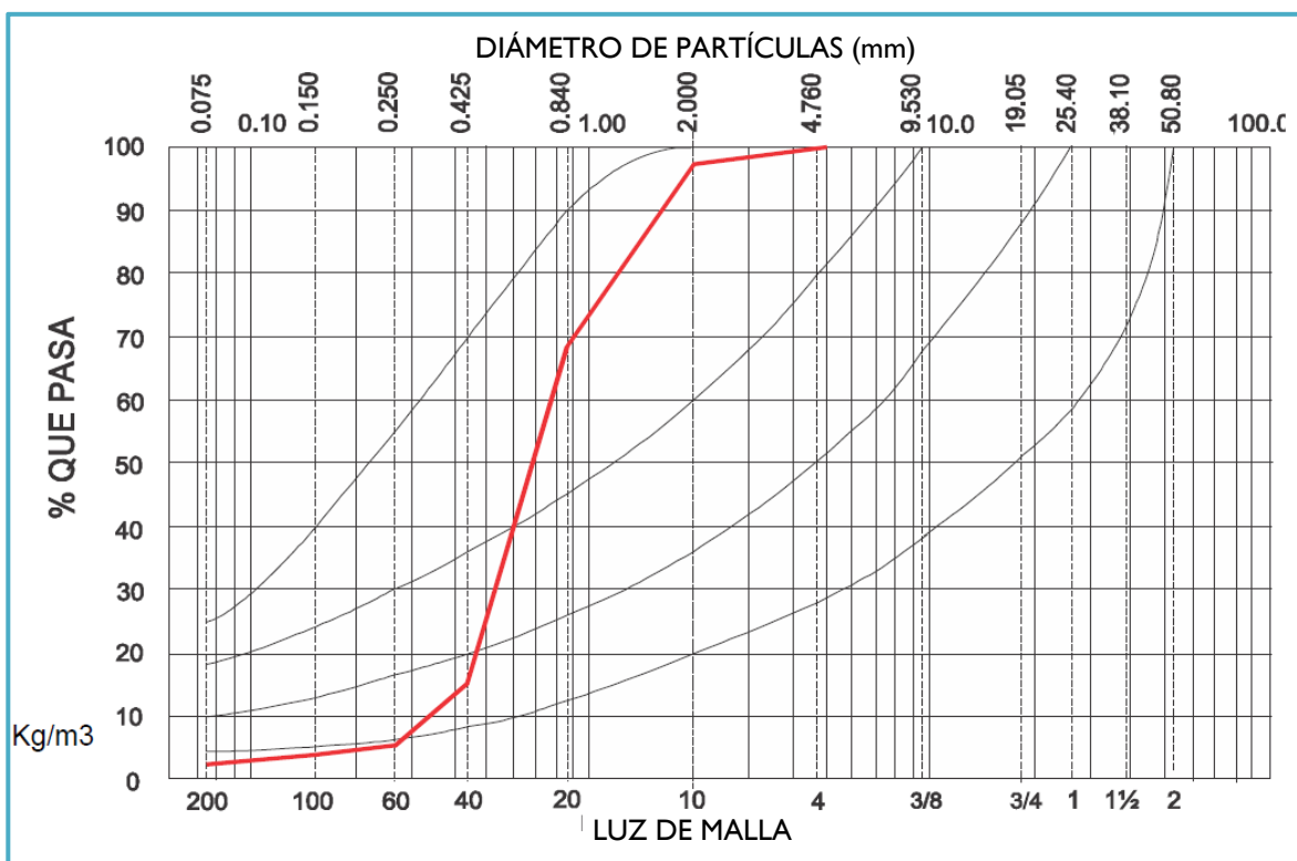
Figura IV_ 14. Análisis de la granulometría de las muestras de arena en el banco.
