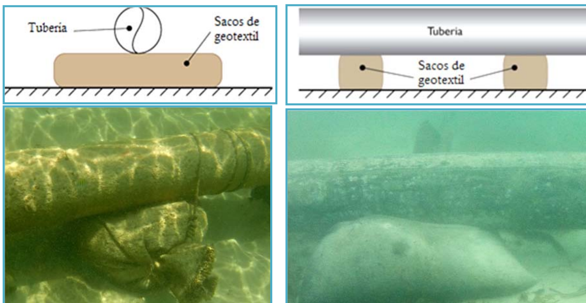
Figura II_ 23. Tuberías y mangueras con lastre de proyectos similares.
