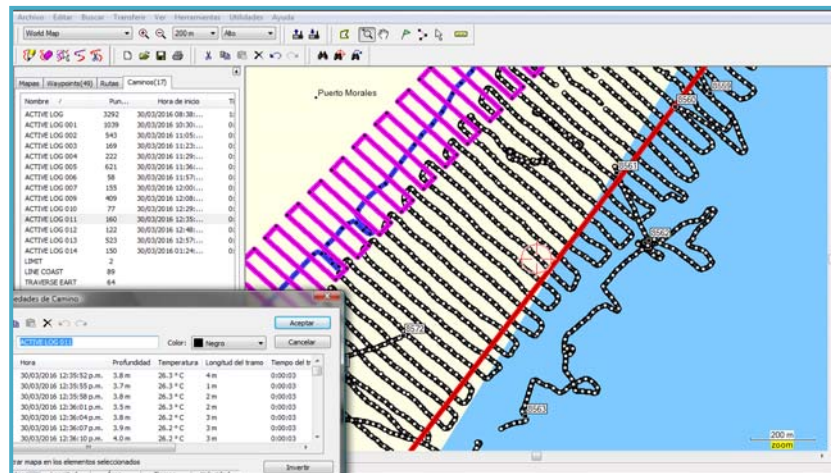
Figura IV_ 10. Transectos batimétricos y áreas de mapeo analizados con Power Nav GNSS.
