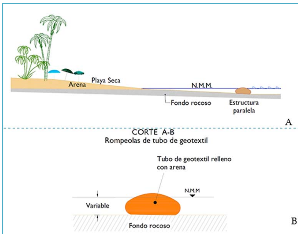
Figura II_ 18. Diseño de rompeolas. A) Corte longitudinal B) Corte transversal.
