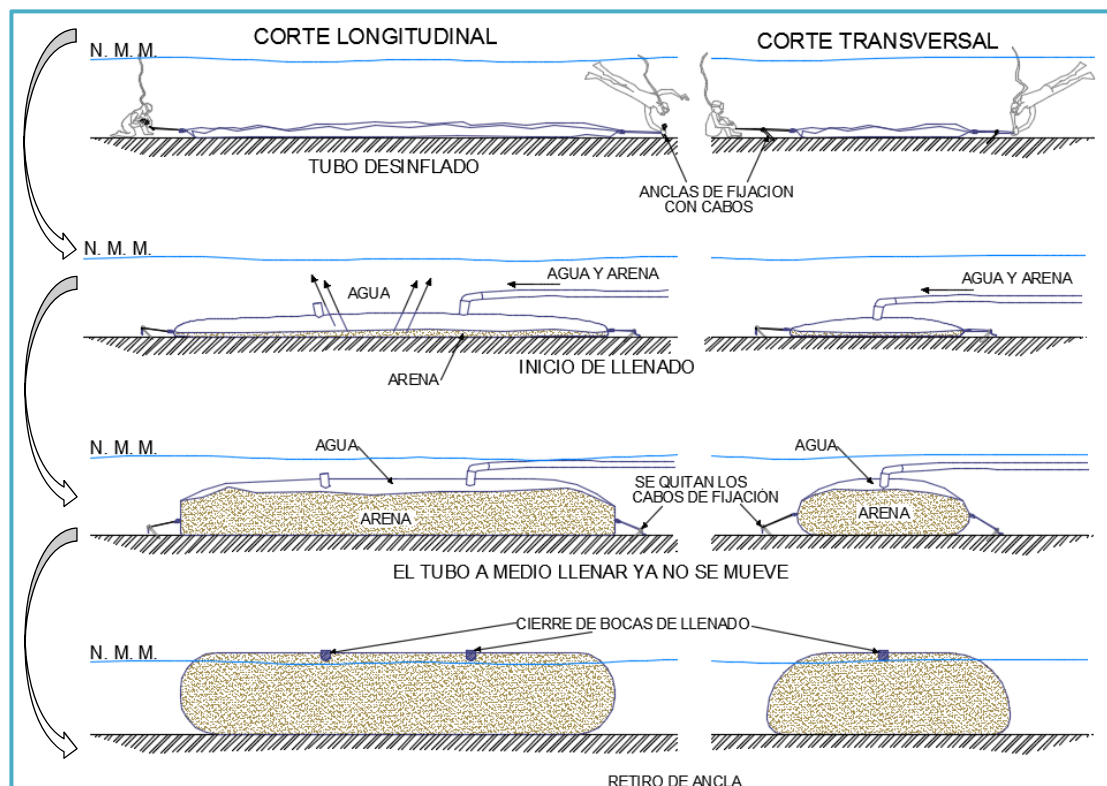
Figura II_ 21. Proceso típico de desplante de un rompeolas.
