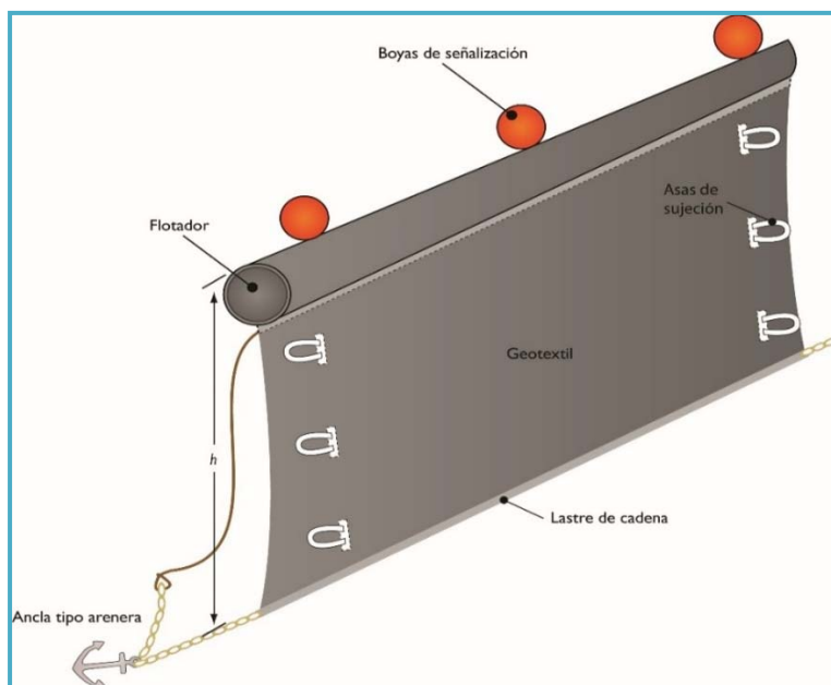
Figura II_ 25. Diseño de la malla de geotextil antidispersión.
