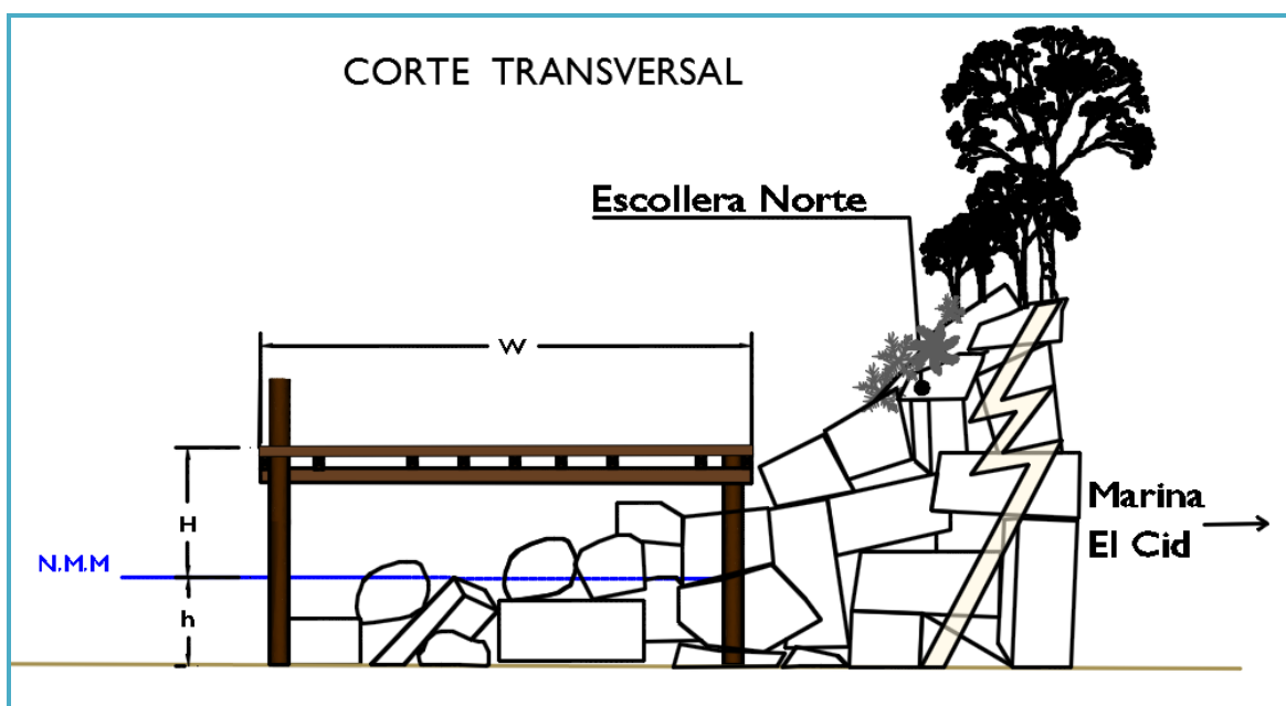
Figura II_ 29. Corte de la terraza
