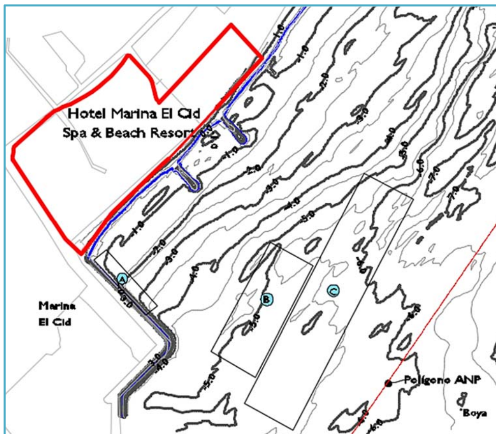
Figura II_9. Polígonos con las zonas de disposición de arena aprovechables al frente del proyecto.
