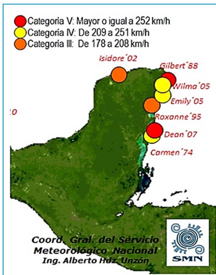
Figura IV_ 9. Huracanes intensos desde 1970.
