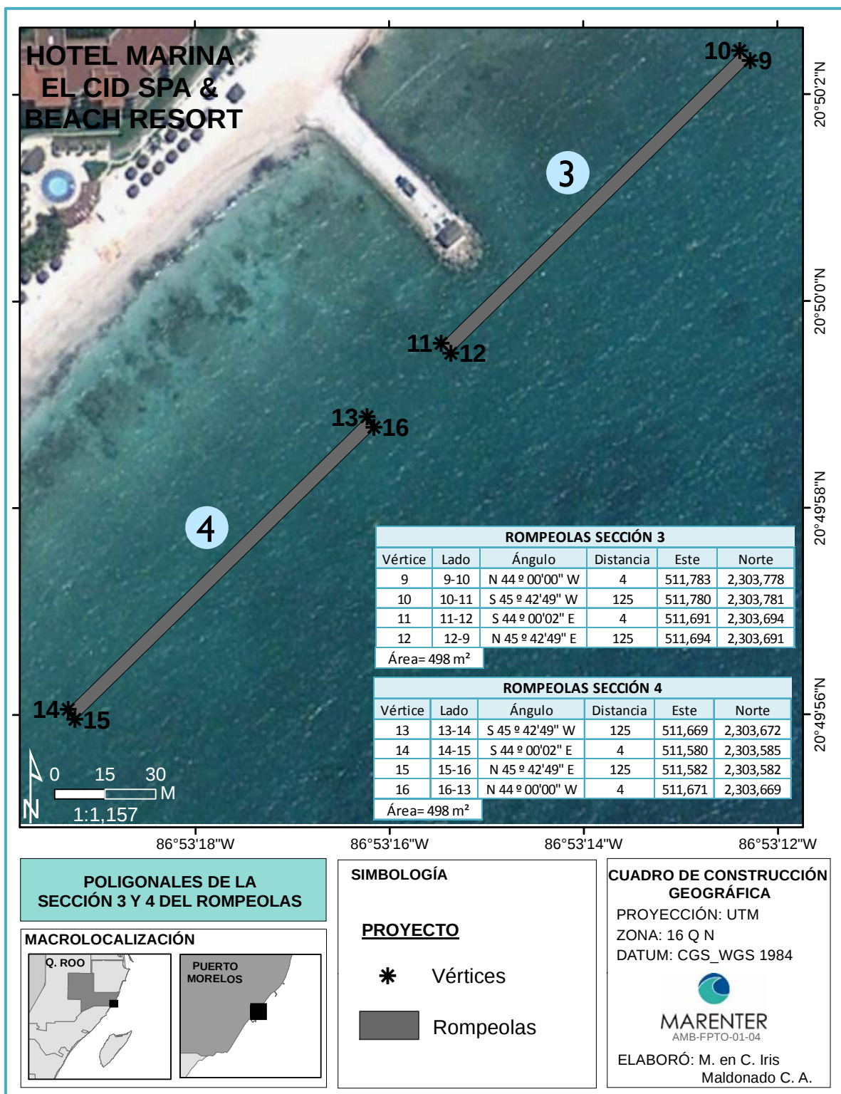
Figura II_ 5. Mapa con los cuadros de construcción en coordenadas UTM de las secciones de rompeolas 3 y 4.
