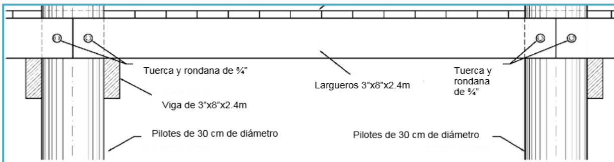
Figura II_ 30. Detalle longitudinal de la estructura de conexión.
