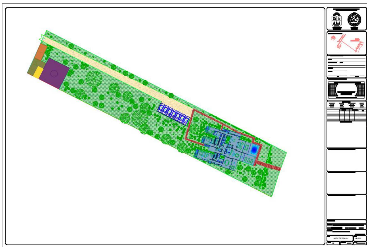
Imagen II.3.- Planta de conjunto de las obras
