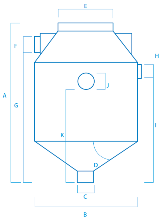
Figura II.8. Dimensiones
