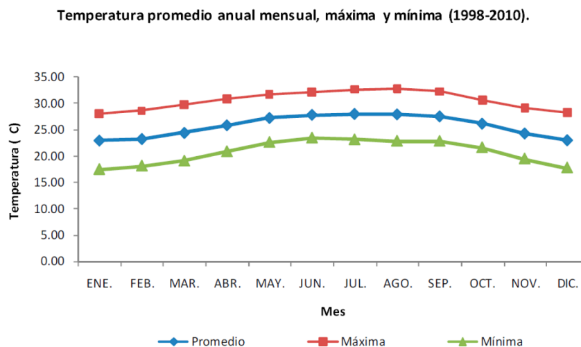
Figura IV.2. Temperatura promedio mensual media, mínima y máxima. La gráfica permite apreciar el rango de temperatura registrado en la zona a lo largo del lapso de 1998-2010 (Fuente: CONAGUA, Estación meteorológica 23163 CNA, Playa del Carmen).
