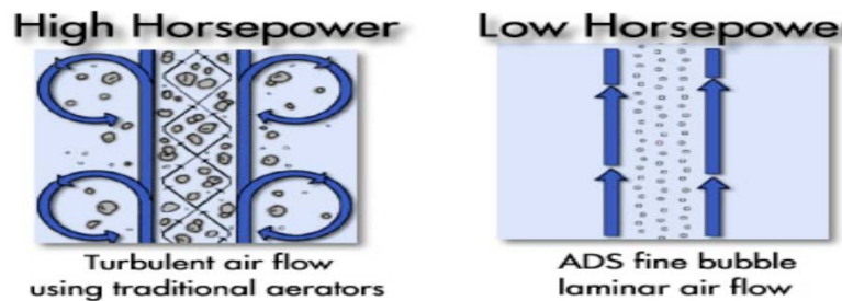
Figura VI.3. Ventajas del ADS sobre aireación convencional.
