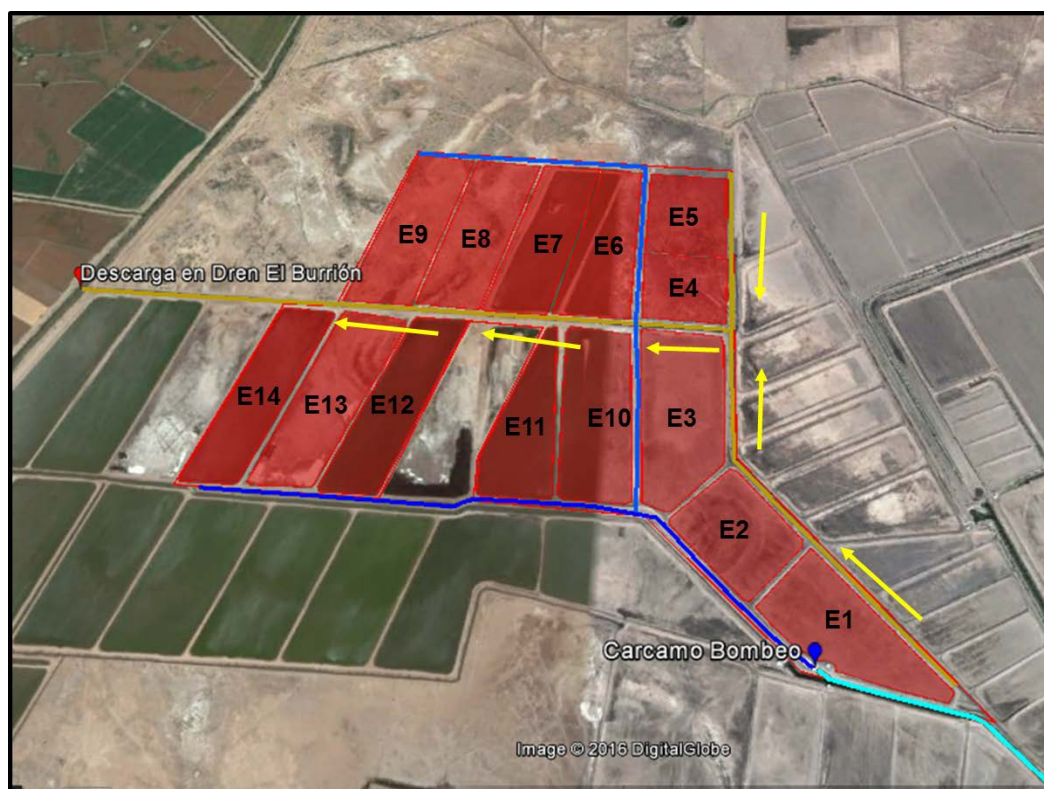
Figura II.1. Distribución de estanques (■), canal de llamada (—), reservorio (—), drenes (—) y flujo de agua (→) en la granja Sociedad Cooperativa Acuícola Aguila-socho, S. de R.L. de C.V. (La Brecha)
