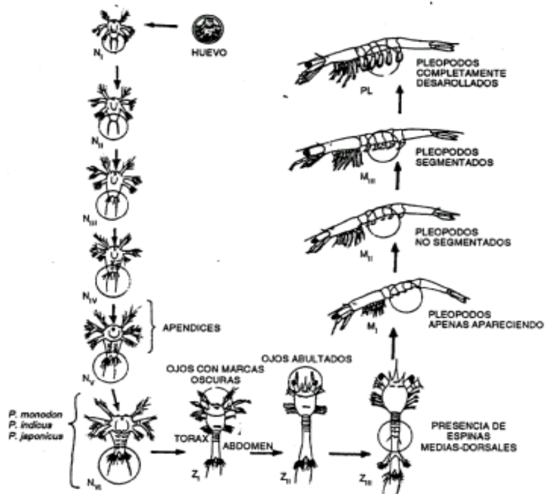
Figura II.9. Desarrollo larvarios general del camarón (PENAEIDAE).
