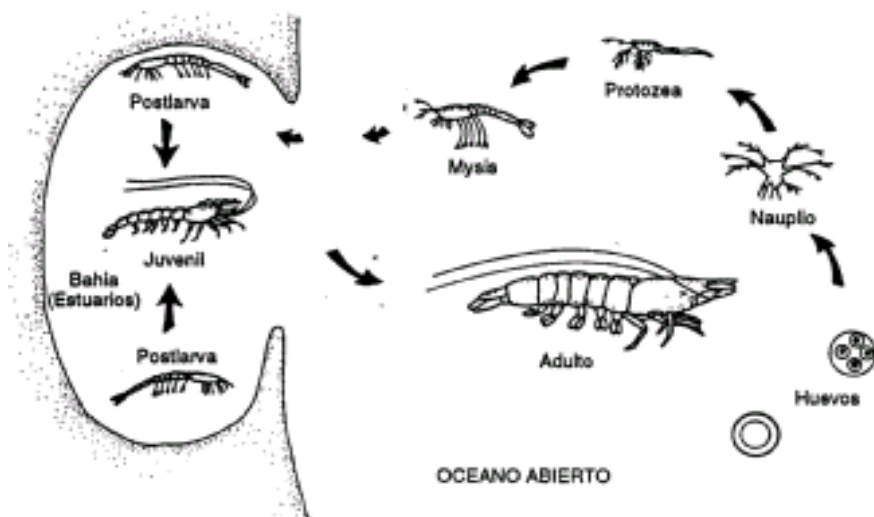
Figura II.8. Ciclo de vida (PENAEIDAE).
