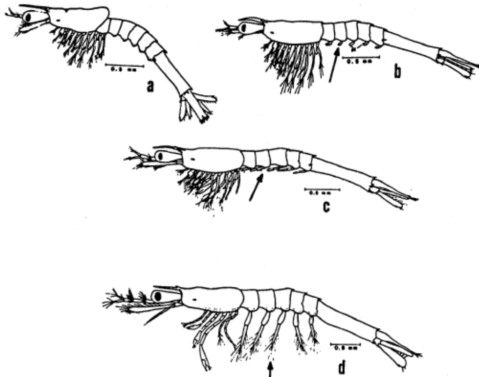
Figura II.10. Subetapas mysis y postlarval del Penaeus duorarum : P1 – pleópodo (en Dobkin, 1961). a) Mysis I: Estructura semejante al camarón; b) Mysis II: Presencia de pleópodos no segmentados; c) Mysis III: Pleópodos alargados y segmentados; d) Postlarva I: (PL1): Las setas de natación presente en pleópodos.
