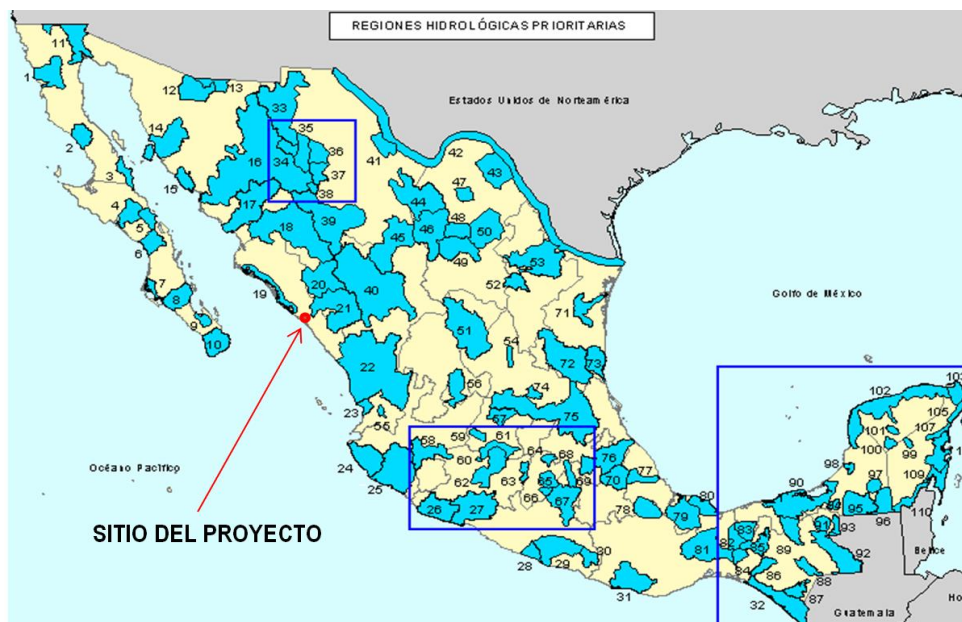
Imagen III.2. Ubicación del sitio de proyecto con respecto a las Regiones Hidrológicas Prioritarias (RHP).
