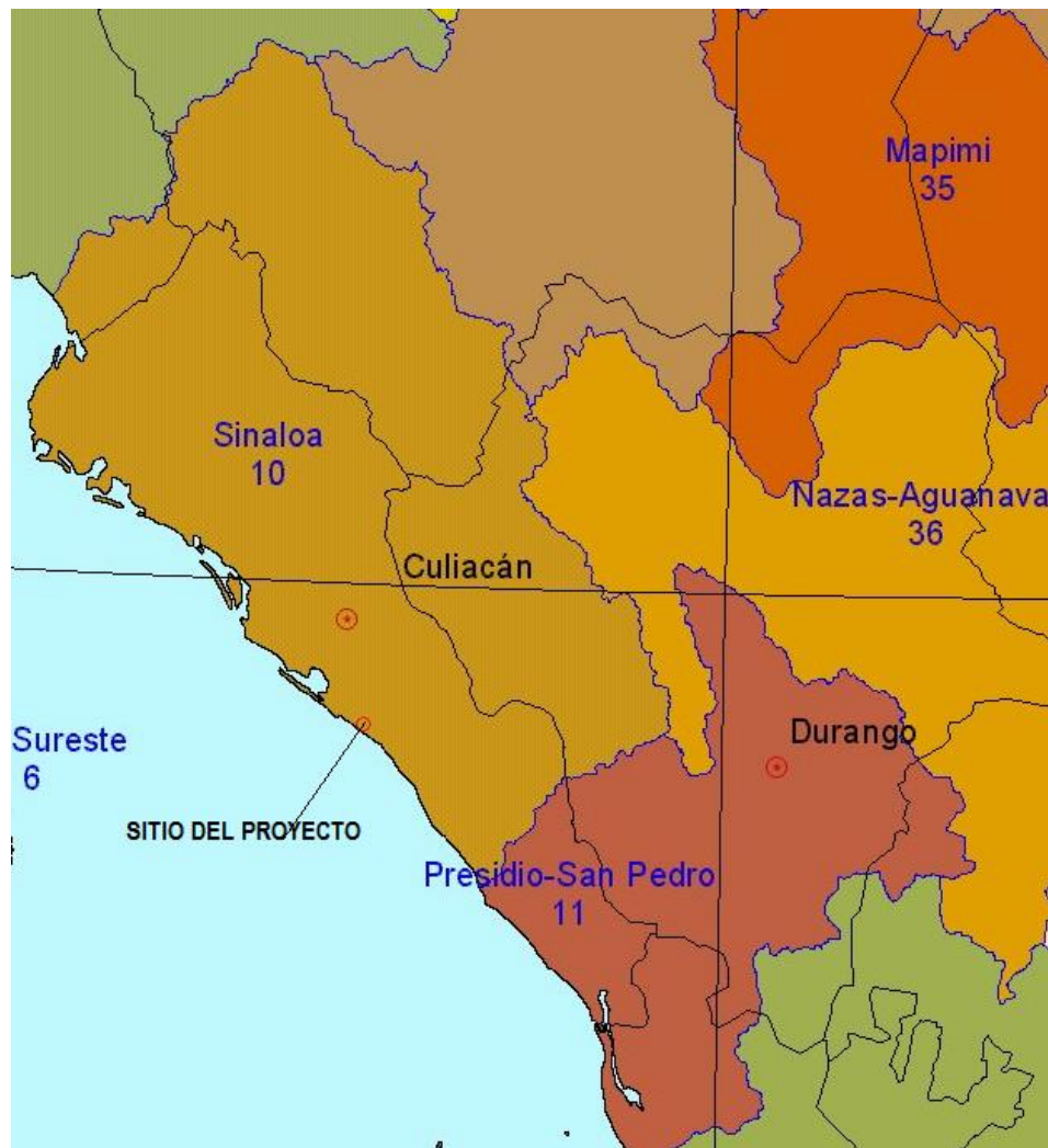
Imagen. Región Hidrológica
