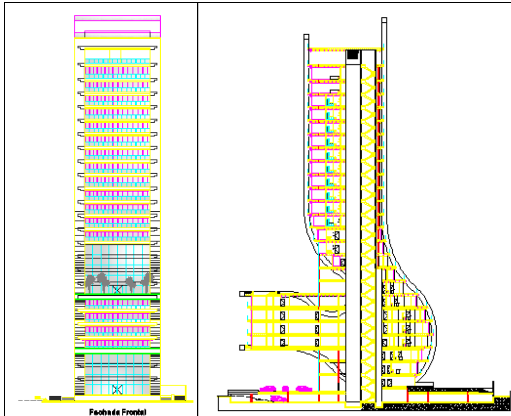
FIGURA 5. TORRE LUZ FACHADA DE LADO Y FRONTAL.
