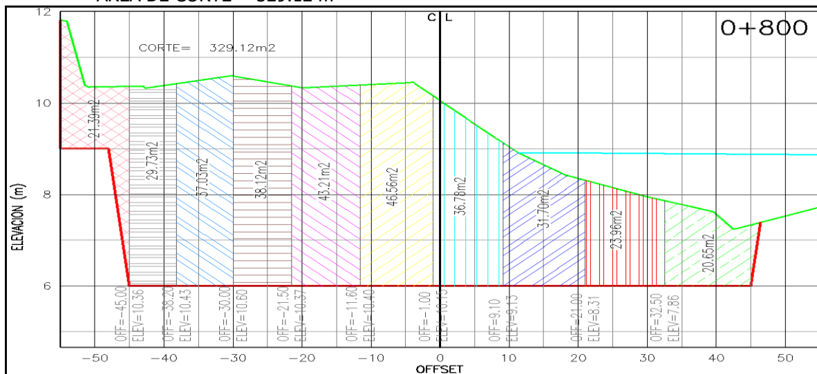
Figura 4.- ESTACION 0+800.000 (Parte final del proyecto):
