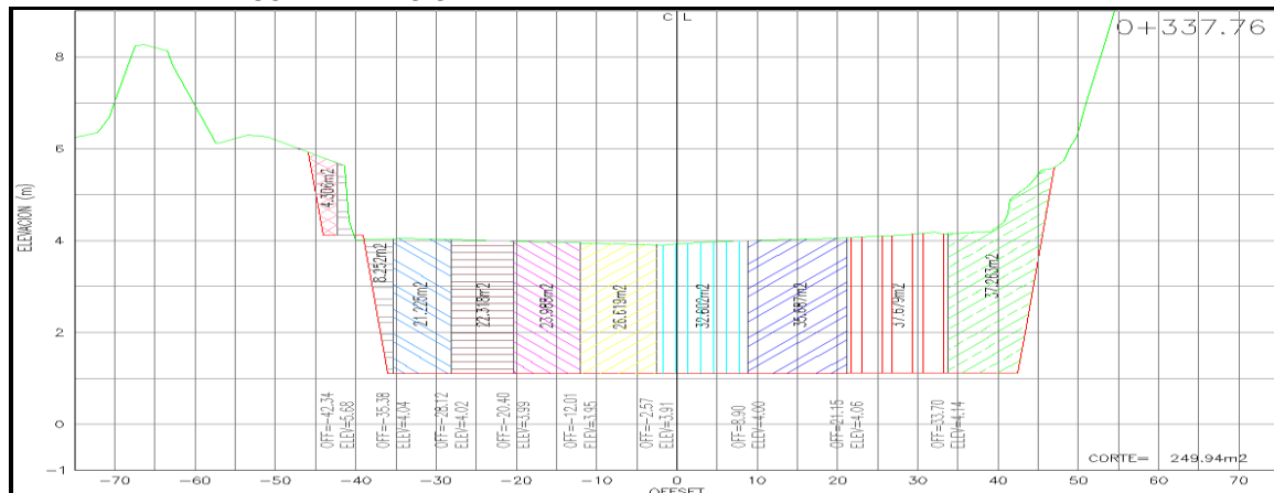
Figura 4.- ESTACION 0+775.000 (Parte final del proyecto): AREA DE TERRAPLEN = 0.000 m 2 AREA DE CORTE = 249.94 m 2
