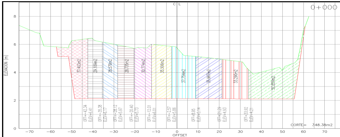
Figura 2.- ESTACION 0+0.000 (Aguas más arriba del proyecto): AREA DE TERRAPLEN = 0.000 m 2 AREA DE CORTE = 348.38 m 2
