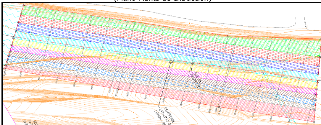
Figura 8.- 10 frentes de extracción divididos en 21 estaciones o secciones. (Plano Planta de extracción)
