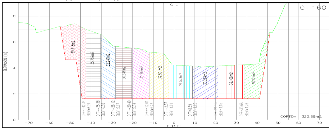
Figura 3.- ESTACION 0+600.000 (Parte central del proyecto): AREA DE TERRAPLEN = 0.000 m 2 AREA DE CORTE = 322.69 m 2
