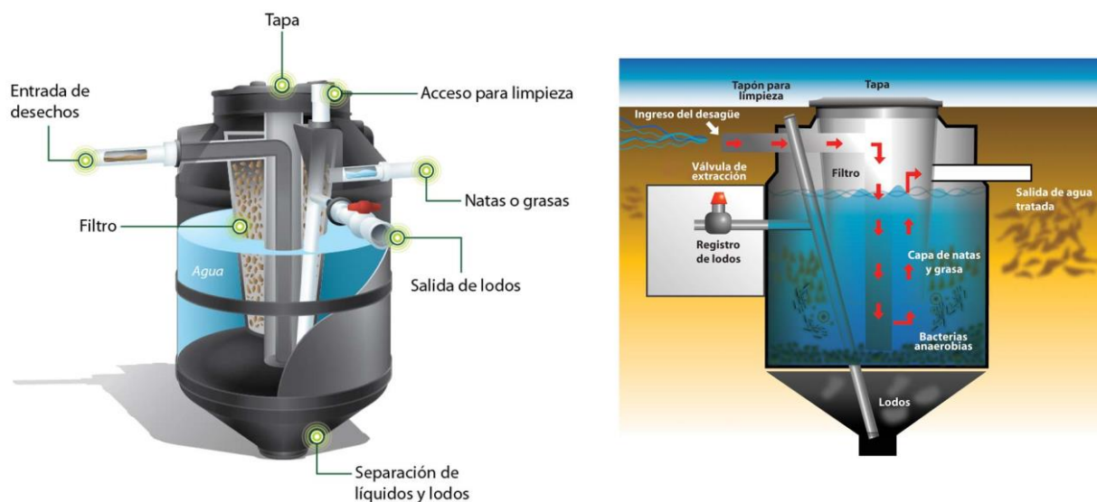
Ilustración 53.- Detalle Biodigestor
