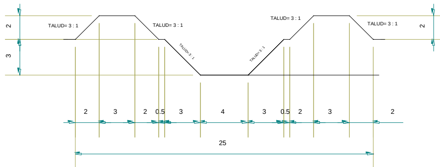
Ilustración 47.- Secciones de Bordos
