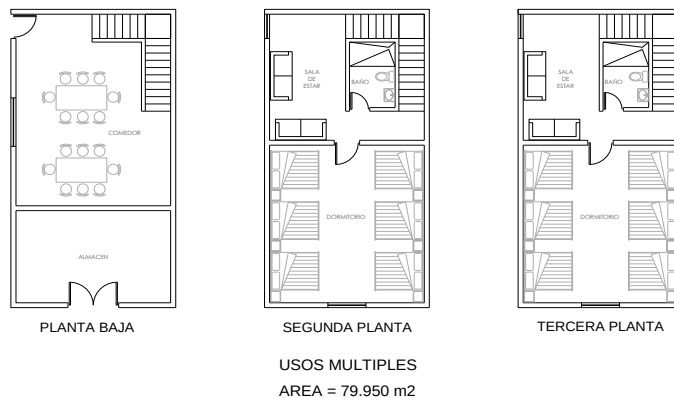
Ilustración 22.- Cuarto de usos múltiples.
