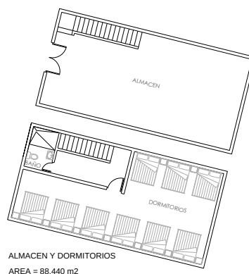
Ilustración 23.- Diseño de Dormitorio-Almacén.
