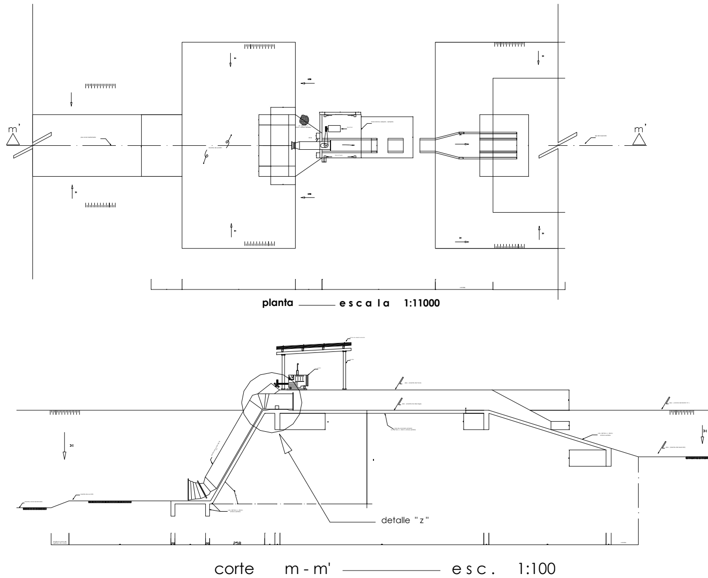
Ilustración 46.- Bombeo ingeniería
