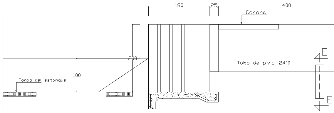
Ilustración 55.- Detalle Ingeniería Compuertas
