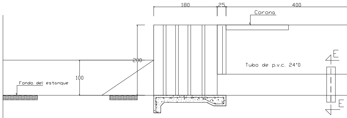
Ilustración 47.- Detalle Ingeniería Compuertas
