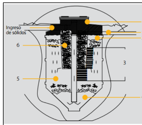
Ilustración 46.- Mecanismo Biodigestor
