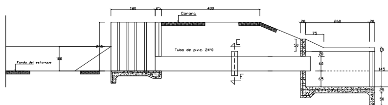
CORTE A-A
