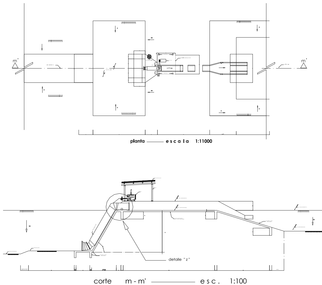
Ilustración 14.- Ingeniería cárcamo de bombeo.
