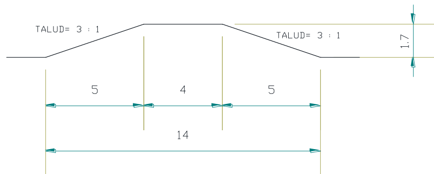
Ilustración 20.- Detalle de bordería del reservorio.
