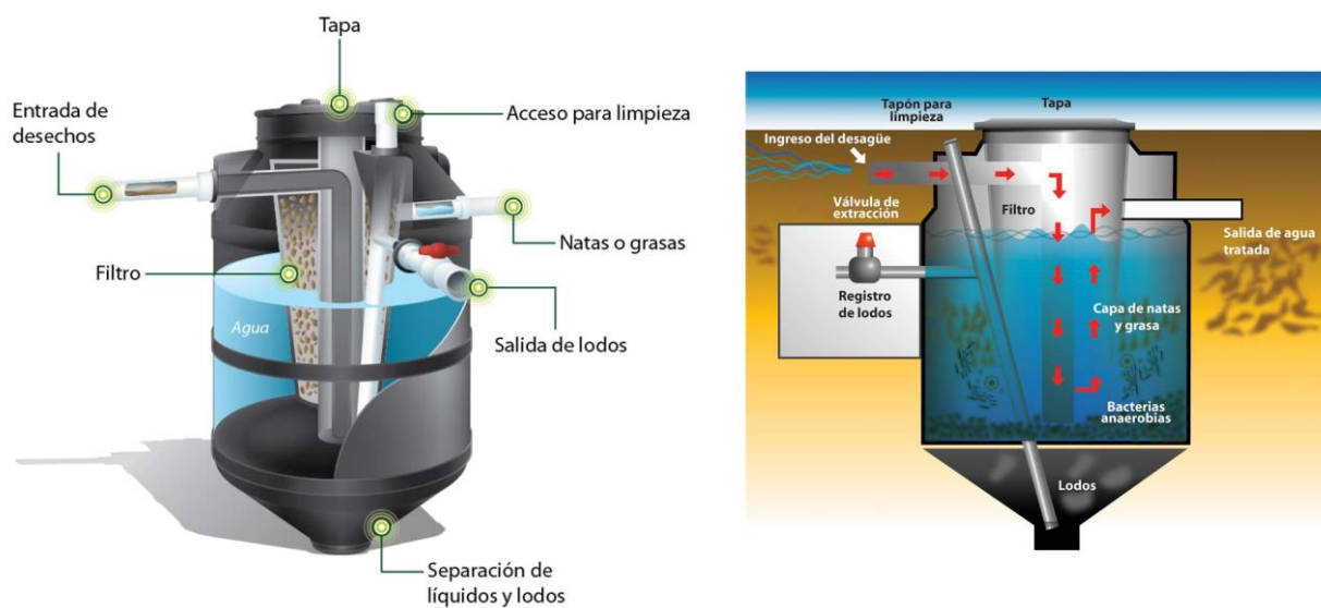
Ilustración 45.- Detalle Biodigestor
