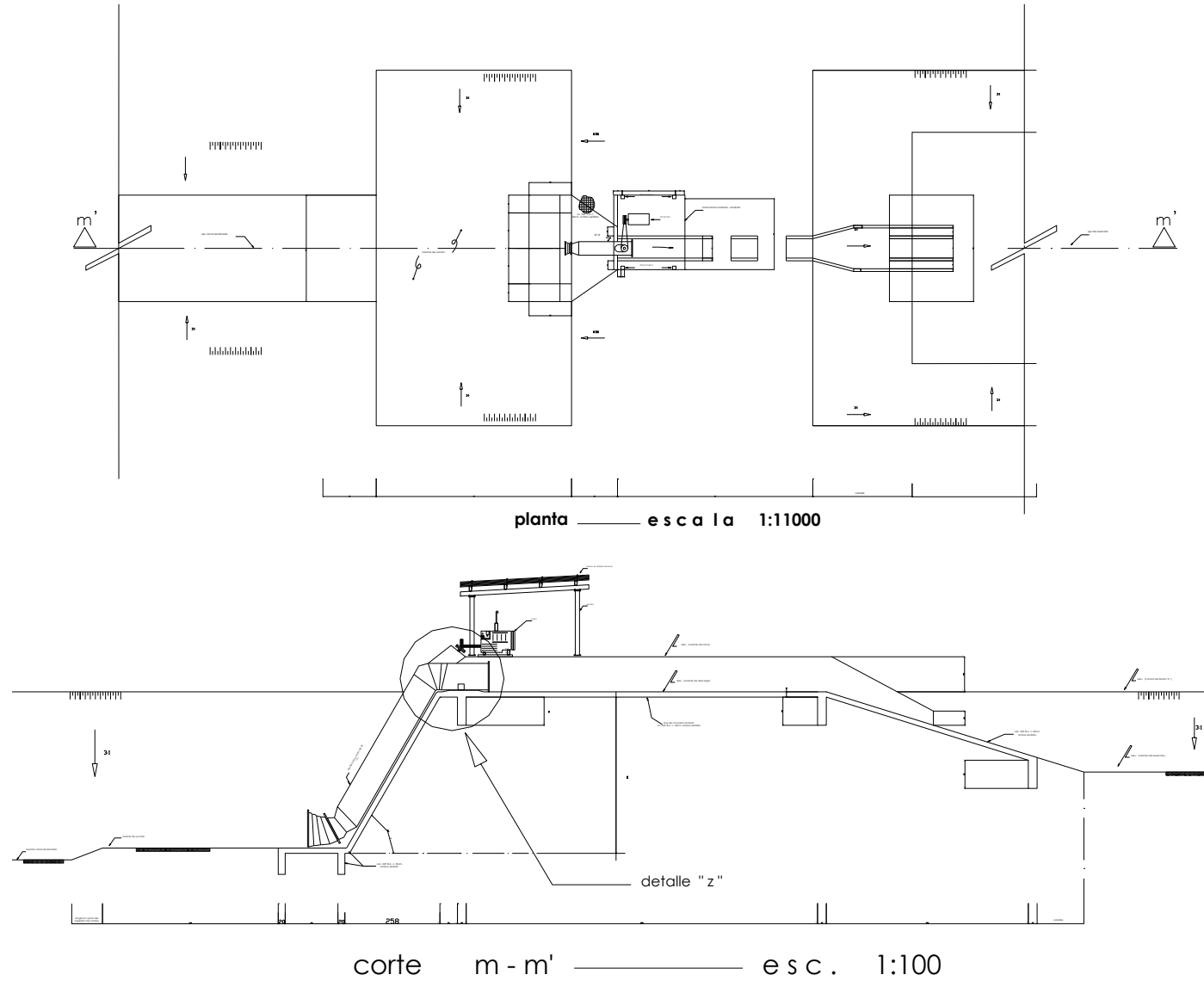
Ilustración 40.- Bombeo ingeniería
