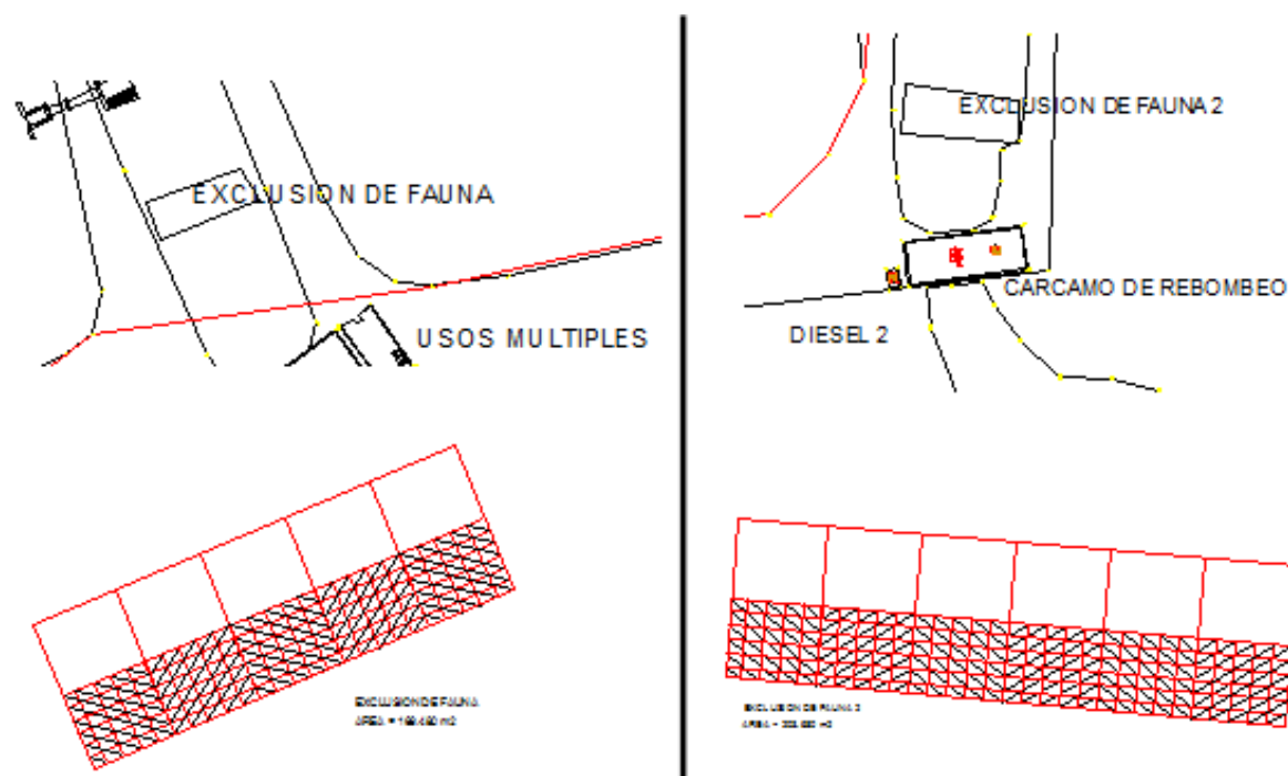
Ilustración 21.- Diseño de los sistemas excluyores de fauna acuática.
