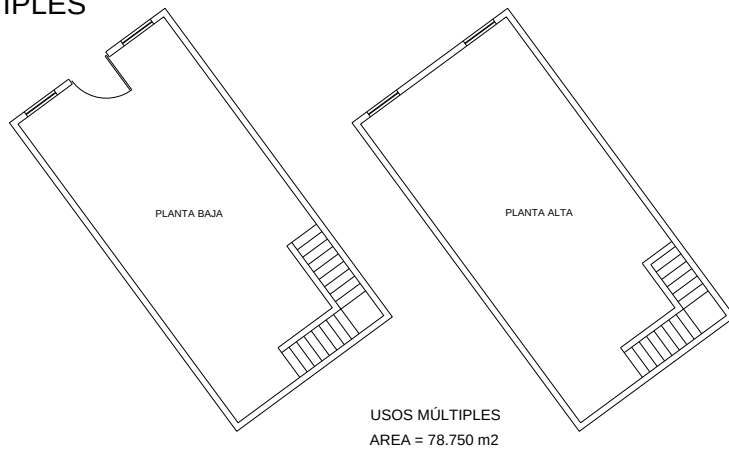
Ilustración 23.- Diseño de cuarto de usos variados (múltiples).
