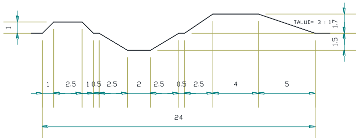
Ilustración 18.- Dren de descarga
