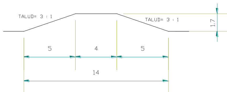
Ilustración 17.- Polígonos de construcción de reservorio
