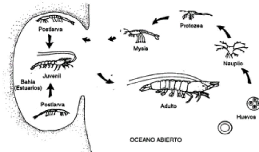
Figura II.5. Ciclo de vida (PENAEIDAE)
