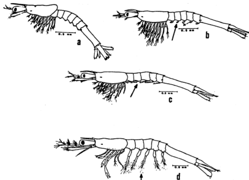
Figura II.10. Subetapas mysis y postlarval del Penaeus duorarum : P1 – pleópodo (en Dobkin, 1961). a) Mysis I: Estructura semejante al camarón; b) Mysis II: Presencia de pleópodos no segmentados; c) Mysis III: Pleópodos alargados y segmentados; d) Postlarva I: (PL1): Las setas de natación presente en pleópodos.
