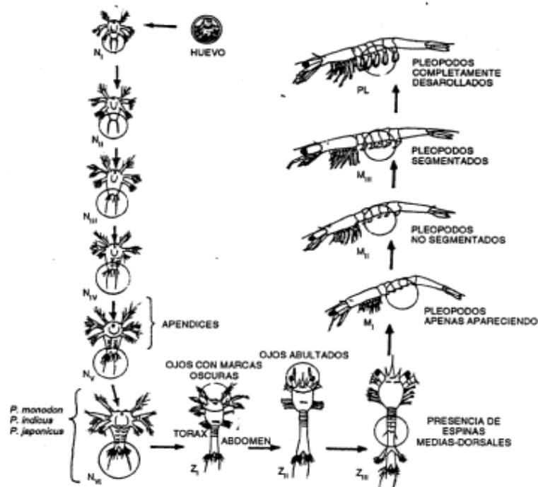
Figura II.6. Desarrollo larvarios general del camarón (PENAEIDAE)
