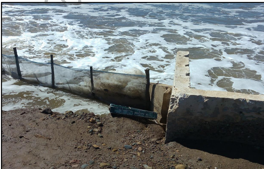
Fotografía No. 9. Malla en el canal de llamada que filtra el agua de desechos vegetales y evita la entrada de fauna de gran talla.
