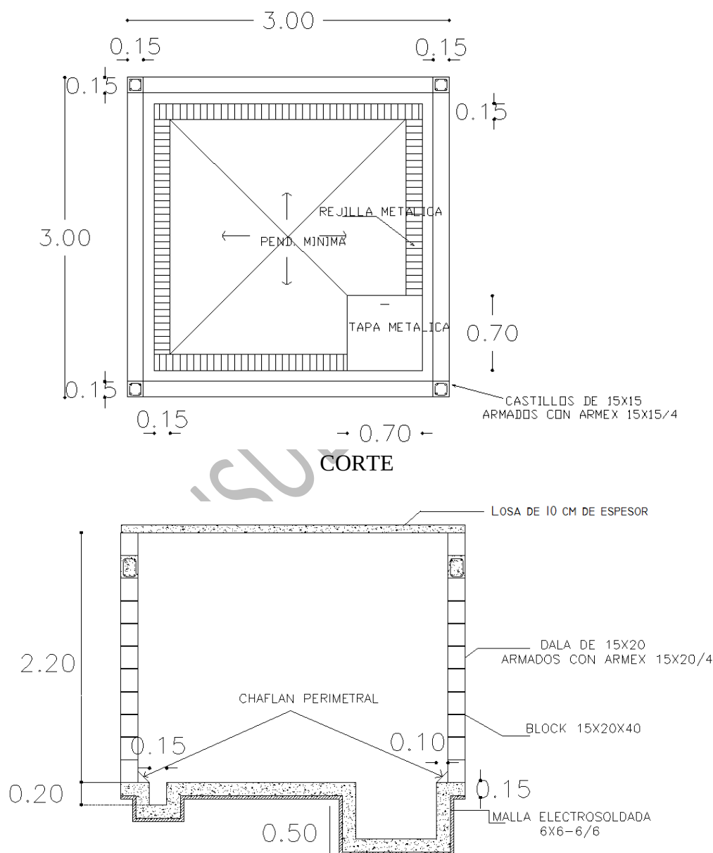
Planta de Almacén de Residuos Peligrosos.
