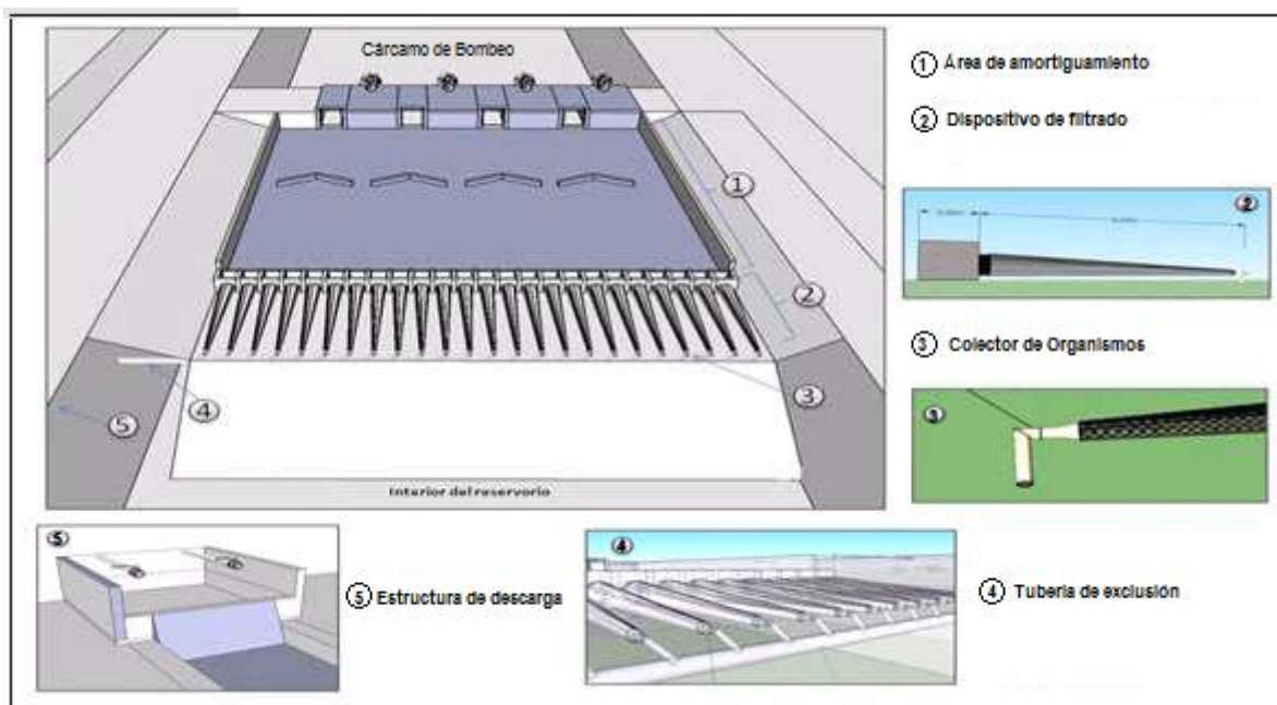
Figura 5.-Esquema general del SEFA-3 que consiste en la adaptación del área de amortiguamiento en el reservorio.
