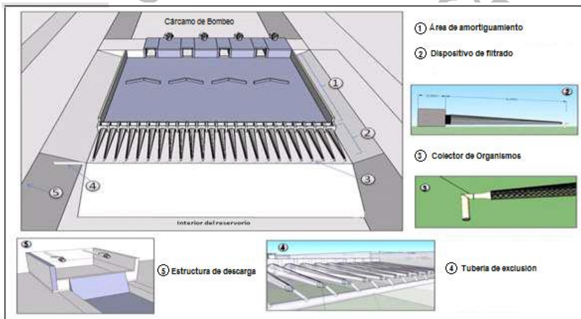
Figura 21.- Esquema general del SEFA-3 que consiste en la adaptación del área de amortiguamiento en una piscina, pileta o reservorio.
