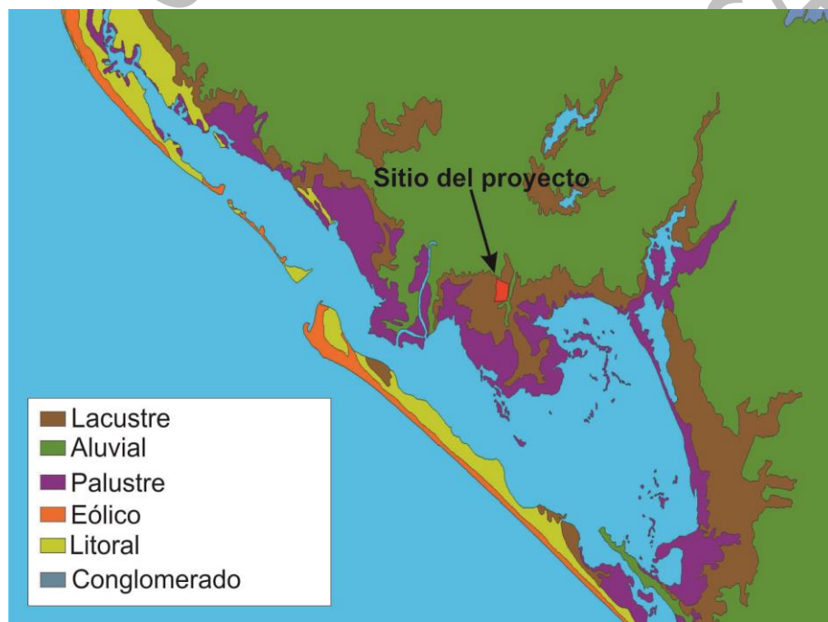
Figura 15.-Geología del área de la presente MIA-P.
