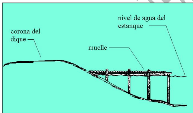
Figura 8.-Vista lateral de un muelle para toma de parámetros de calidad del agua.
