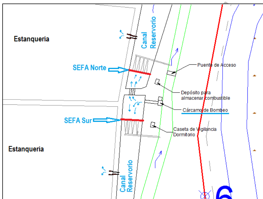
Figura 20.- Ubicación de los Sistemas Excluidores de Fauna Acuática.
