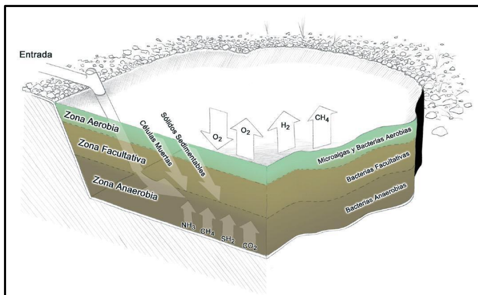
Figura 6.- Esquema del ciclo natural de la laguna de oxidación; Autor: ITC, Instituto Tecnológico de Canarias
