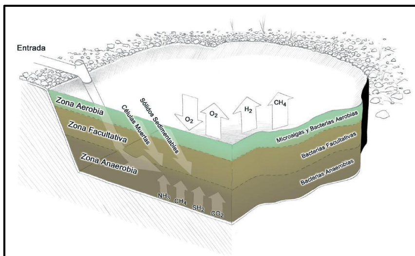
Imagen 19. Esquema del ciclo natural de la laguna de oxidación; Autor: ITC, Instituto Tecnológico de Canarias
