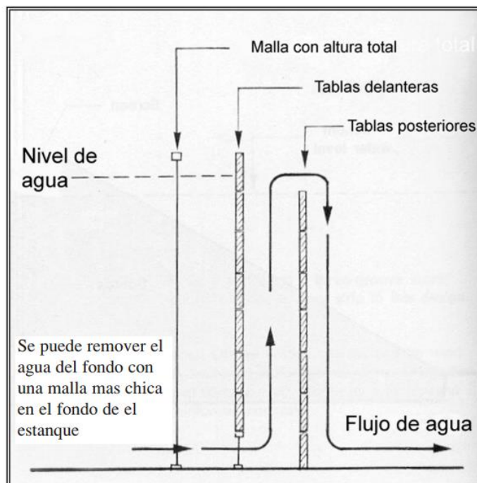
Figura 8. Vista lateral de una estructura de drenaje, muestra la ubicación correcta de la malla y el uso de las tablas para controlar el nivel del drenaje.
