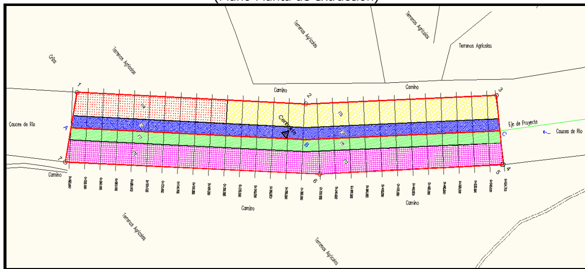
Figura 8.- 5 frentes de extracción divididos en 29 estaciones o secciones. (Plano Planta de extracción)
