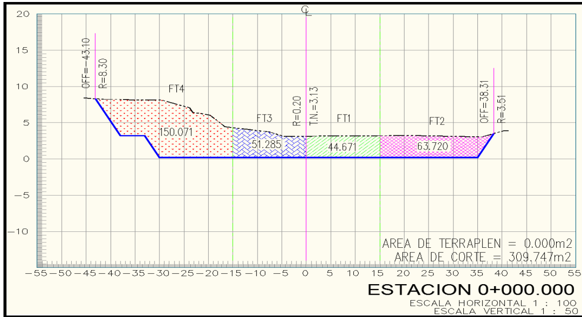
Figura 2.- ESTACION 0+000.000 (Aguas más arriba del proyecto): AREA DE TERRAPLEN = 0.000 m 2 AREA DE CORTE = 309.747 m 2
