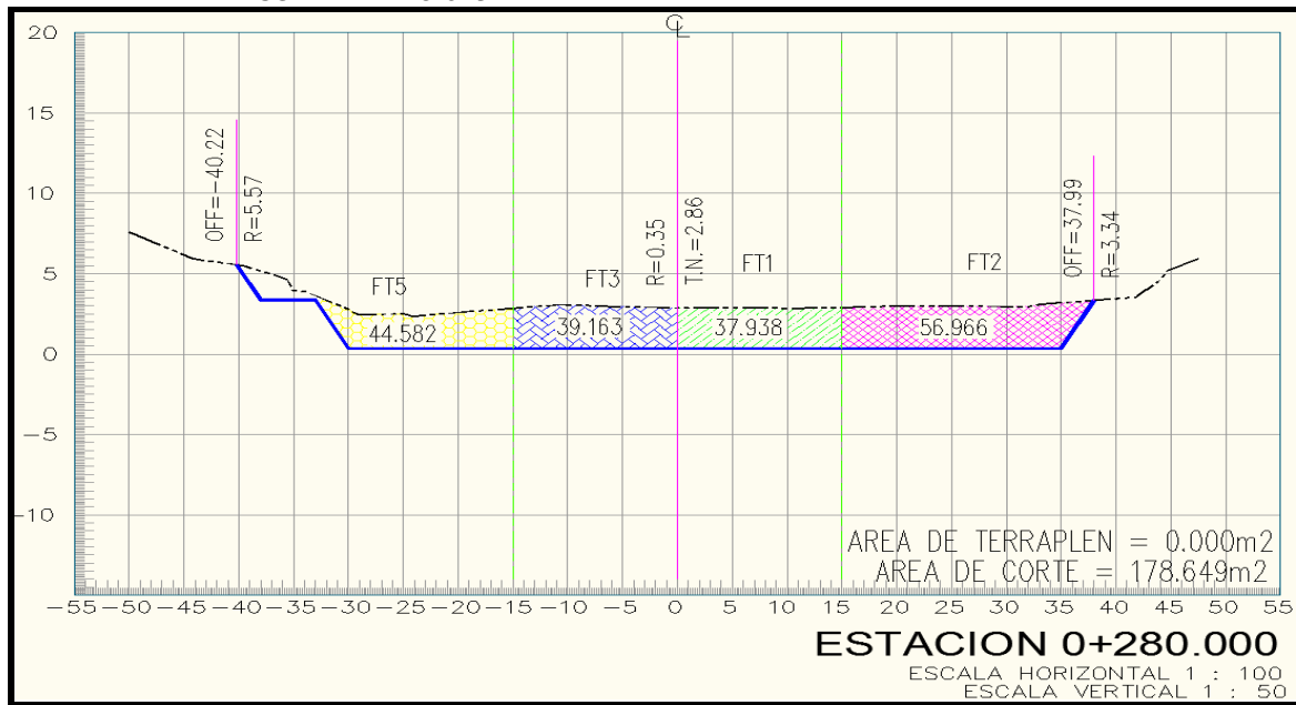
Figura 3.- ESTACION 0+280.000 (Parte central del proyecto): AREA DE TERRAPLEN = 0.000 m 2 AREA DE CORTE = 178.649 m 2
