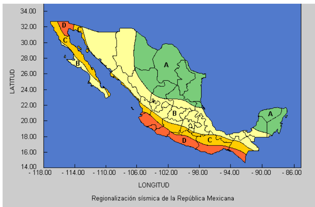
Regiones sísmicas en la República Mexicana
