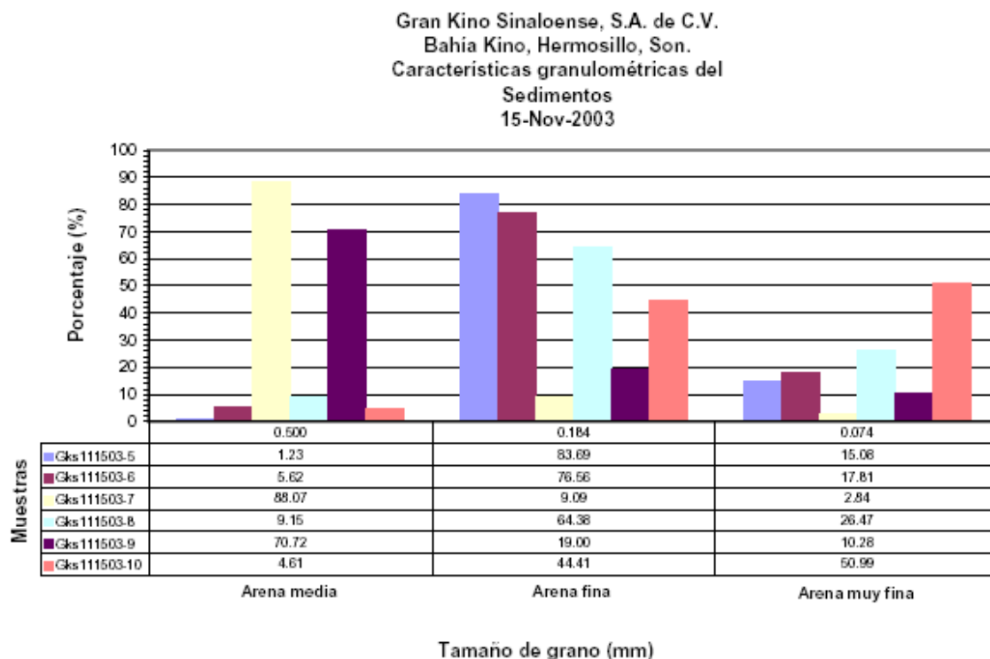
Figura 27. Distribución de tamaño de granos en sedimentos (2 de 2)
