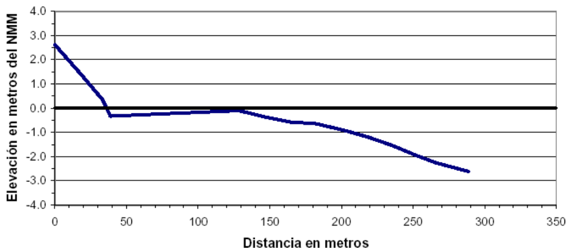
Figura 6. Perfil playero 0+500 noviembre 2003
