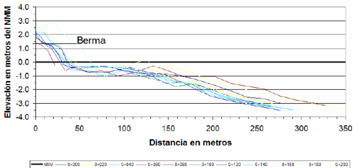
Figura 10. Perfiles playeros de Enero 2004.
