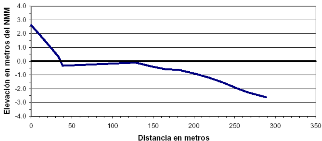
Figura 5. Perfil playero 0+000 noviembre 2003
