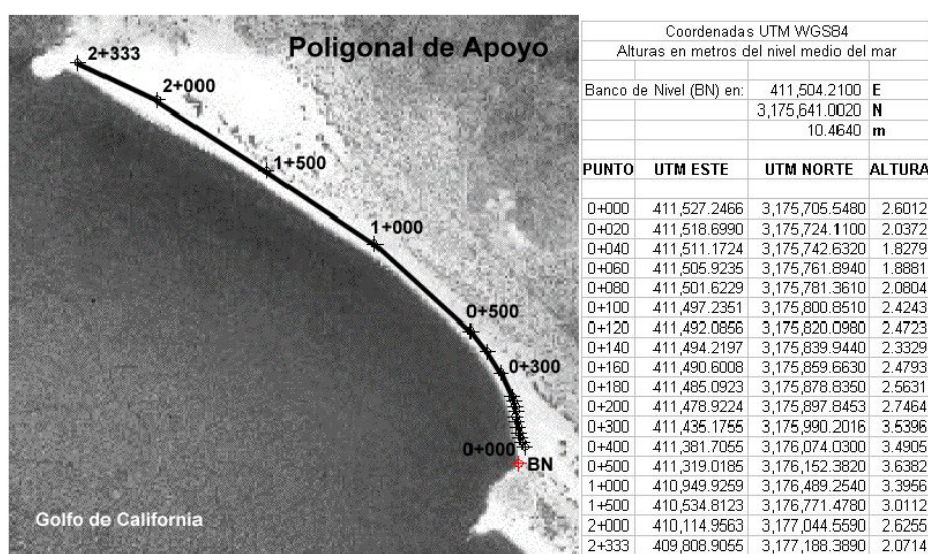
Figura 1 Poligonal de apoyo
