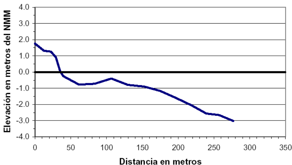
Figura 8. Perfil playero 0+000 enero 2004
