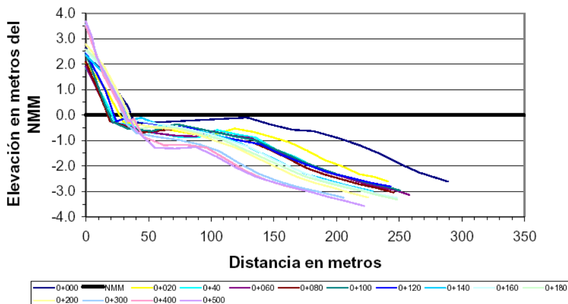
Figura 7. Perfiles playeros Noviembre 2003
