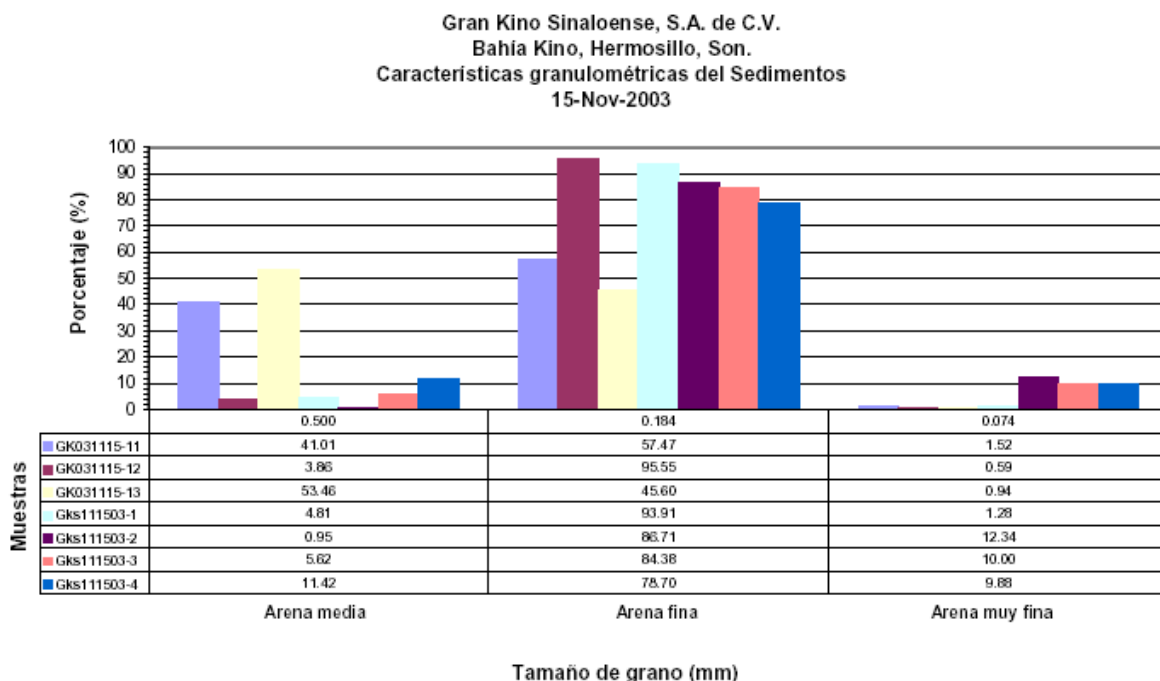
Figura 26. Distribución de tamaño de granos en sedimentos (1 de 2)
