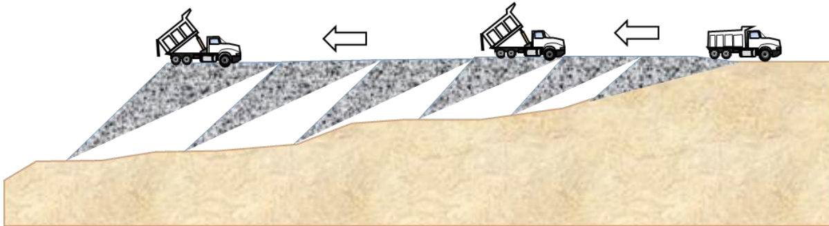
Figura II-10. Representación gráfica del vaciado en forma de cascada sistemática para la disposición del suelo estéril (tepetate).
