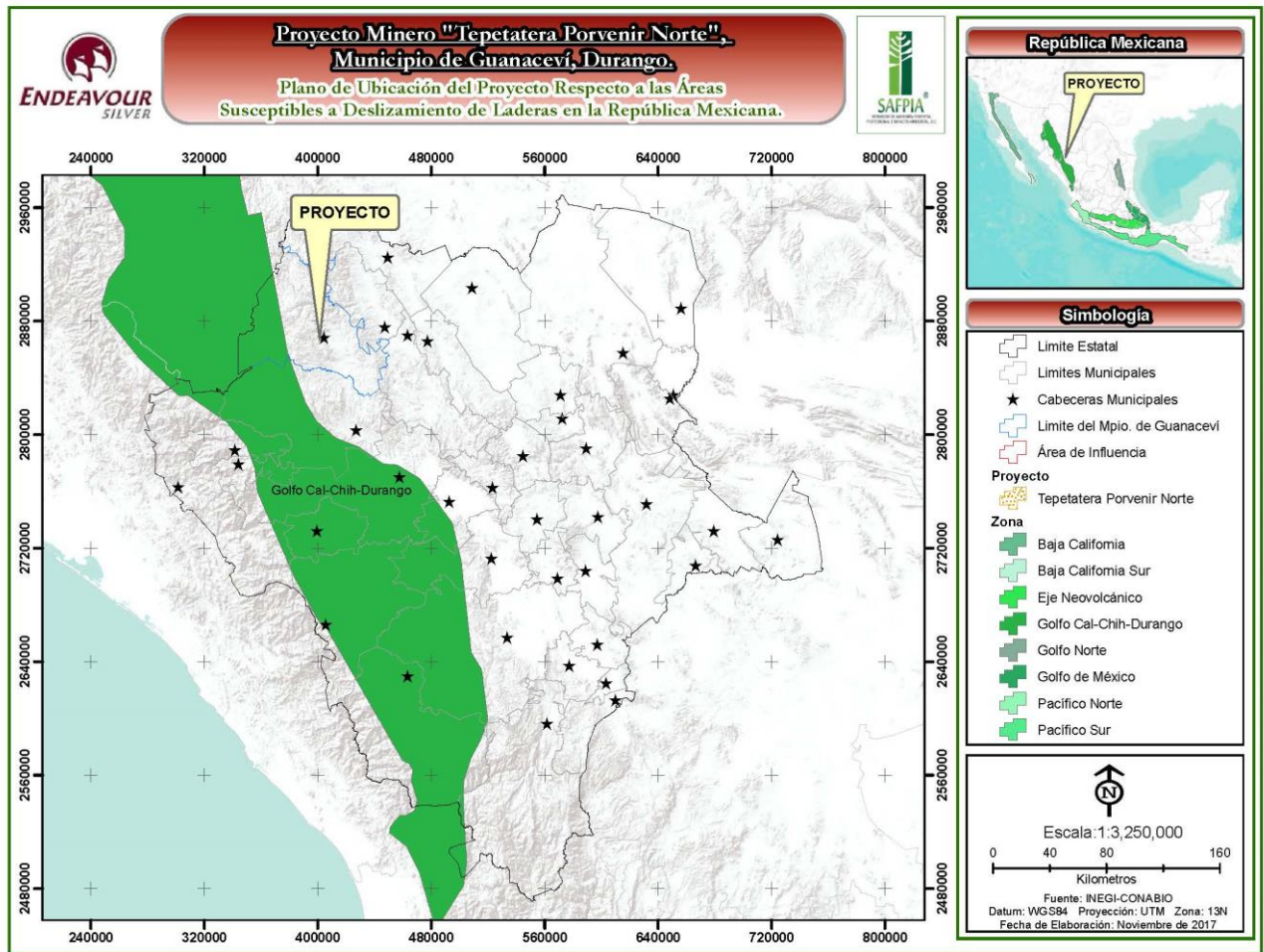
Figura IV-13. Ubicación del proyecto respecto a las Áreas Susceptibles a Deslizamiento de Laderas en la República Mexicana.
