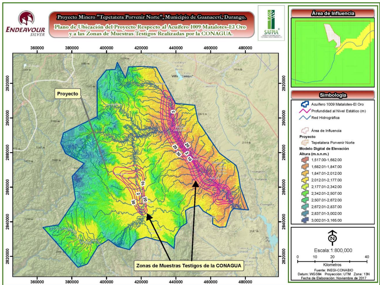
Figura IV-16. Ubicación del proyecto dentro del Acuífero 1009 Matalotes-El Oro.
