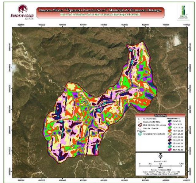
Figura IV-11. Pendiente de la SA.
