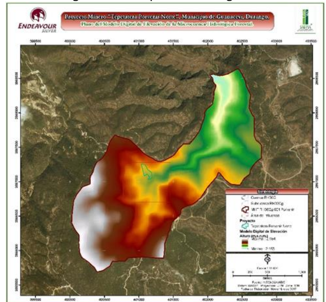
Figura IV-9. Modelo digital de elevación.
