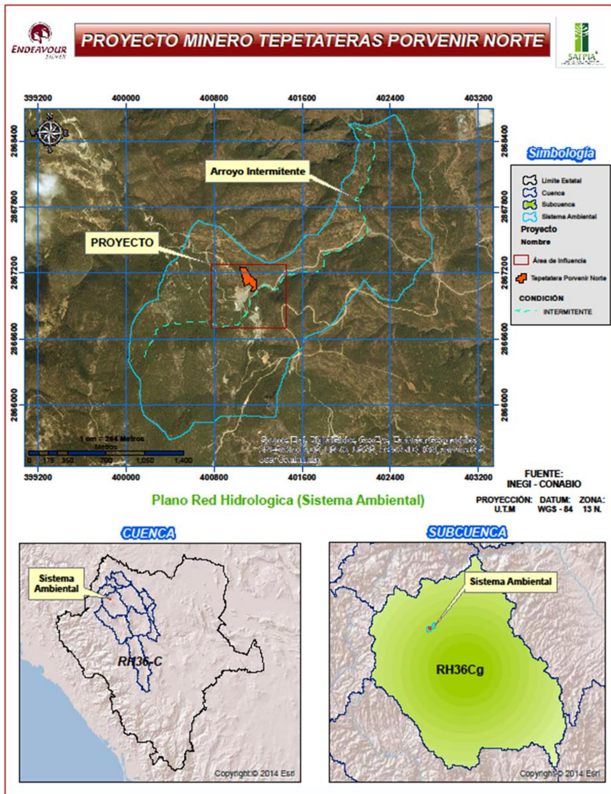
Figura IV-15. Ubicación del SA, AI y AP en el sistema hidrológico.
