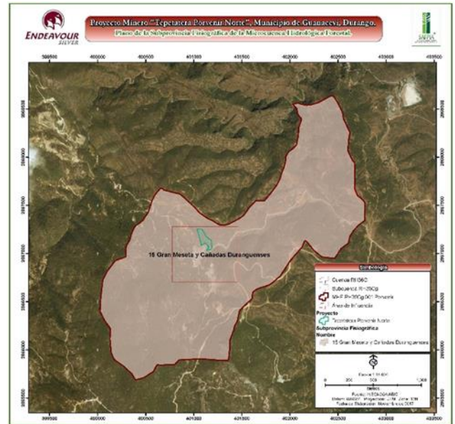
Figura IV-7. Subprovincia fisiográfica.
