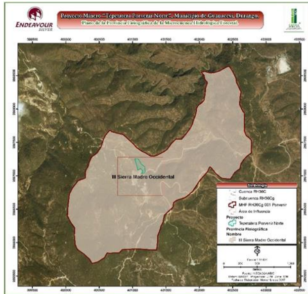
Figura IV-6. Provincia fisiográfica.
