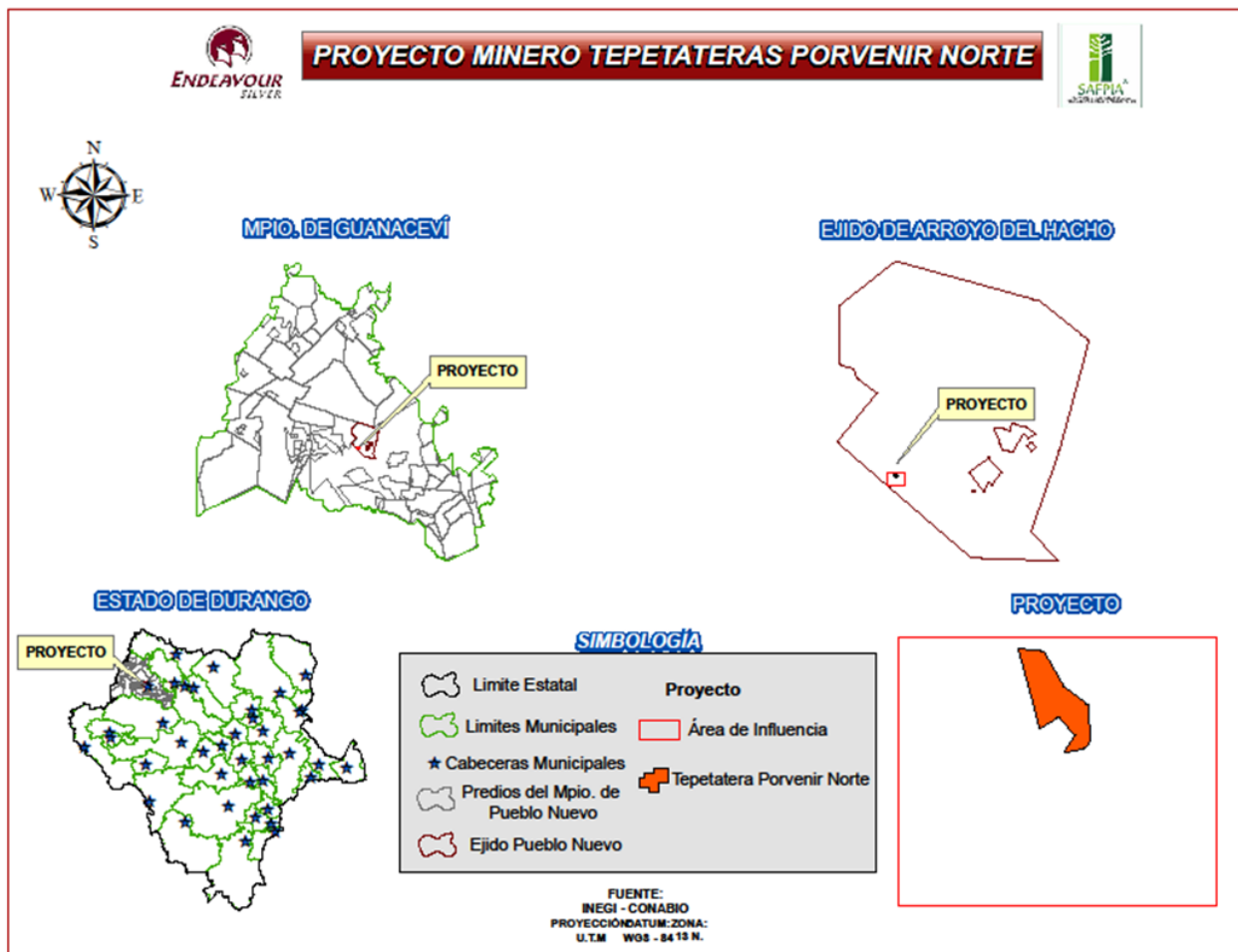
Figura II-6. Ubicación geopolítica del proyecto.
