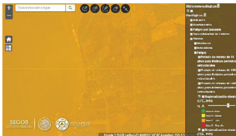
Figura IV.15 Regionalización sísmica.
