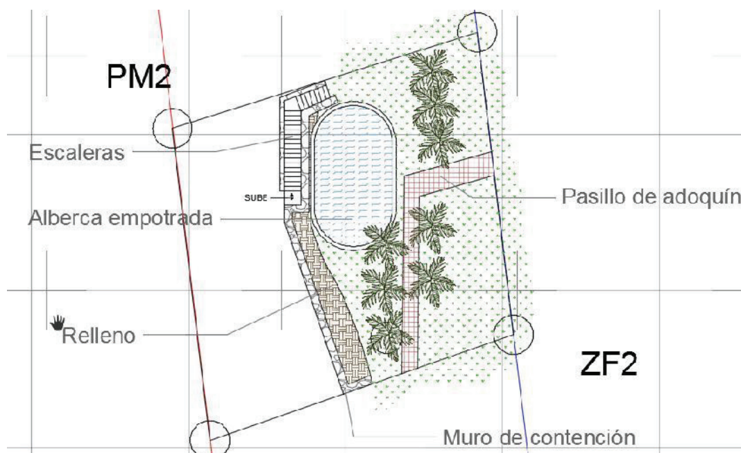
Figura II.4 Diagrama general del "Muro de contención y obras asociadas en Playa La Manzanilla, San Blas, Nayarit"
