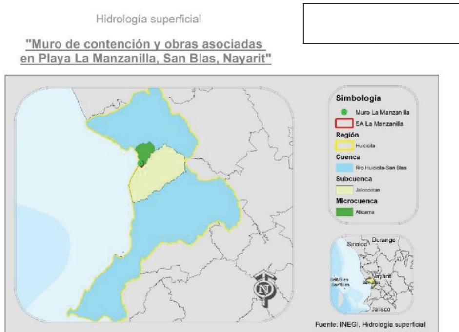
Figura IV.17 Hidrología superficial
