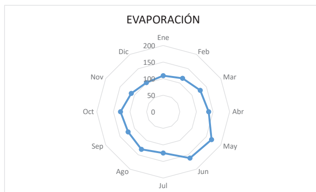
Fig. IV.31 Tasa de el área del proyecto.
