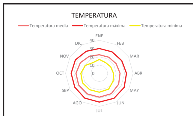
Fig. IV.28 Temperatura máxima, media y mínima mensual del área del proyecto.
