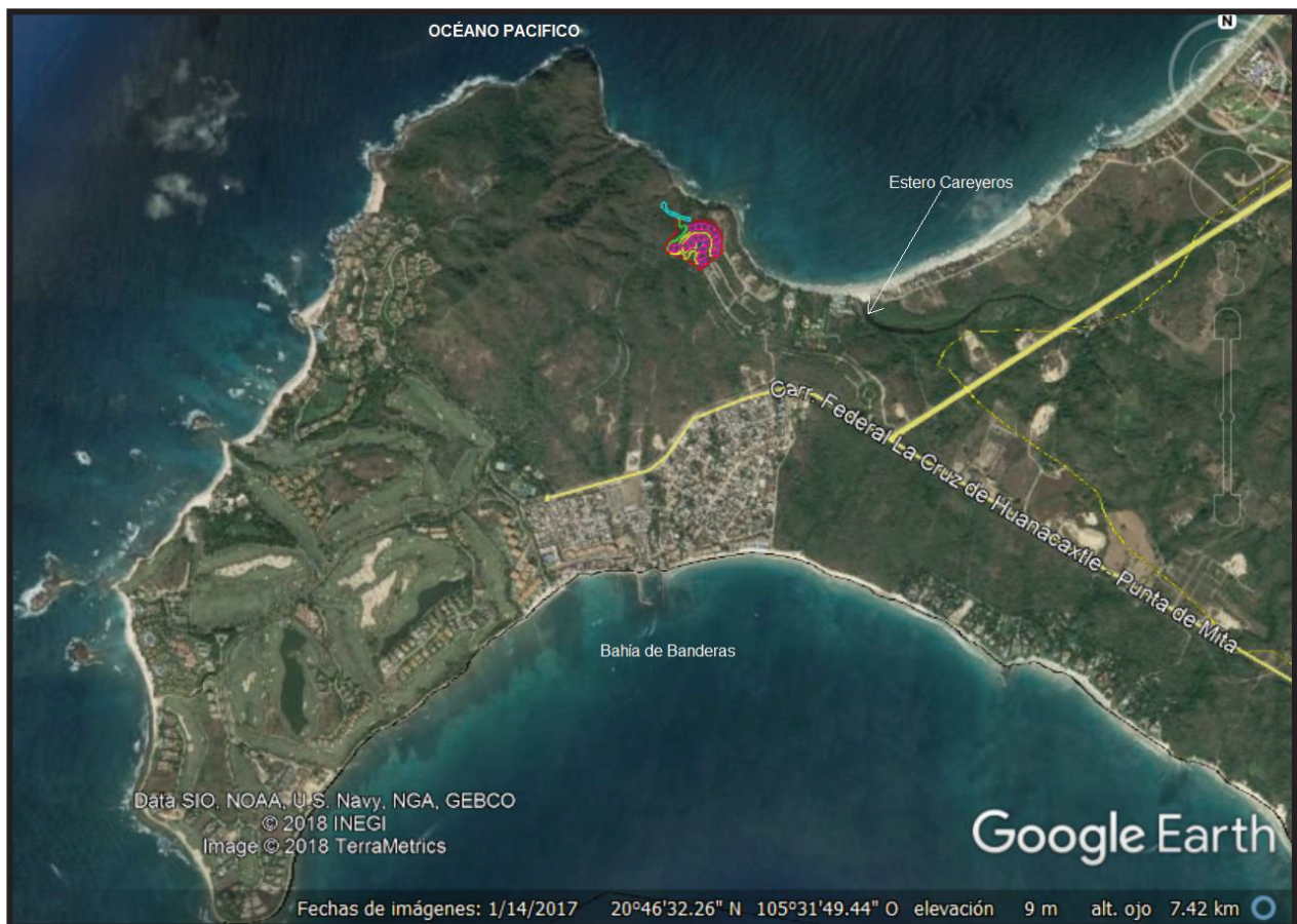
Fig. II.3 Cuerpos de agua cercanos al área del proyecto
