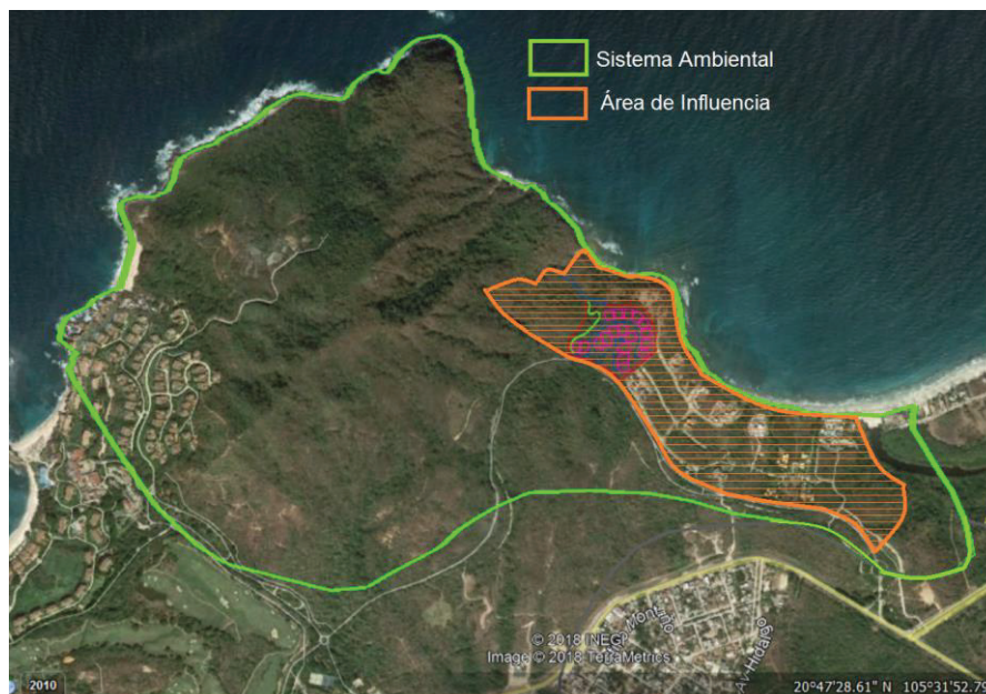
Fig. IV.18 Polígono General del área de influencia determinada para el proyecto.
