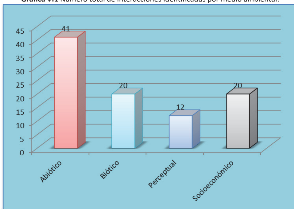
Gráfica V.1 Número total de interacciones identificadas por medio ambiental.
