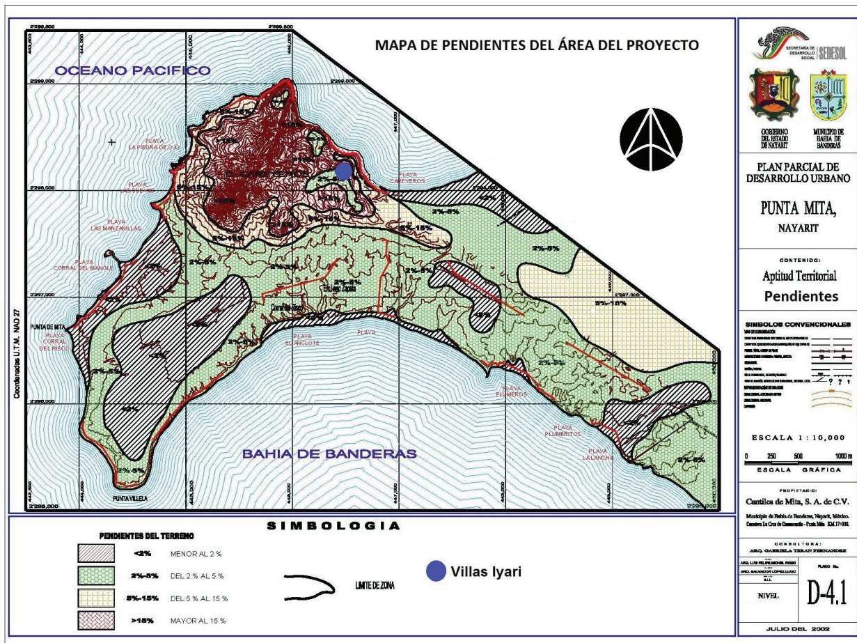
Fig. IV.32 Mapa de pendientes del área del proyecto
