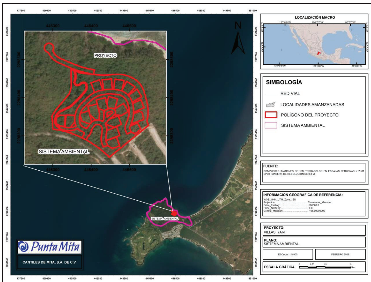
Fig. IV.1 Delimitación del Sistema Ambiental Unidad Ambiental 3E-1 denominada Cerro Careyeros
