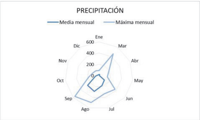
Fig. IV.29 Precipitación mensual en el área del proyecto.
