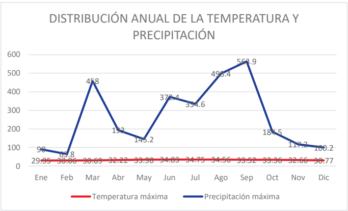
Fig. IV.30 Distribución anual de la temperatura y precipitación mensual en el área del proyecto.
