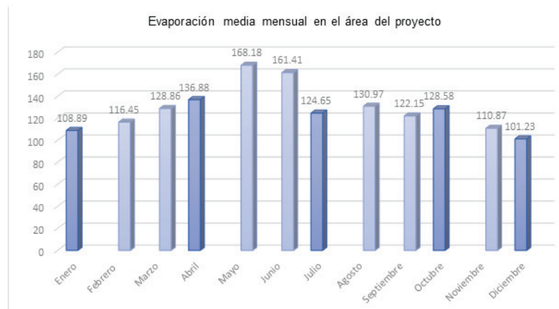
Fig. IV.40 Tasa de evaporación mensual en el área del proyecto.
