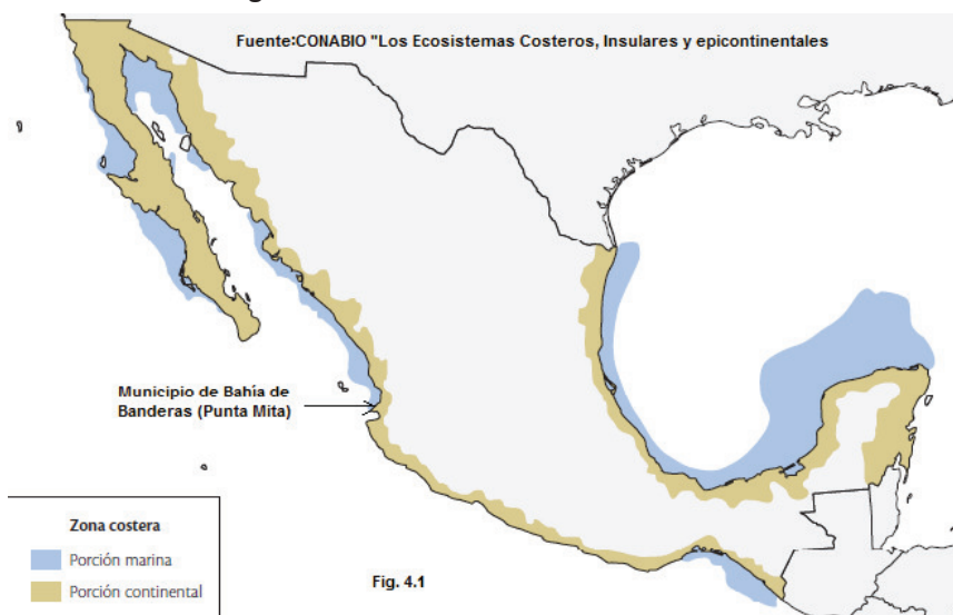
Fig. IV.36 Ecosistemas Costeros de México.
