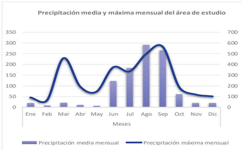
Fig. IV.38 Precipitación media y máxima mensual en el área del proyecto.
