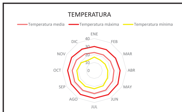
Fig. IV.37 Temperatura máxima, media y mínima mensual del área del proyecto.
