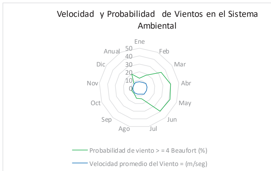
Fig. IV.41 Comportamiento de los vientos en el Sistema Ambiental
