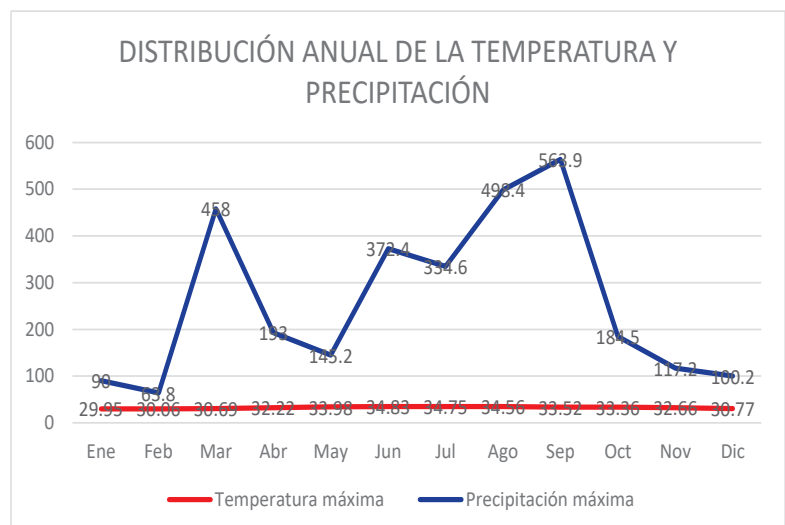
Fig. IV.39 Distribución anual de la temperatura y precipitación en el área del proyecto.
