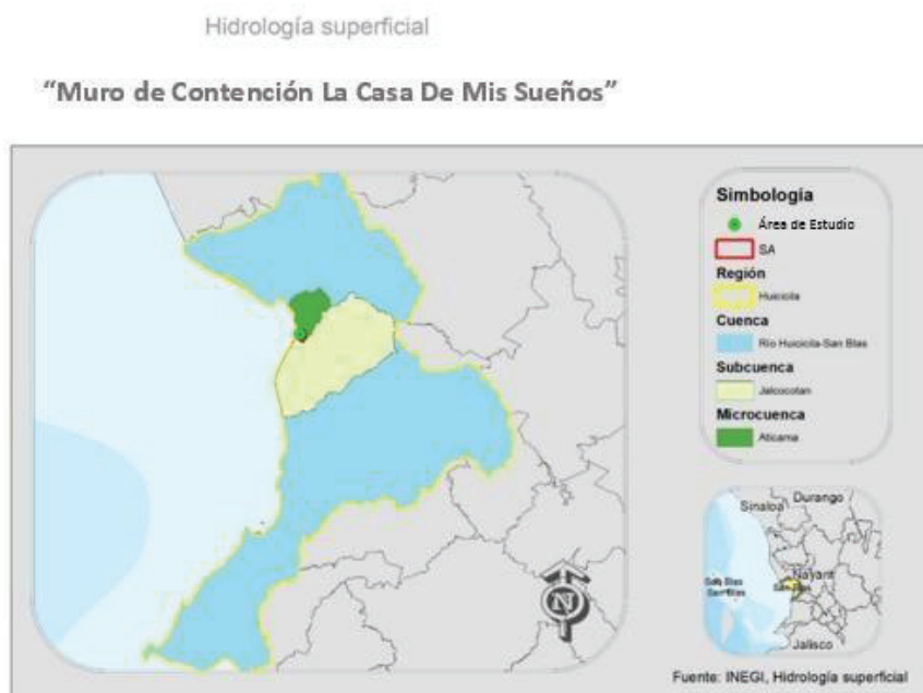
Figura IV.17 Hidrología superficial
