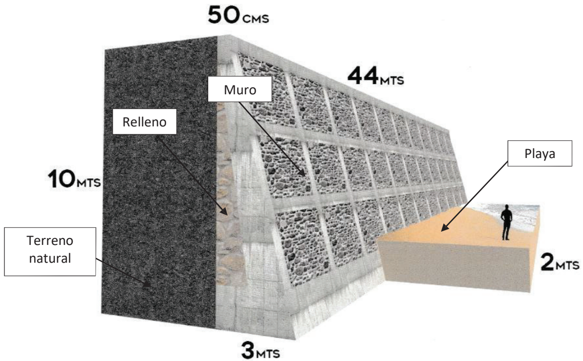
Ilustración 1: Sección del muro de contención.
