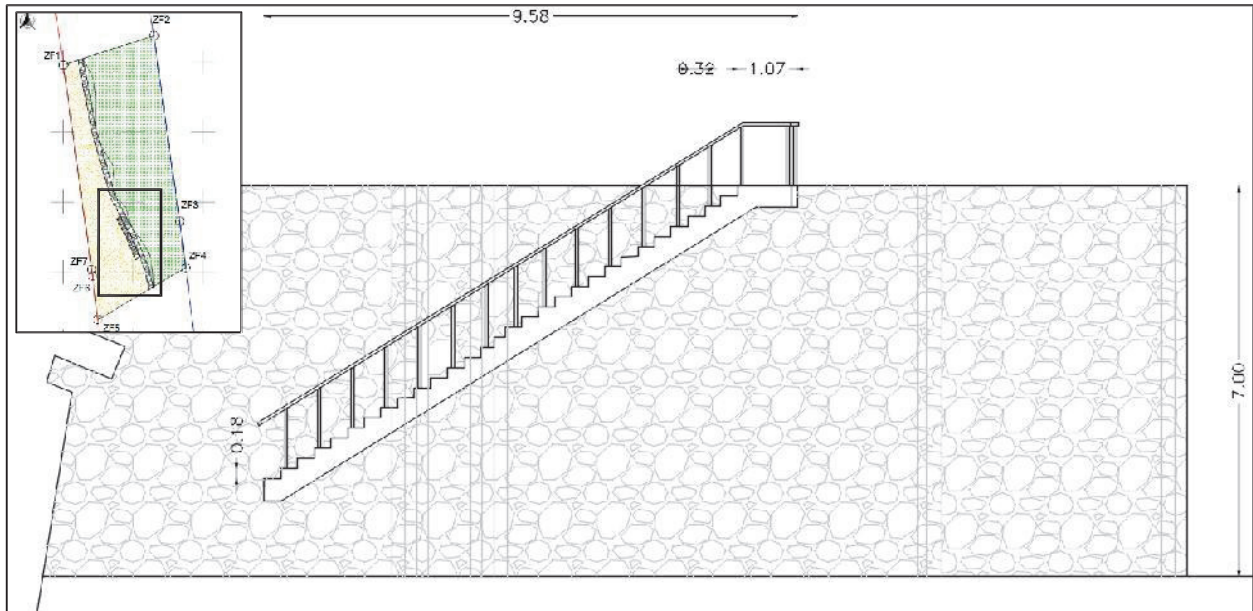
Figura II.7. Tipo de escalera
