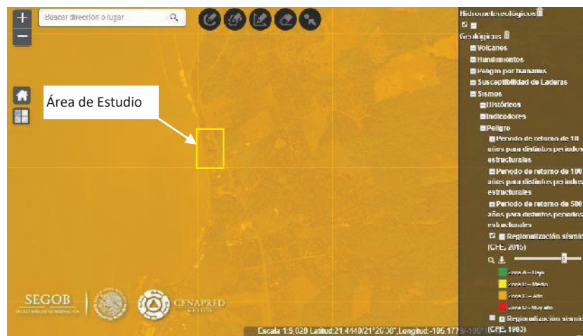
Figura IV.15 Regionalización sísmica.
