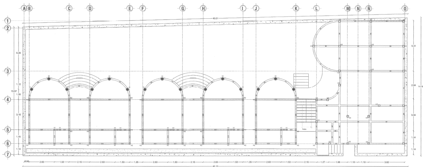
Figura 7 Planta estructural del proyecto
