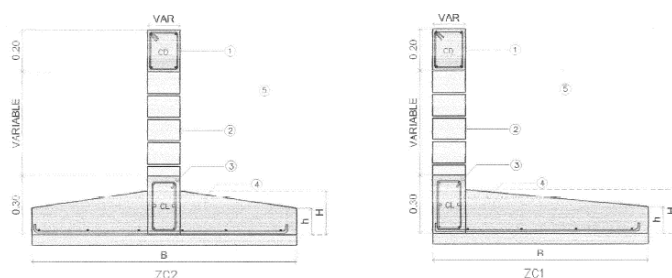
Figura 3 Cimentaciones que serán utilizadas en el proyecto
