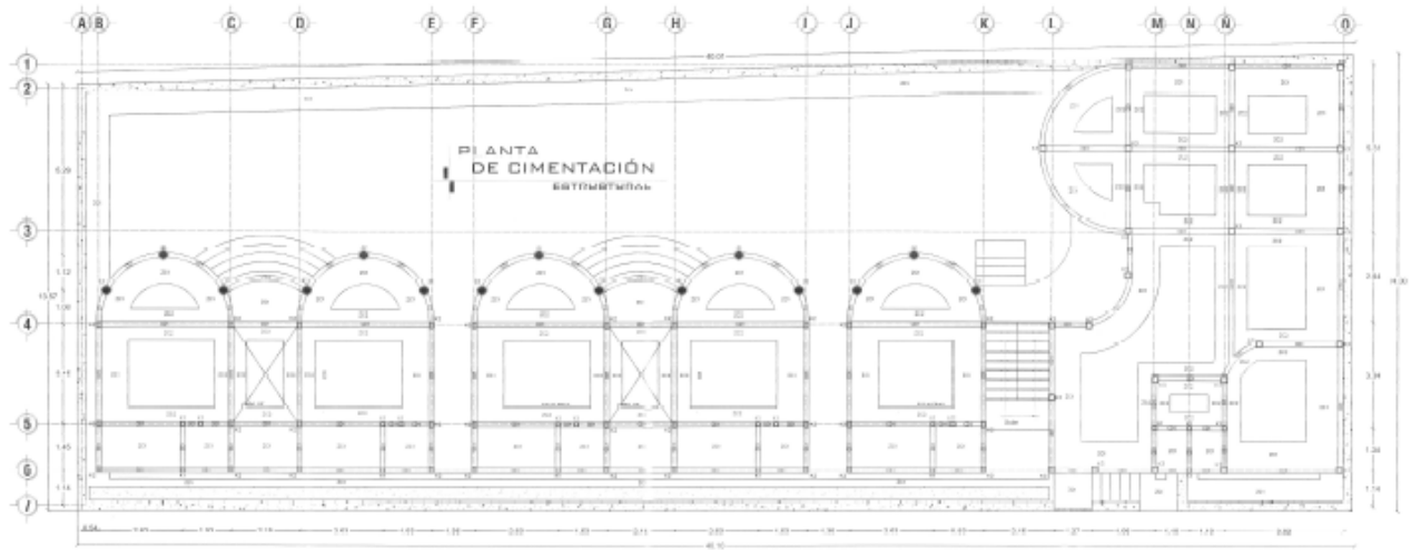
Figura 4 Planta de cimentación del proyecto
