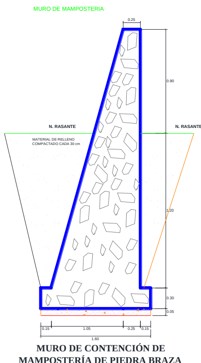
Figura 8 Muro de contención perimetral
