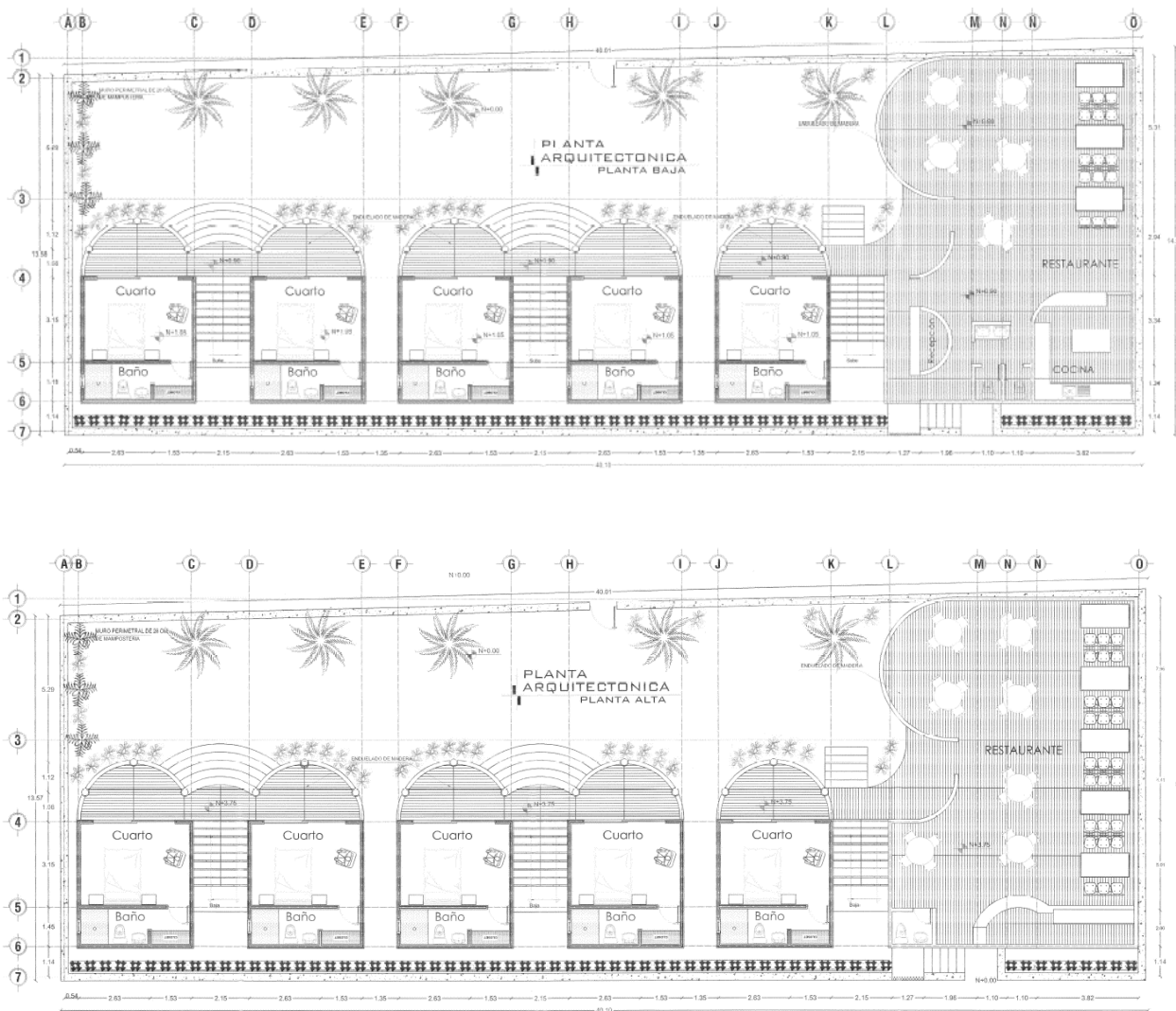
Figura 2 Plantas arquitectónicas planta baja y primer nivel
