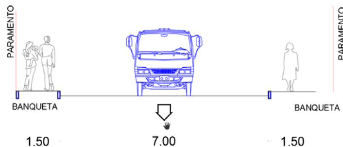
Figura II.6. Corte de la vialidad tipo C-C' que se habrá de implementar.
