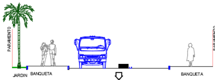
Figura II.4. Corte de la vialidad tipo A-A' que se implementará.
