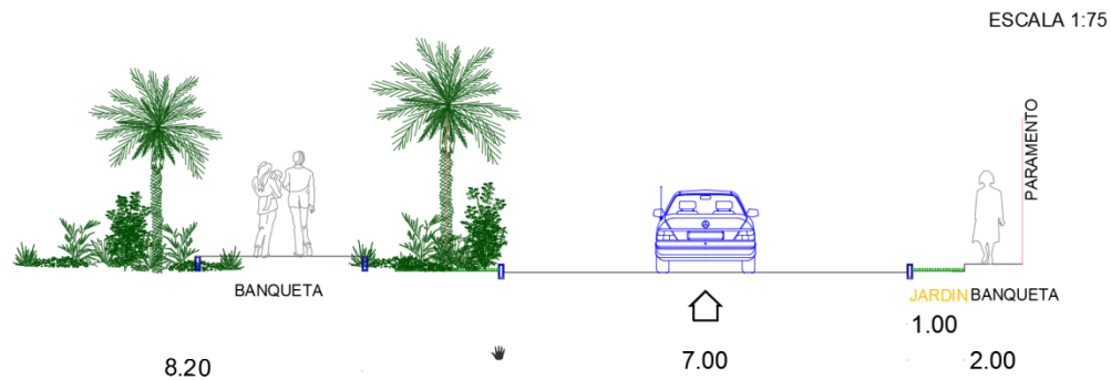
Figura II.5. Corte de la vialidad tipo B-B' que se implementará.
