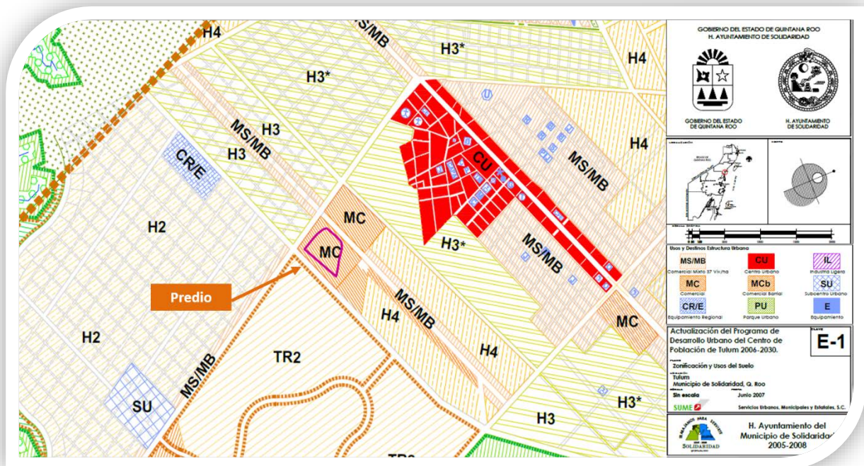
Figura III.4. Plano zonificación y usos del sitio E-1.
