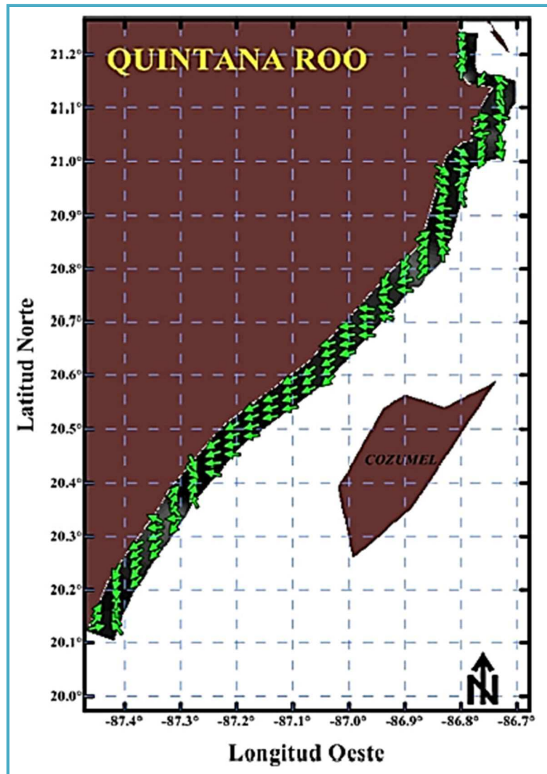
Figura IV_ 12. Dirección de transporte de sedimentos.
