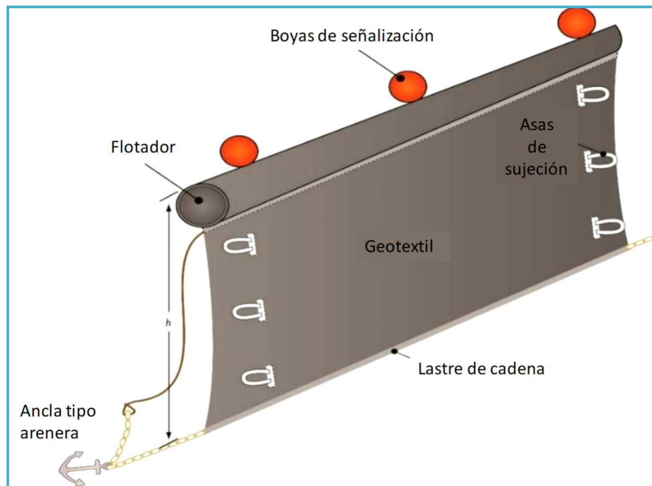
Figura II_ 34. Diseño de la malla de geotextil antidispersión.
