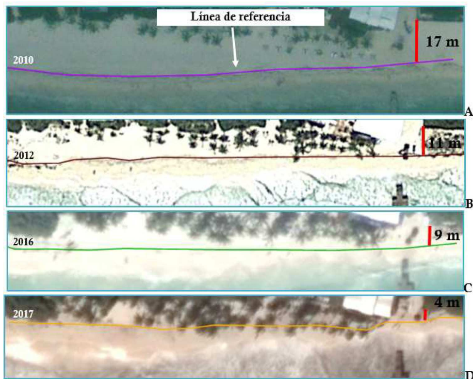
Figura II_ 7. Línea de costa de la zona del proyecto: A) 2010, B) 2012, C) 2016 y D) 2017 durante evento hidrometeorológico.
