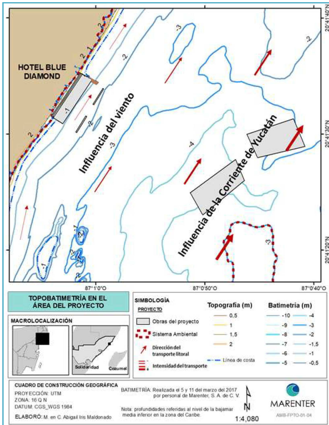
Figura IV_ 14. Análisis del transporte litoral en la zona del proyecto.
