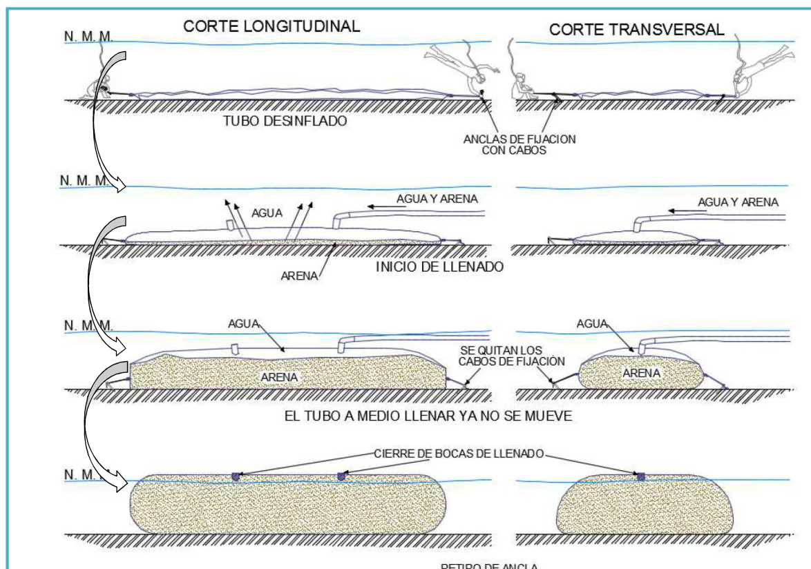
Figura II_ 25. Proceso típico de desplante de un rompeolas.
