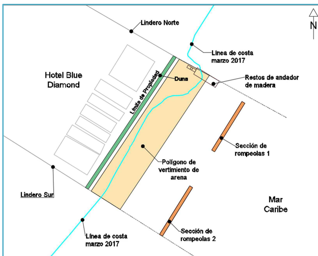
Figura VII_1. Plano general de obras del proyecto.
