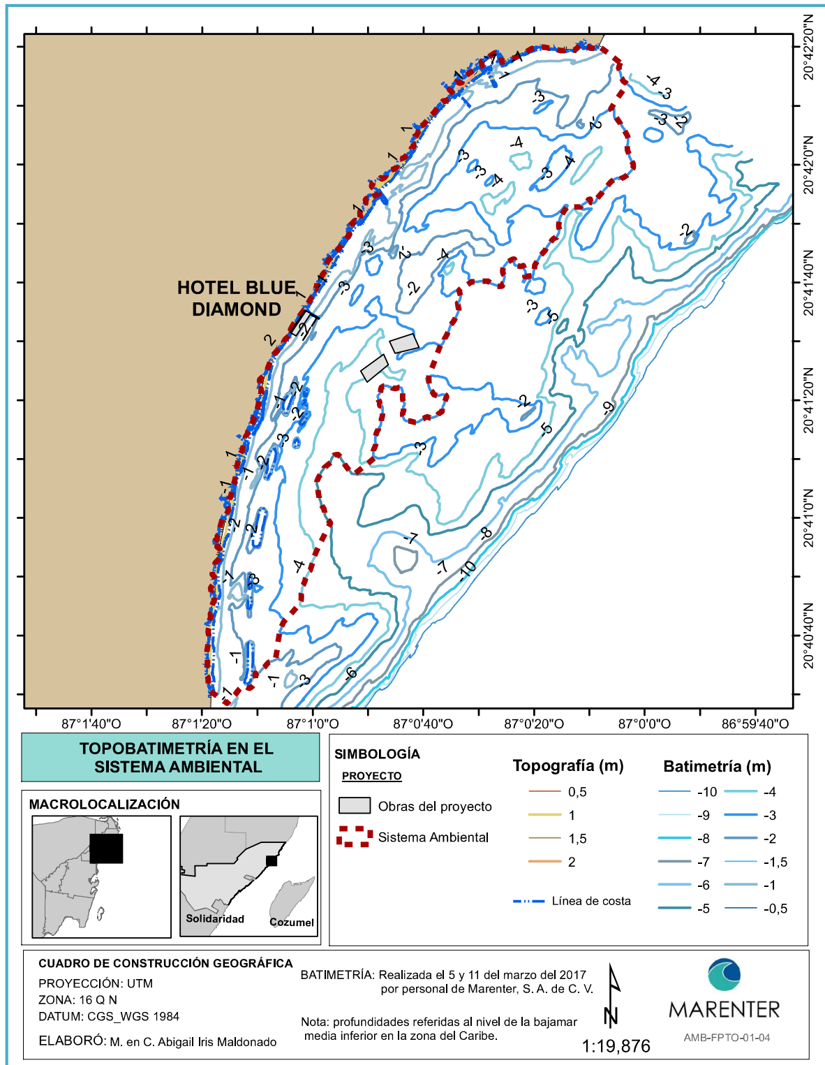
Figura IV_ 20. Topobatimetría en Sistema Ambiental.
