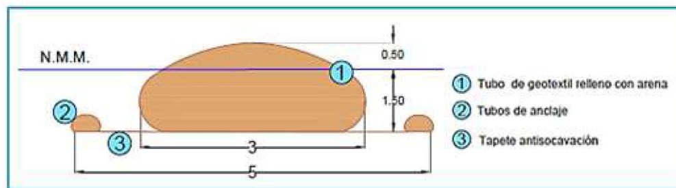
Figura II_ 5. Corte transversal de rompeolas
