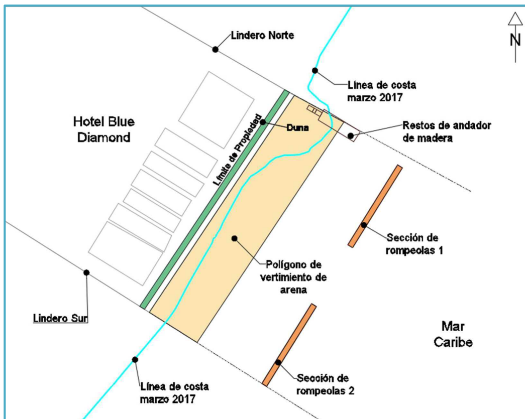
Figura II_ 4. Plano general de obras del proyecto.
