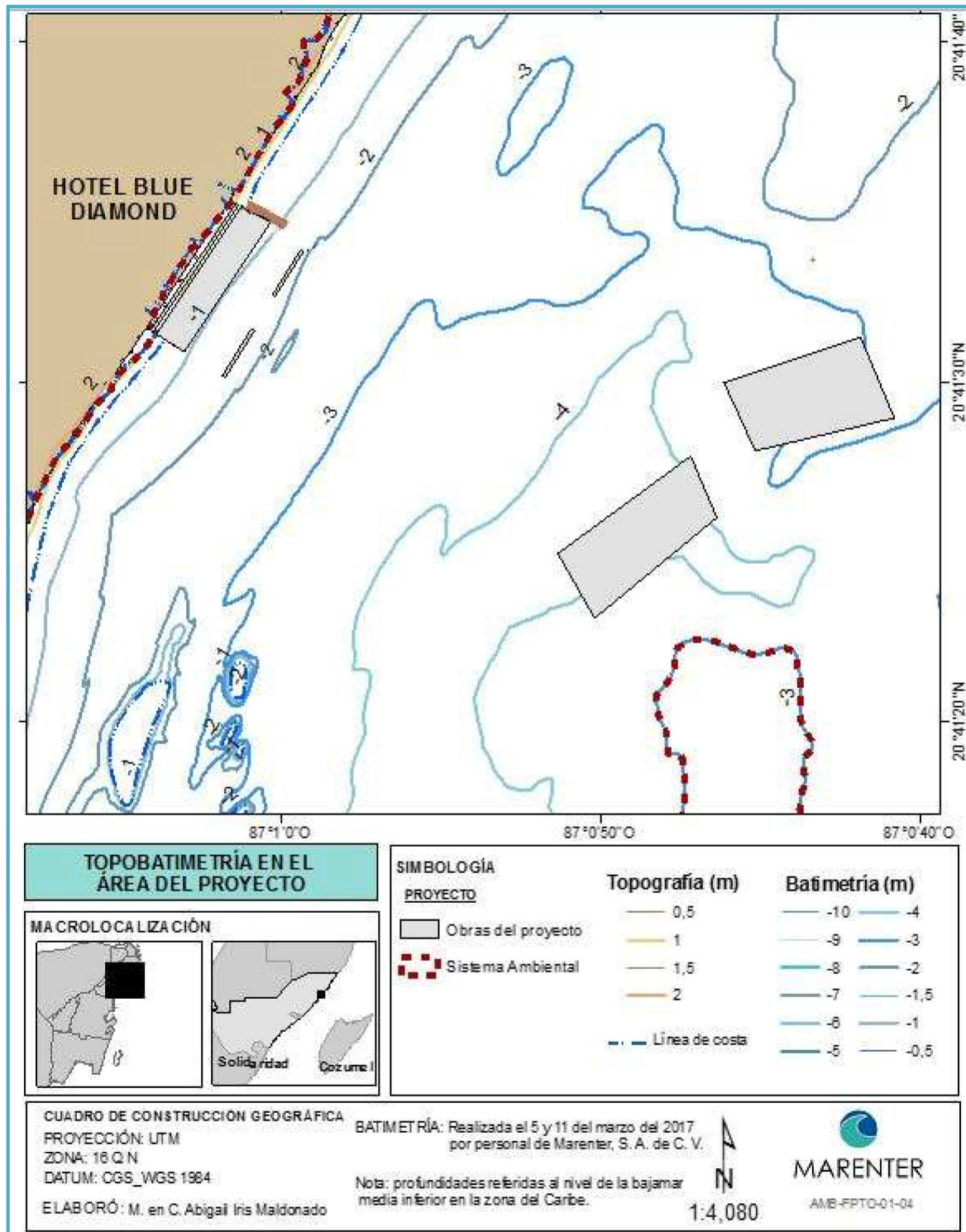
Figura IV_ 21. Topobatimetría en el área del proyecto.
