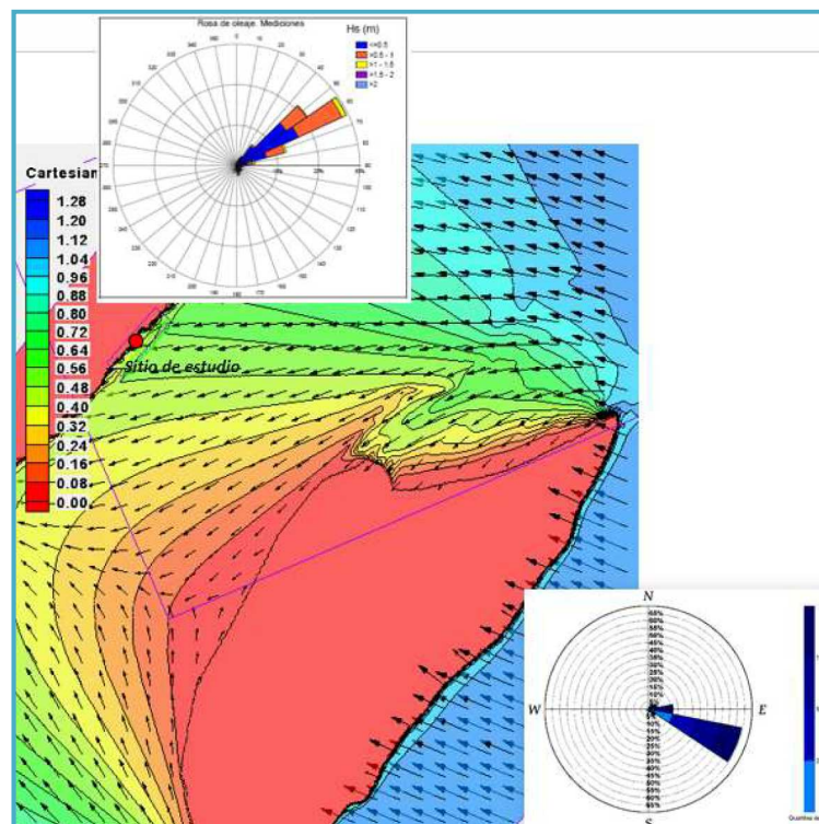
Figura IV_ 15. Oleaje del Este-Sureste. A) Forma en que se difracta el oleaje antes de llegar a la zona de estudio.
