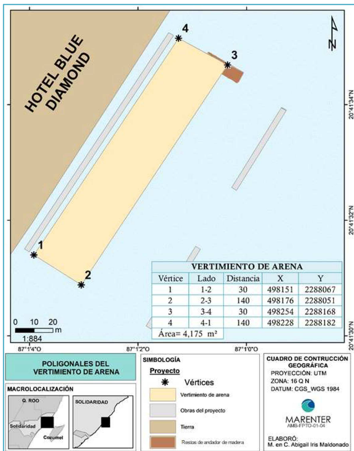
Figura II_ 10. Mapa con el cuadro de construcción en coordenadas UTM de la zona de vertimiento de arena.
