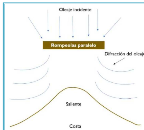
Figura II_ 20. Efecto ante la presencia de un rompeolas paralelo.
