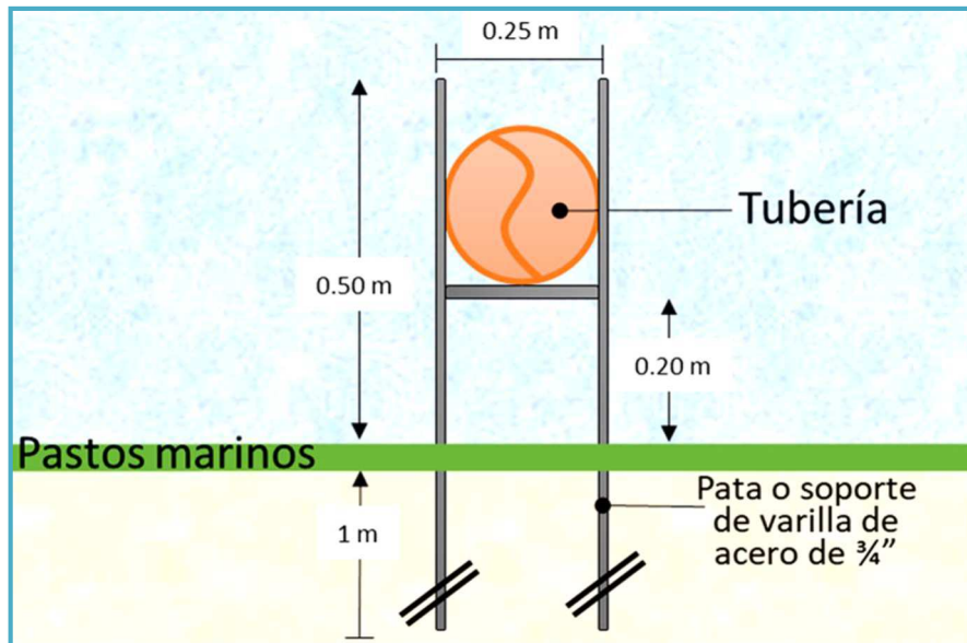
Figura II_ 32. Tuberías y mangueras con lastre de proyectos similares para zonas con pastos marinos.
