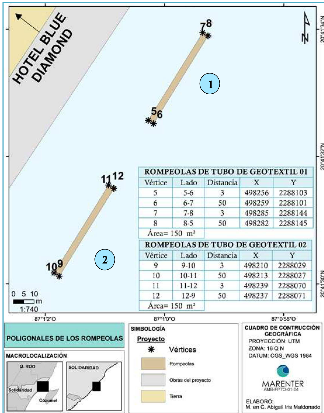
Figura II_ 8. Mapa con el cuadro de construcción en coordenadas UTM de las secciones de rompeolas 1 y 2.
