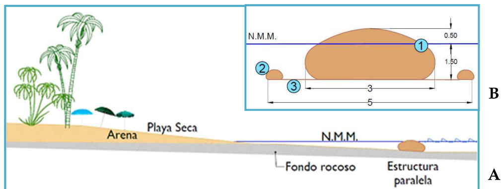
Figura II_ 18. Diseño de rompeolas. A) Corte longitudinal B) Corte transversal.
