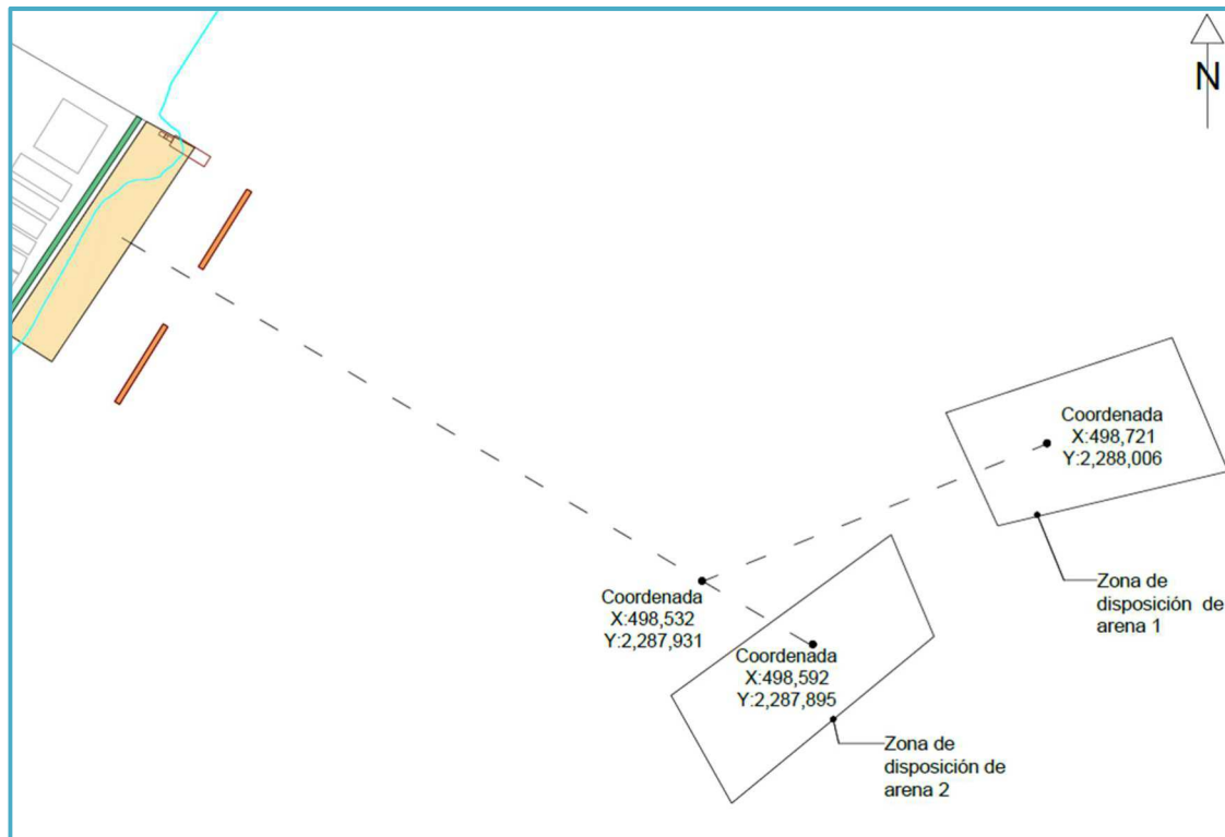
Figura II_ 30. Trayectoria de la tubería.
