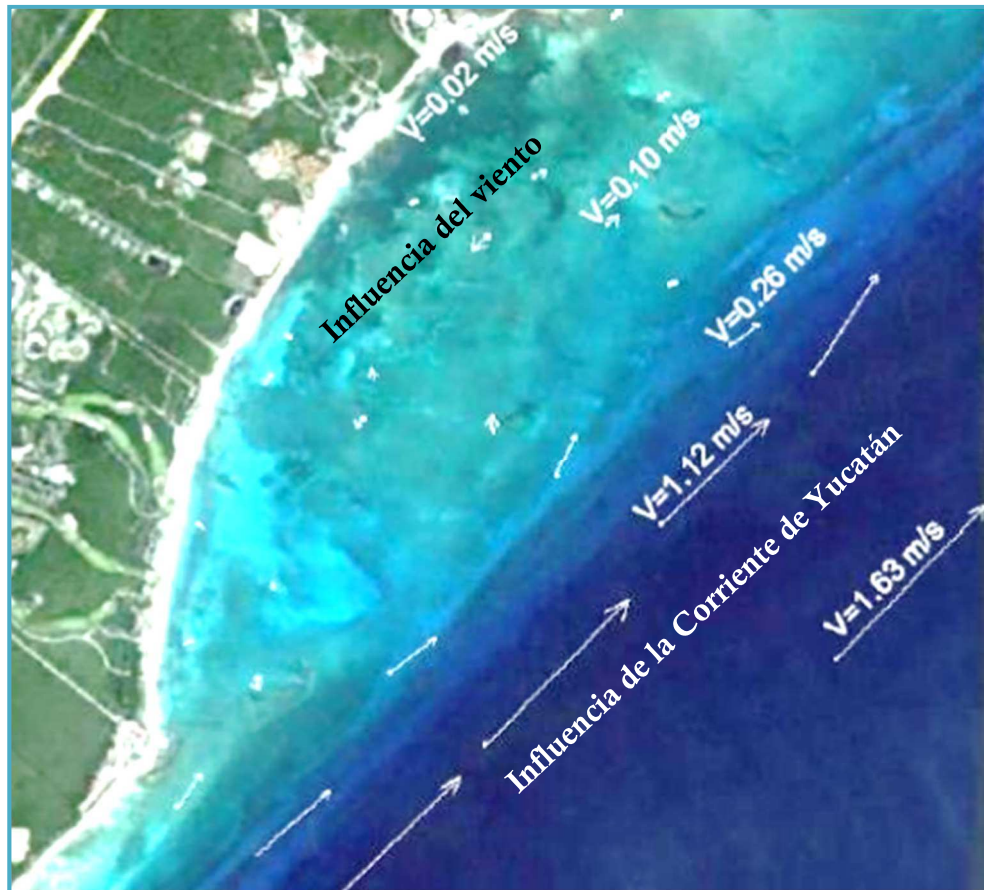
Figura IV_ 13. Sistema de transporte litoral en el SA (tomada de la MIA – 23QR2014T0007).
