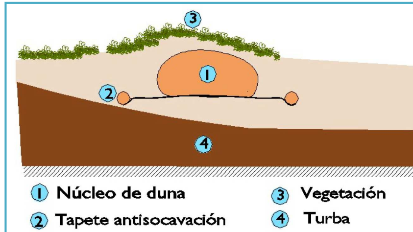
Figura II_ 26. Detalle de los elementos que conforman la duna.
