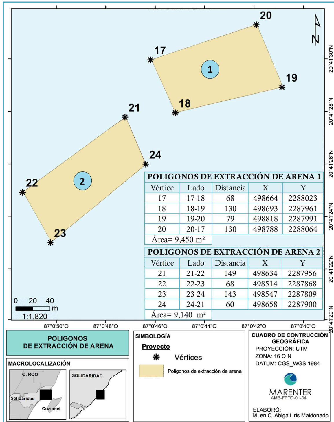
Figura II_ 11. Mapa con el cuadro de construcción en coordenadas UTM de las zonas de disposición de arena.
