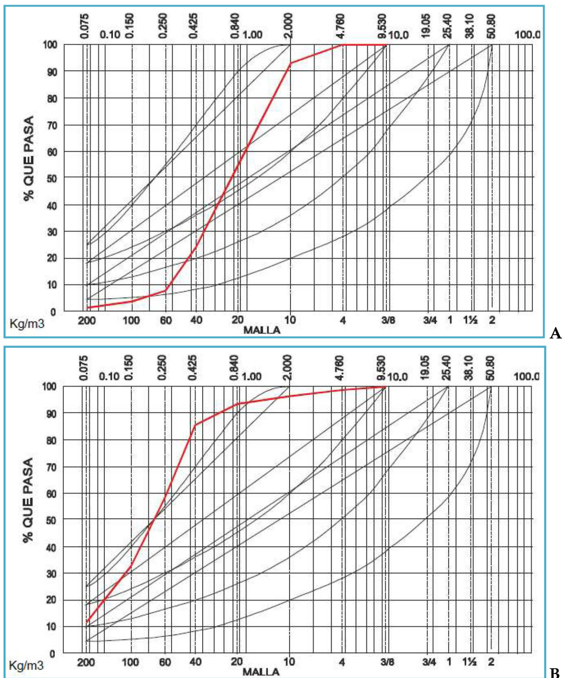
Figura IV_25. Análisis de la granulometría de las muestras de arena en la playa. A) Polígono 1, B) Polígono 2.
