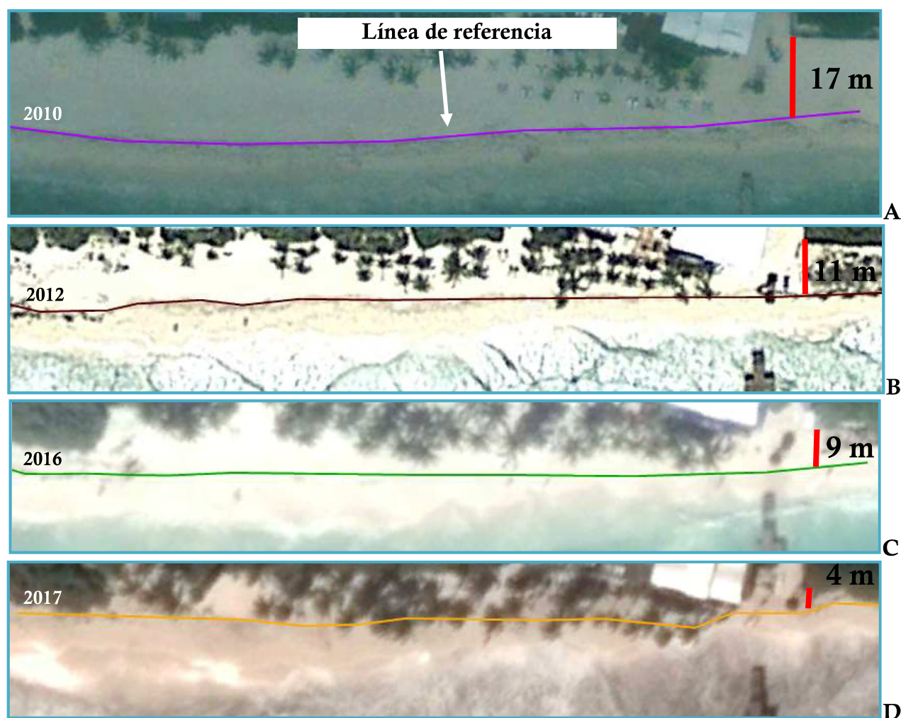
Figura VII_ 3. Línea de costa de la zona del proyecto, A) 2010 y C) 2016 en condiciones actuales. B) 2012 y D) 2017 durante evento hidrometeorológico.
