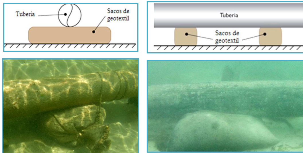
Figura II_ 31. Tuberías y mangueras con lastre de proyectos similares para zonas libres de pastos marinos.
