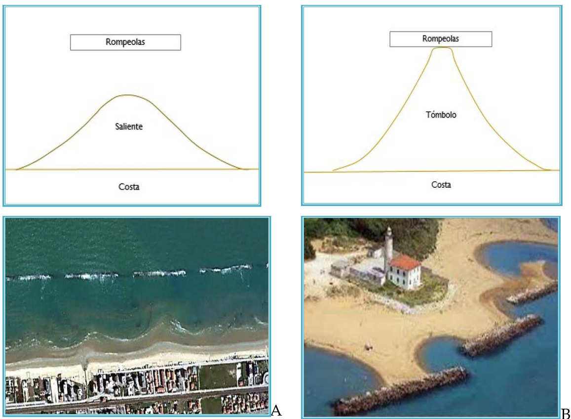
Figura II_ 22. Ejemplos de respuesta de playa con rompeolas paralelos (A Salientes, B tómbolos).
