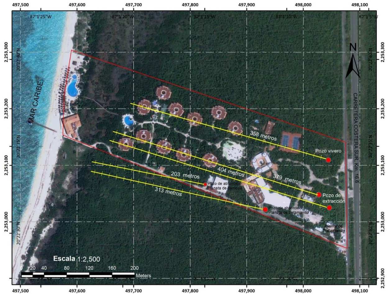
Figura 18. Localización de la planta de ósmosis y de los pozos de extracción y de absorción de agua, con relación al humedal que se ubica en las inmediaciones de la propiedad.
