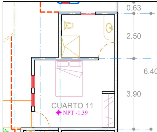
Figura 2.14. Cuartos 11 y 12 planta baja.
