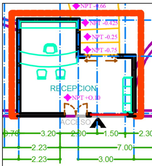
Figura 2.6. Recepción.
