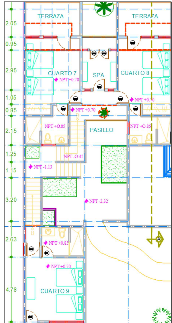
Figura 2.13. Planta alta de los cuartos 5-8.
