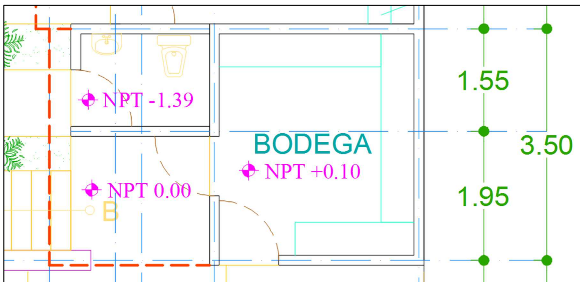
Figura 2.15. Bodega y baños mixtos.
