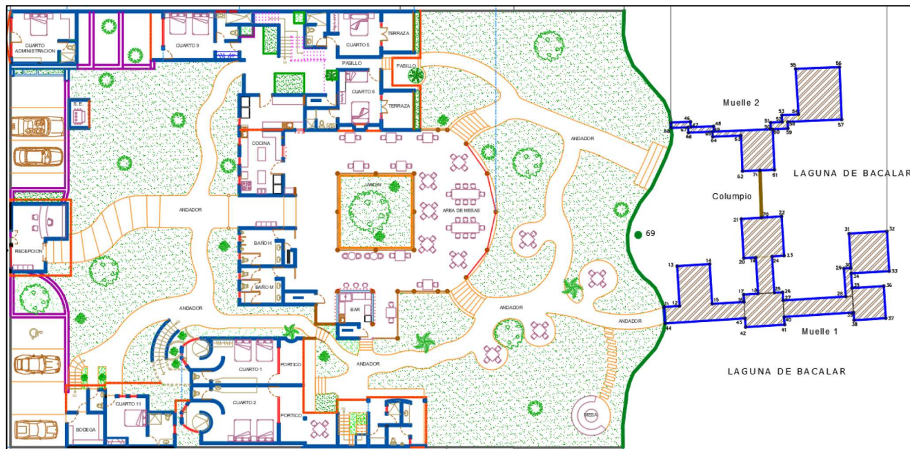
Figura 2.5. Plano de conjunto del proyecto.
