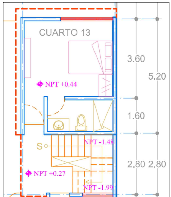
Figura 2.16. Planta baja del edificio de las regaderas. Figura 2.17. Planta alta del edificio del cuarto 13.
