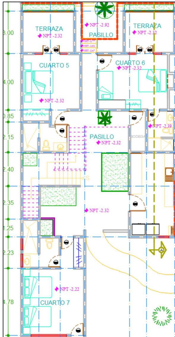
Figura 2.12. Planta baja de los cuartos 5-8.
