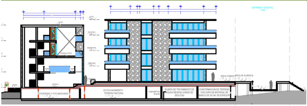
Sección longitudinal de los edificios. El sótano se desplanta a partir de la cota +1.00 que es la que continúa en el nivel del camino, a partir de ahí la losa de piso se desplanta a los +1.92 y +2.38 metros, es decir entre 2.92 y 3.38 ml por encima de la cota del nivel medio del mar. La altura máxima de las edificaciones es de 12.00 ml o 4 niveles a partir de la losa de piso.
