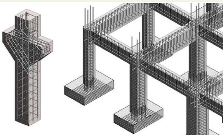
Diagrama de armado de losa de piso en un sistema de cimentación a base de zapatas aisladas:
