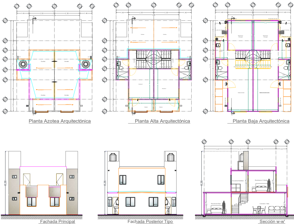
Ilustración 5.-prototipo de vivienda Koh de forma horizontal
