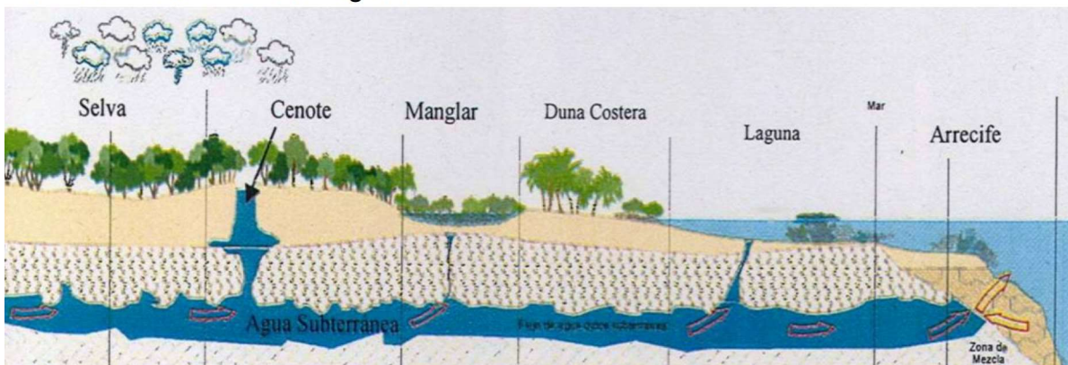
Ilustración 20.- Esquema de los escurrimientos subterráneos de la Península de Yucatán.
