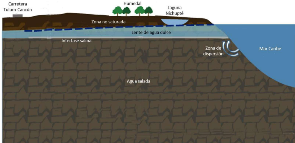
Ilustración 21.- Modelo conceptual hidrogeológico local
