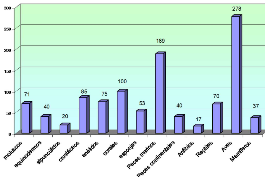
Ilustración 33.- Riqueza de especies de cada uno de los grupos de fauna silvestre reportados para el municipio Benito Juárez. POEL 2013
