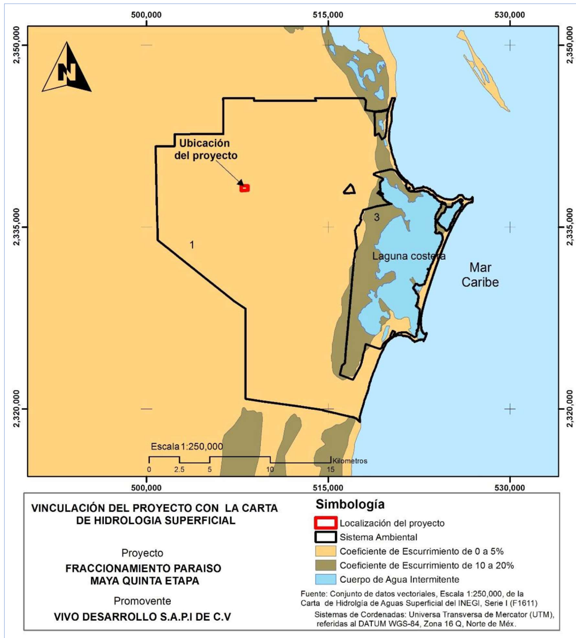
Ilustración 23.- Distribución espacial de las principales características y condiciones del acuífero subterráneo del SA.
