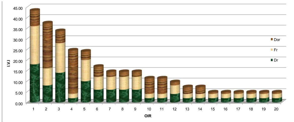
Ilustración 32.- Índice de Valor de Importancia (I.V.I.) para el estrato herbáceo. Dr-Densidad relativa, Fr-Frecuencia relativa y Dor- Cobertura relativa.
