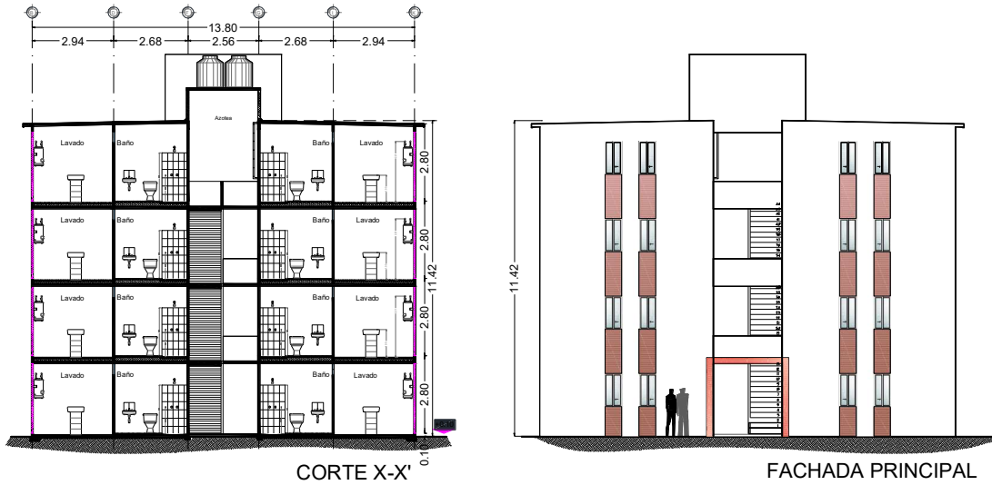
Ilustración 3.- Prototipo Buran, vivienda vertical
