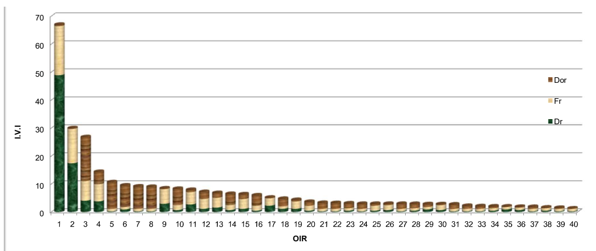
Ilustración 31.- Índice de Valor de Importancia (I.V.I.) para el estrato arbustivo. Dr- Densidad relativa, Fr-Frecuencia relativa y Dor Dominancia relativa.
