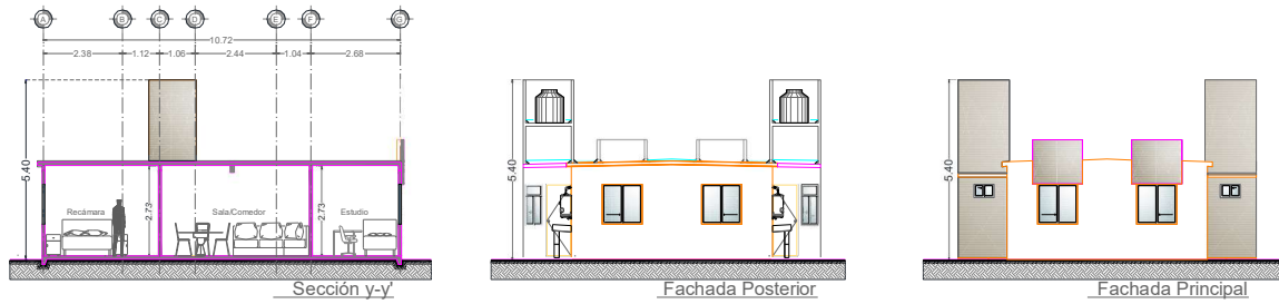
Ilustración 4.- Prototipo de vivienda Kai de forma Horizontal
