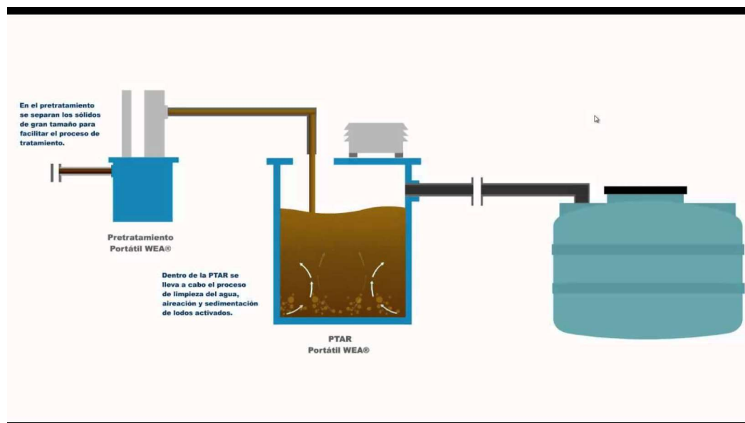
Figura II.4. Diagrama del tratamiento de aguas residuales.
