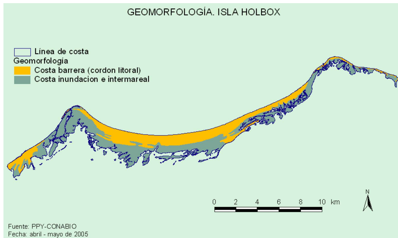
Figura IV.5. Geomorfología de la Isla de Holbox.
