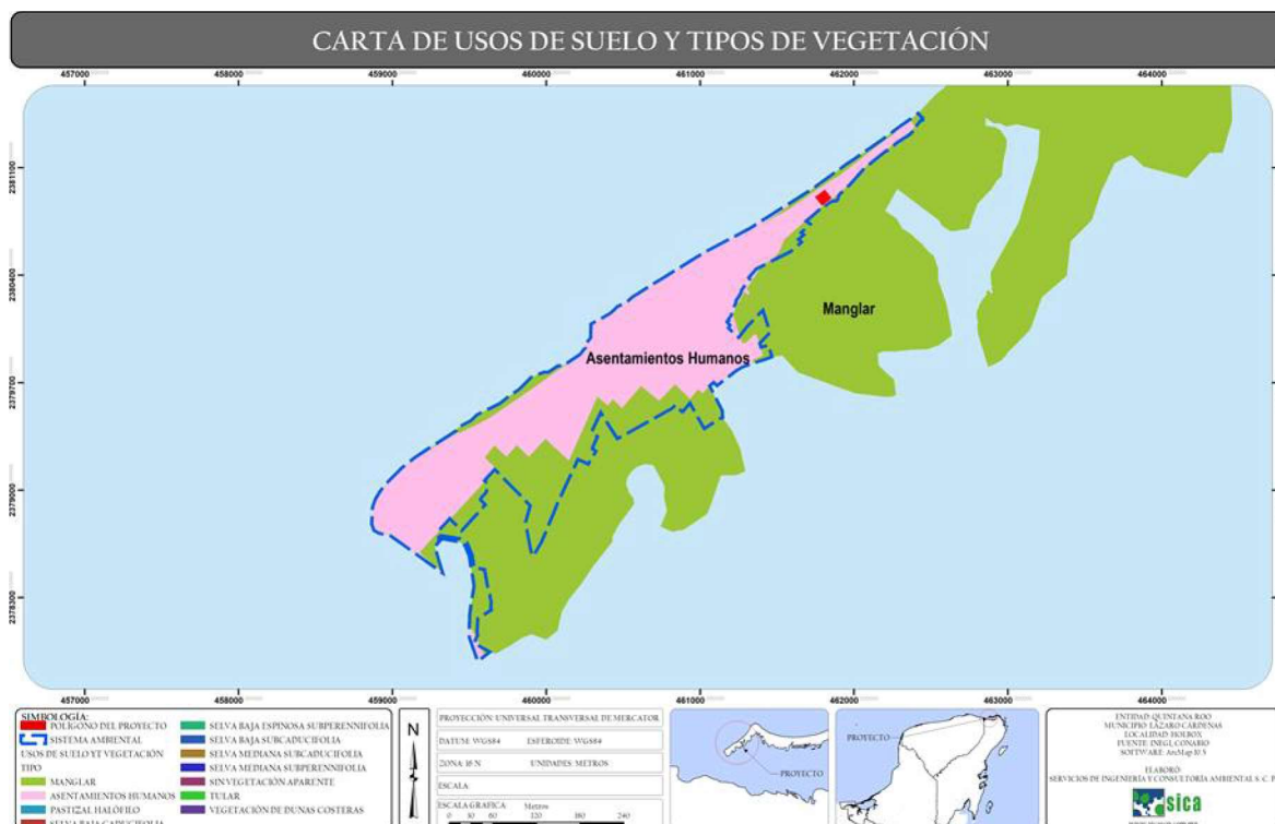
Figura IV.10. Vegetación potencial del área de estudio.
