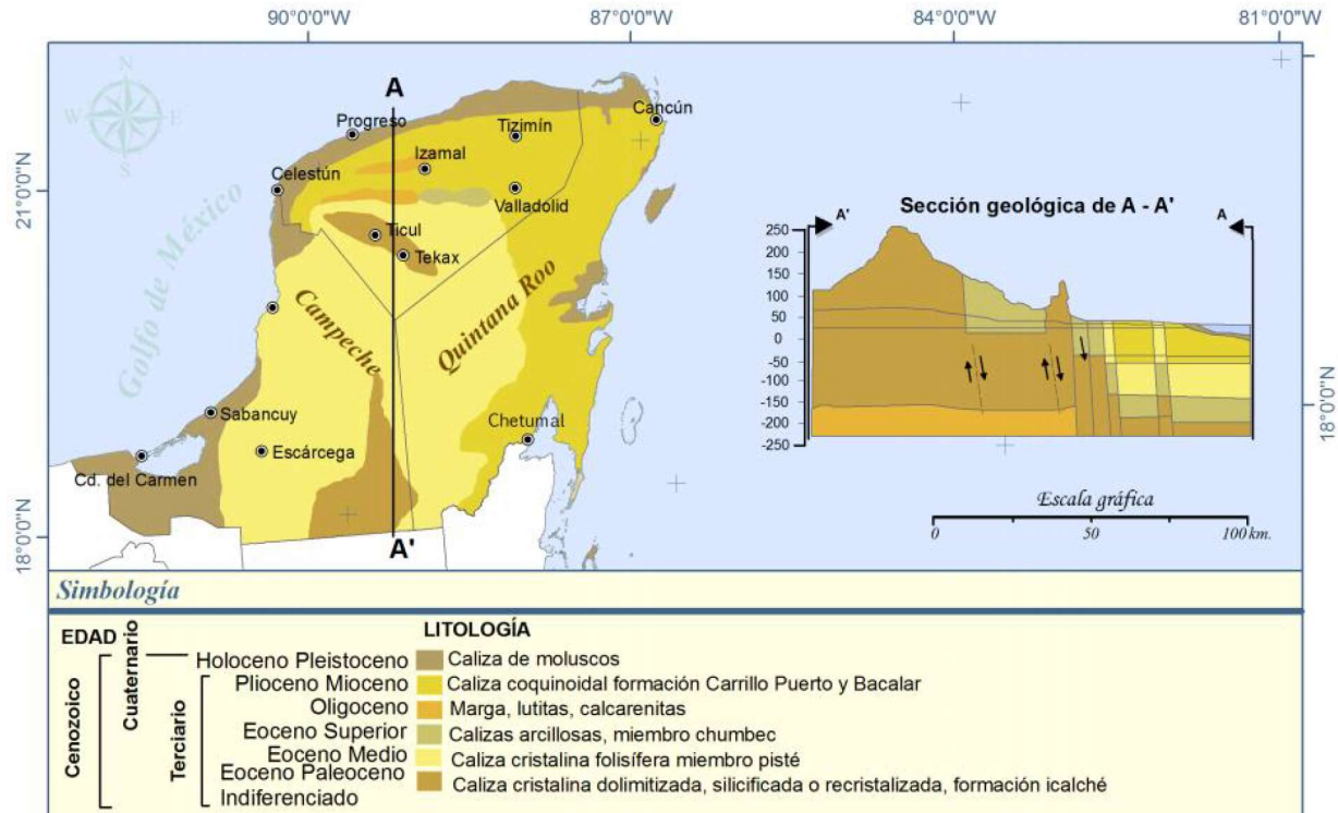
Figura IV.3. Clasificación geológica de la Península de Yucatán.
