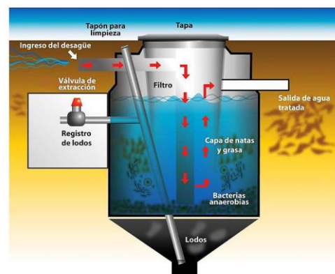
Figura 2.4 Operación del Biodigestor
