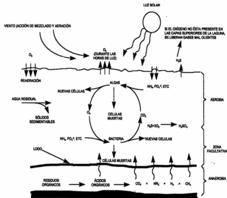
Figura 2.14 Descomposición de materia orgánica.
