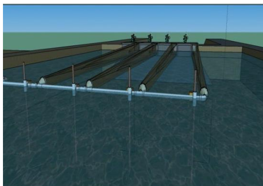
Figura 2.10 Diagrama tubería de exclusión del SEFA.
