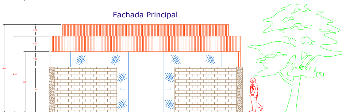
Figura 2.12 Almacén para los residuos sólidos.
