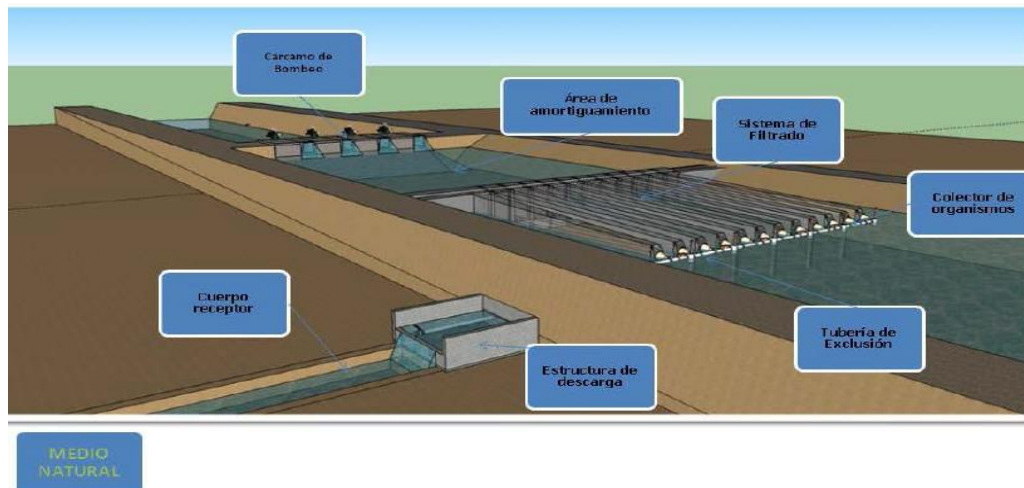
Figura 6.2 Diagrama Operativo del SEFA
