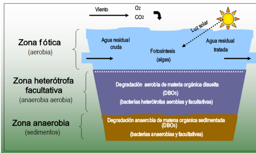
Figura 6.4 Operación de la Laguna de Oxidación
