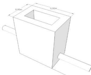
Figura 2.11 Diagrama Registros de recuperación del SEFA.
