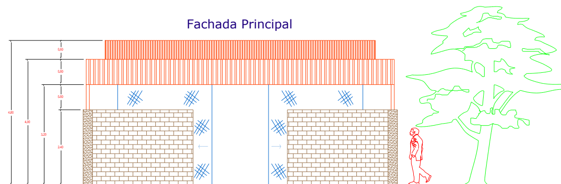
Figura 6.5 Propuesta para el almacen de residuos peligrosos
