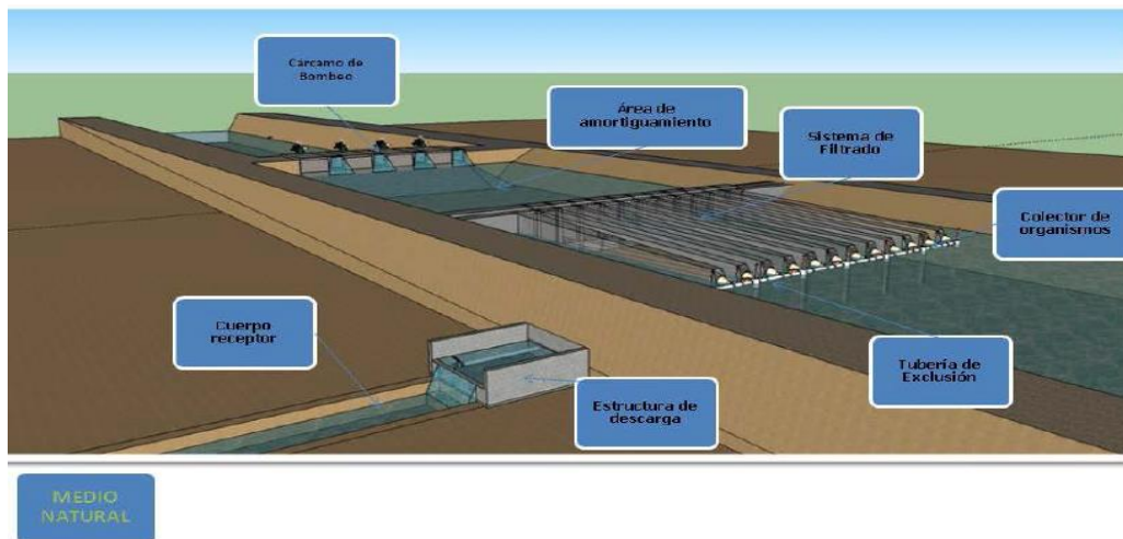
Figura 2.6 Diagrama Operativo del SEFA.
