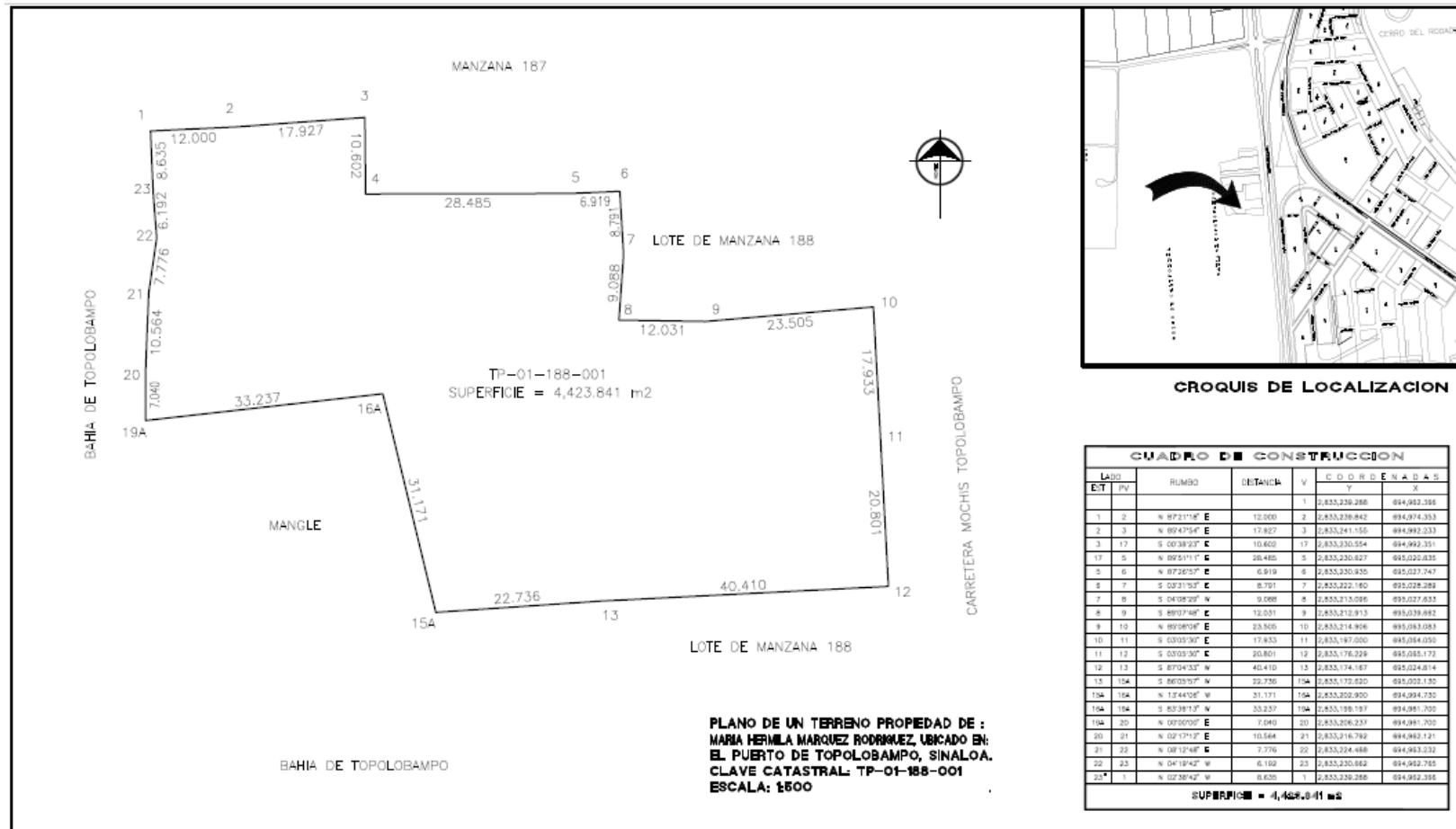
Imagen II.4.- Dimensiones del Polígono del proyecto (4,423.841 m²). Plano 2 anexo. Ver detalles en Plano 2.
