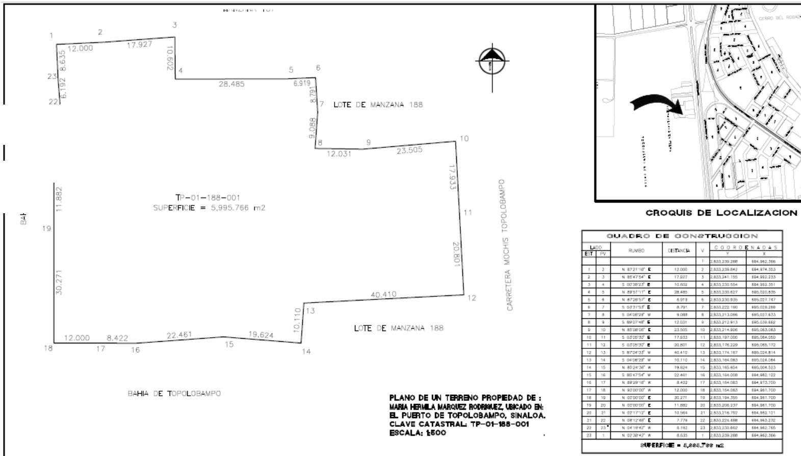
Imagen II.3.- Dimensiones del Polígono general (5,995.766 m²). Plano 1 anexo. Ver detalles en Plano 1.
