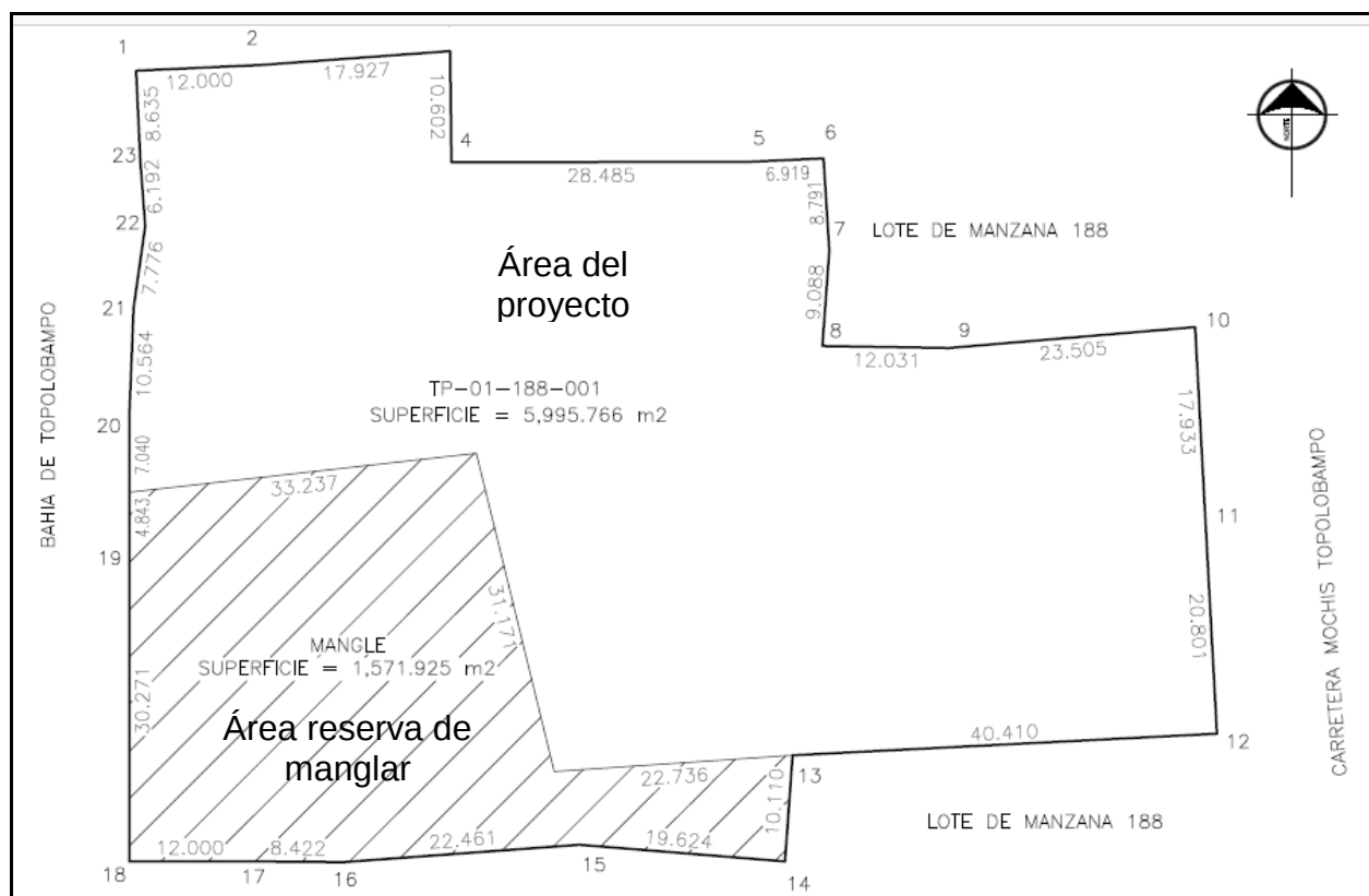
Imagen II.5- Dimensiones del área que se pretende dejar como reserva de manglar y que no será afectada por el desarrollo del proyecto. Se describen sus medidas y coordenadas en la Tabla II.5. Ver detalles en Anexo 1, Plano 3.
