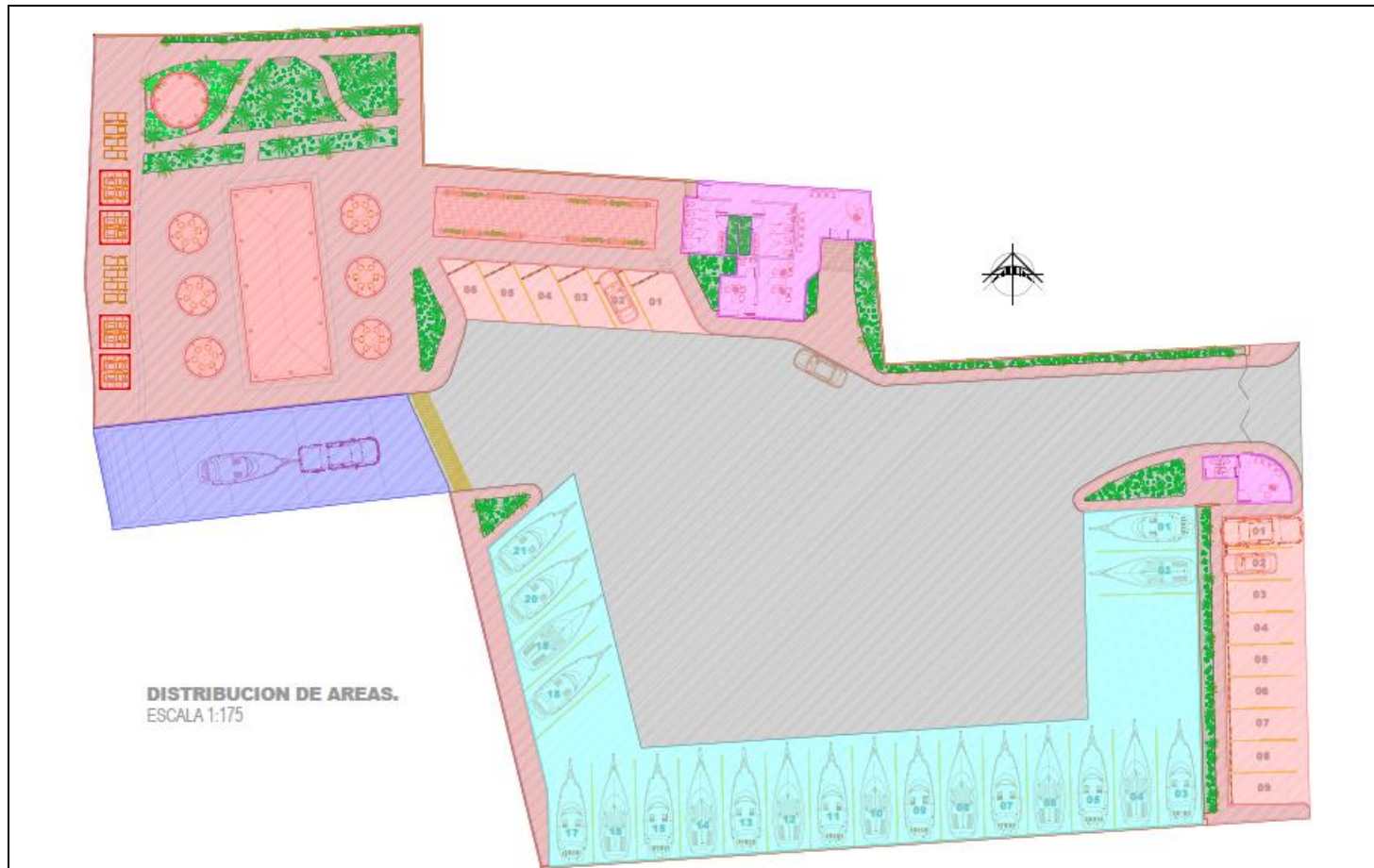
Imagen II.7.- Distribución de áreas. Ver detalles en Plano A-02.
