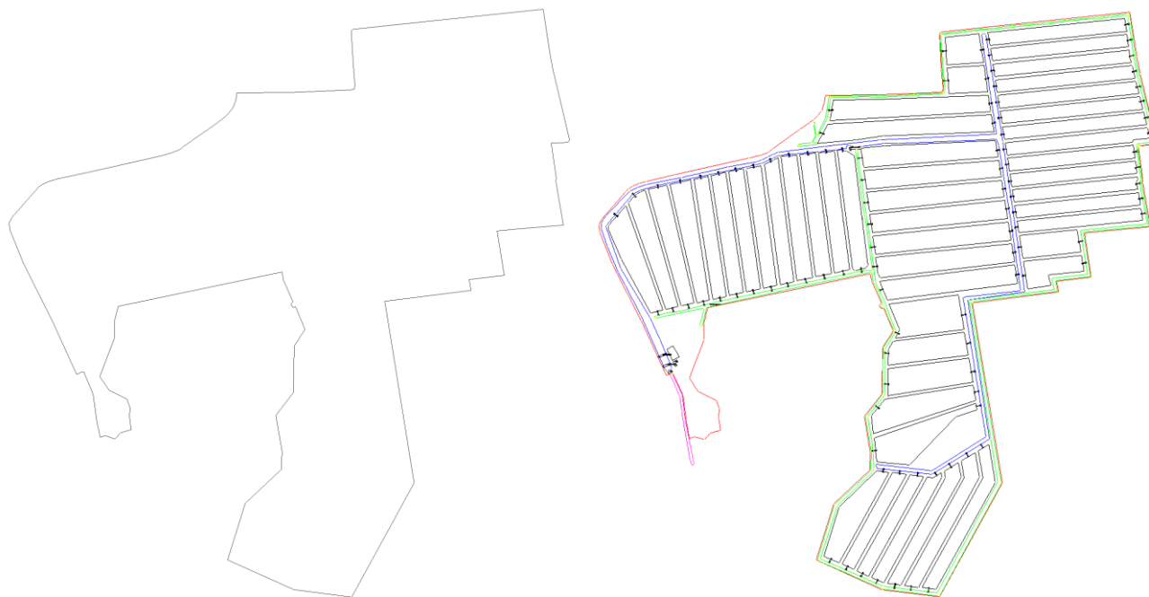
Ilustración 1.-Plano general del proyecto y polígono envolvente
