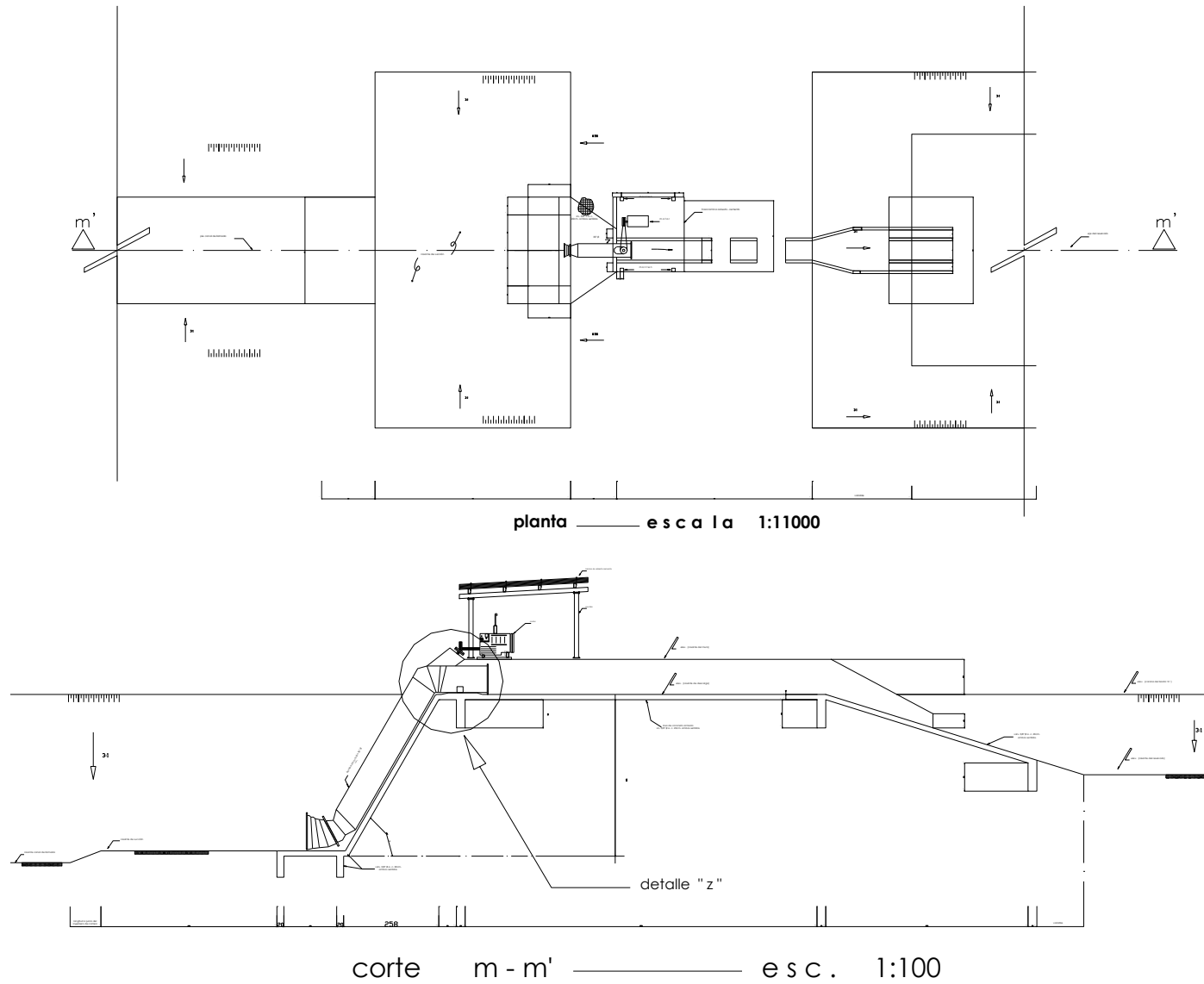
Ilustración 34.- Bombeo ingeniería
