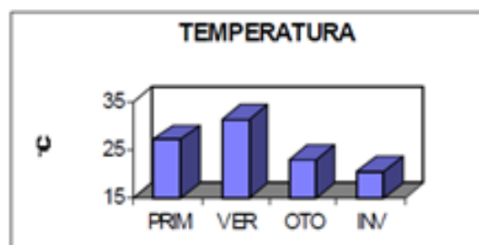
Ilustración 42.- Temperatura superficial del mar (°C) promedio en el Sistema Lagunar Bahía Santa María-Topolobampo-Ohuira registrada en los diferentes meses de muestreo.
