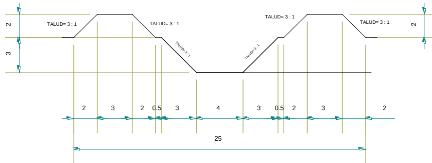
Ilustración 35.- Secciones de Bordos
