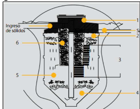
Ilustración 39.- Mecanismo Biodigestor
