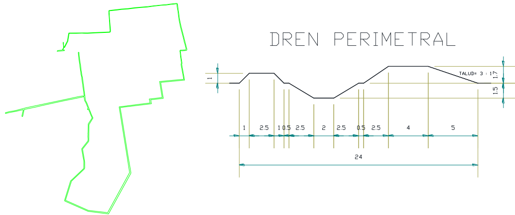
Ilustración 15.- Dren de descarga
