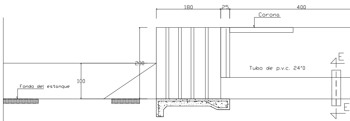
Ilustración 41.- Detalle Ingeniería Compuertas
