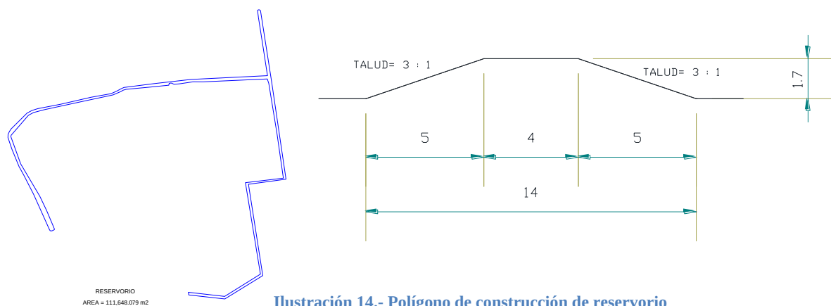
CUADRO DE CONSTRUCCIÓN DEL RESERVORIO
