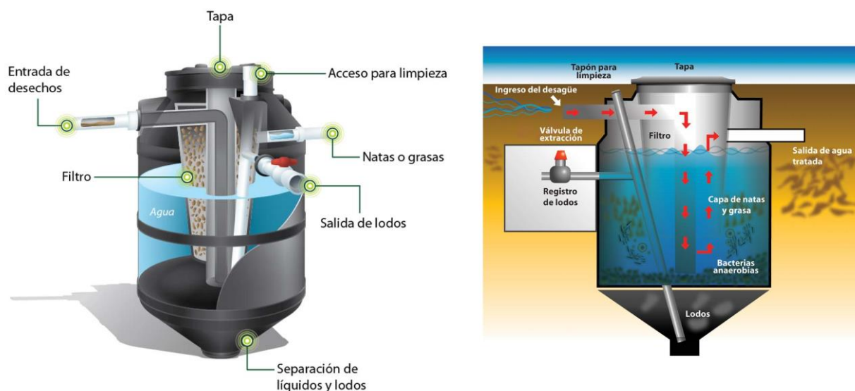
Ilustración 38.- Detalle Biodigestor
