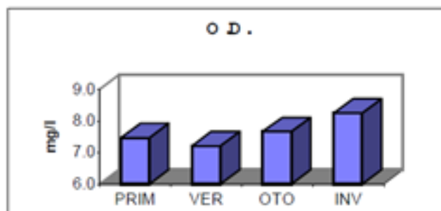
Ilustración 44.-Oxígeno Disuelto promedio en el Sistema Lagunar Sistema Lagunar Bahía Santa María-Topolobampo-Ohuira en los diferentes meses de muestreo.
