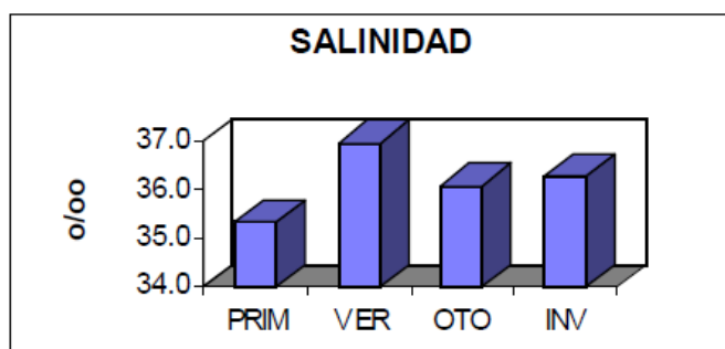
Ilustración 43.-Salinidad promedio en el Sistema Lagunar Sistema Lagunar Bahía Santa María-Topolobampo-Ohuira en los diferentes meses de muestreo.
