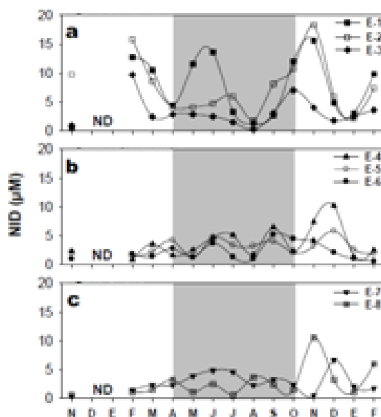
Ilustración 45.-Nitrógeno inorgánico disuelto promedio en el Sistema Lagunar Sistema Lagunar Bahía Santa María-Topolobampo-Ohuira registrado en los diferentes meses de muestreo.
