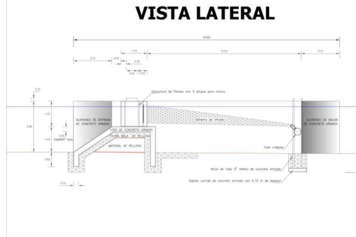
Prototipo 4 de acuerdo con la NORM-074-SAG/PESC-2014
