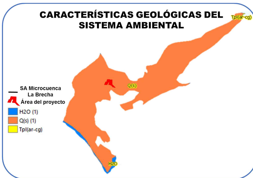
Figura IV.7.-Características Geológicas del SA
