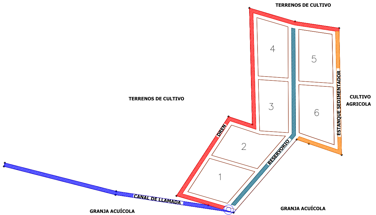
Imagen 4.- Vista de la infraestructura proyectada de la granja.
