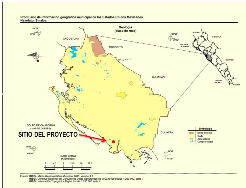
Imagen IV.8. Geología del Municipio de Navolato. INEGI.
