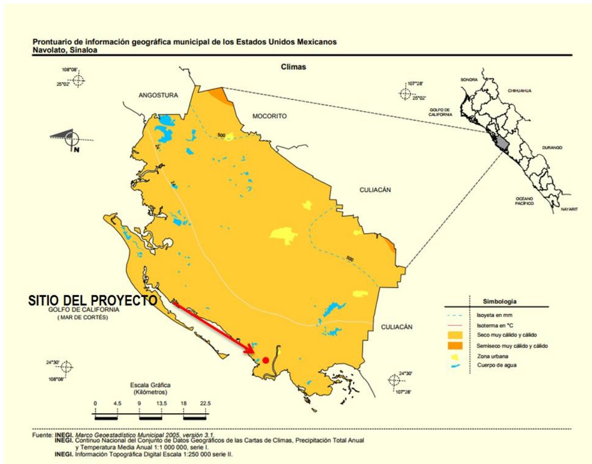
Imagen. Clima del municipio de Navolato. INEGI.
