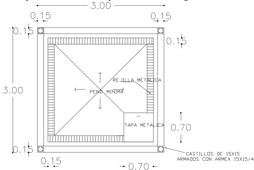
Vista en planta del Almacén Temporal de Residuos Peligrosos
