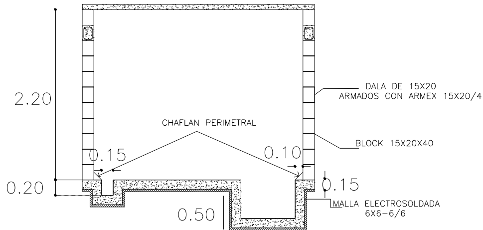
Imagen No. 11.- Planta de Almacén de Residuos Peligrosos.
