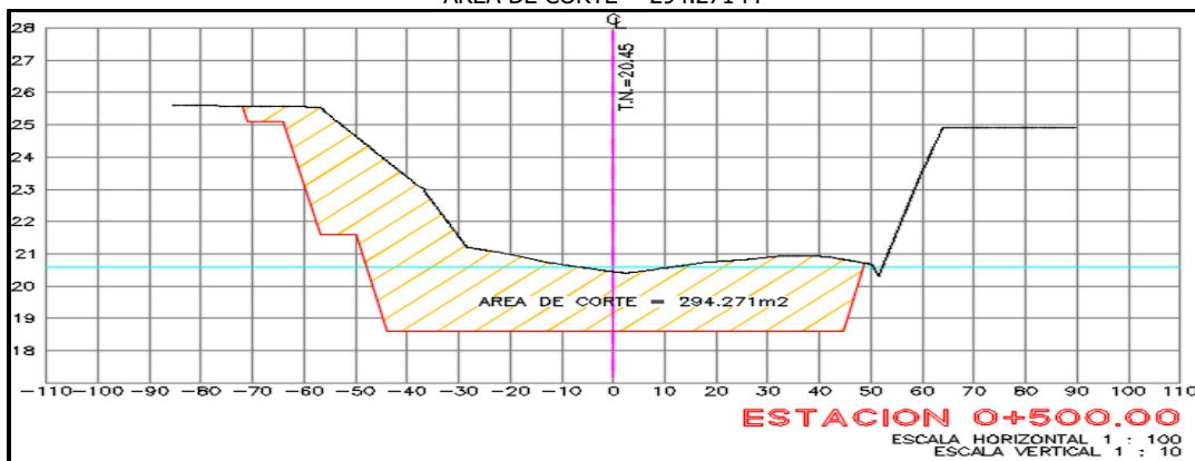
FIGURA 3.- ESTACION 0+500.000 (PARTE CENTRAL DEL PROYECTO): AREA DE TERRAPLEN = 0.000 M 2 AREA DE CORTE = 294.271 M 2
