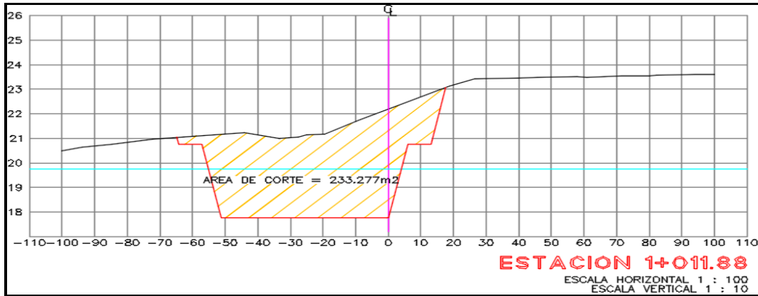
FIGURA 4.- ESTACION 1+011.88 (PARTE FINAL DEL PROYECTO): AREA DE TERRAPLEN = 0.000 M 2 AREA DE CORTE = 233.277 M 2
